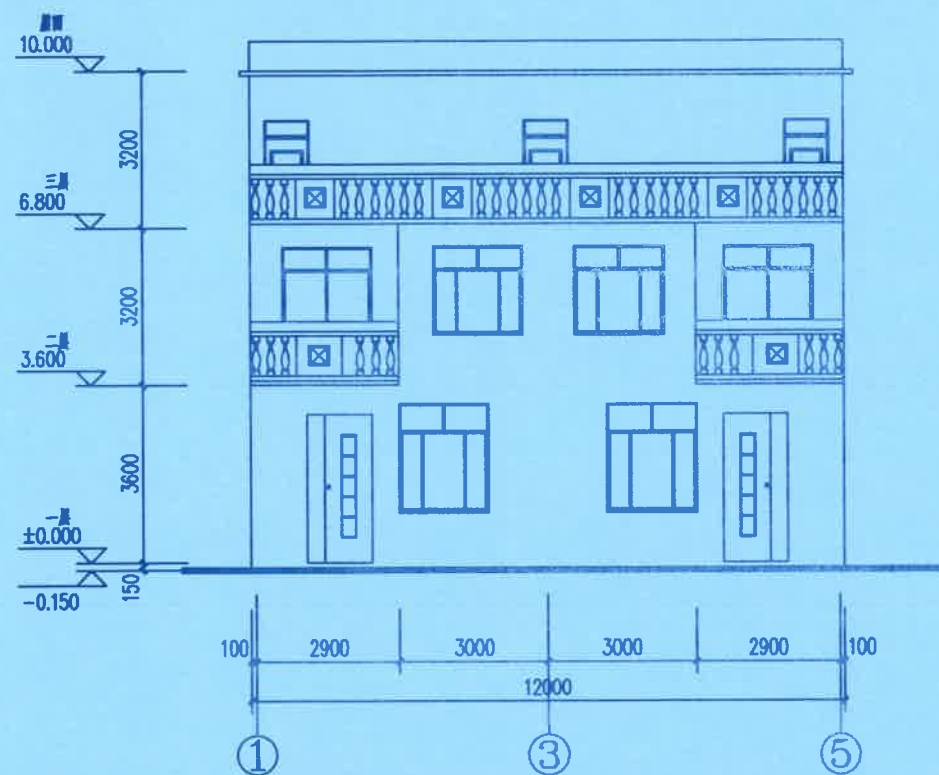
①-⑤ 轴立面图 1:100
