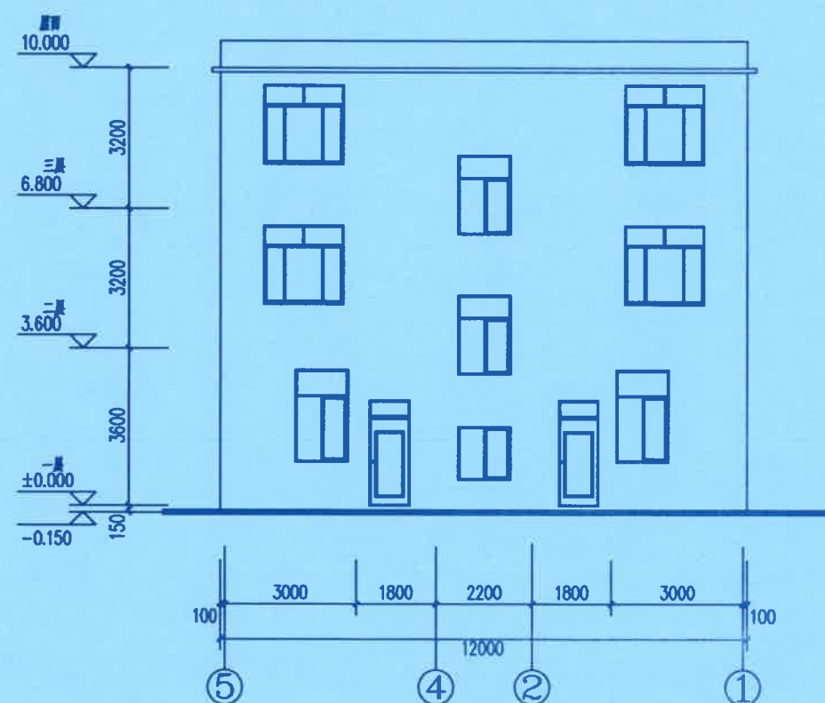
⑤ - ① 轴立面图 1:100
