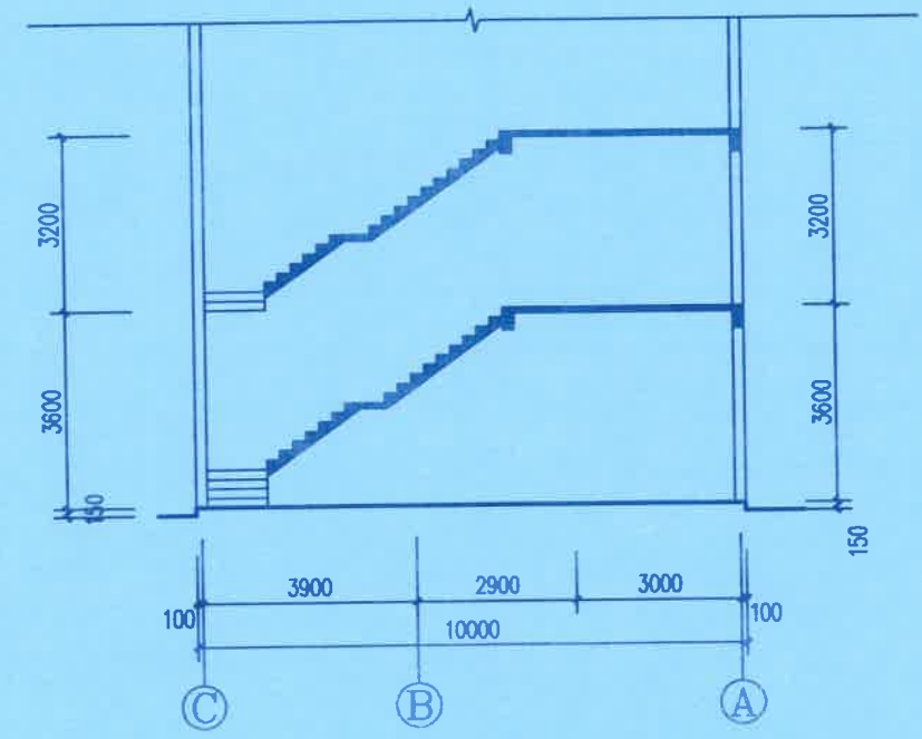
楼梯间剖面图 1:100
