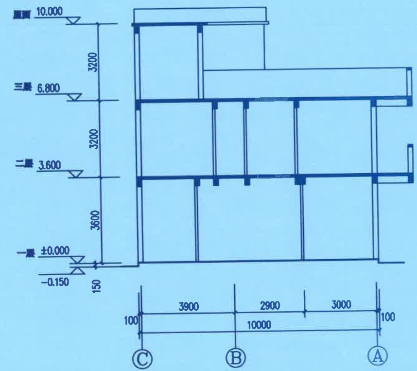
1-1 剖面图 1:100
