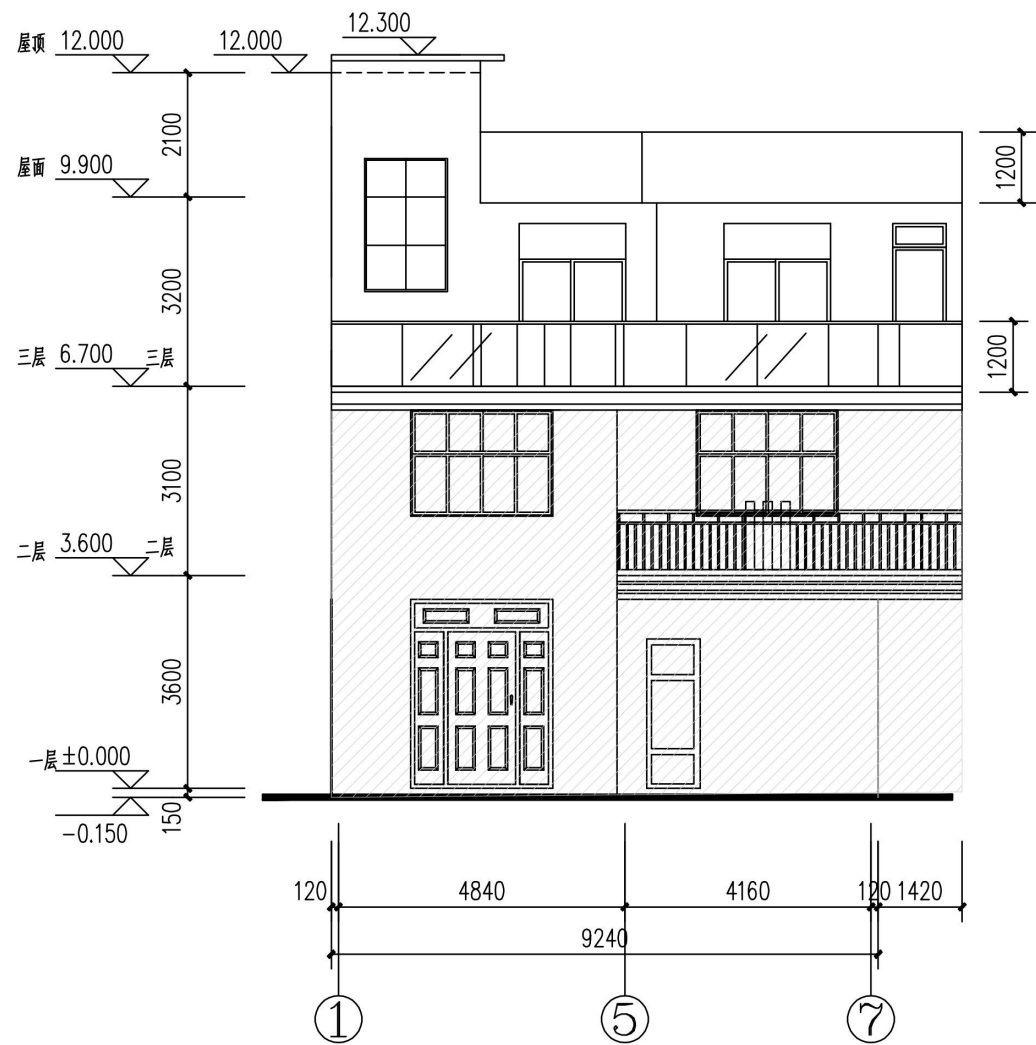
①~⑦轴立面图 1:100
