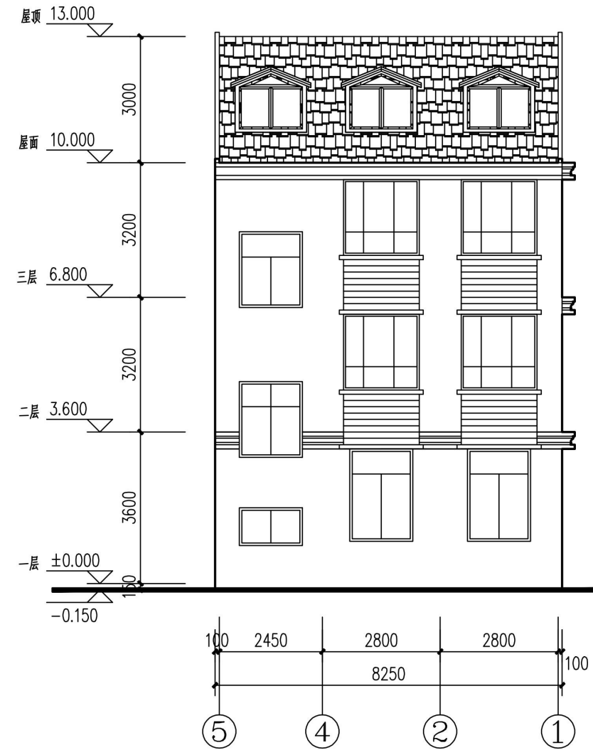
北立面图 1:100
