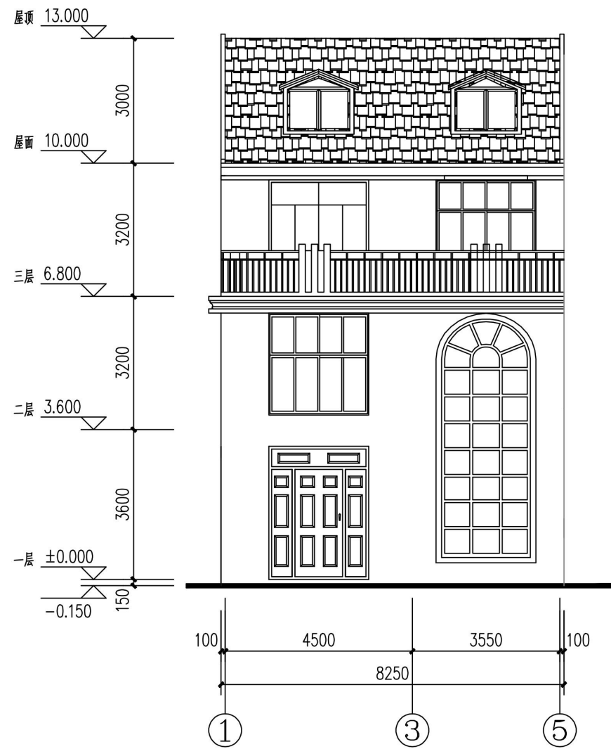
南立面图 1:100
