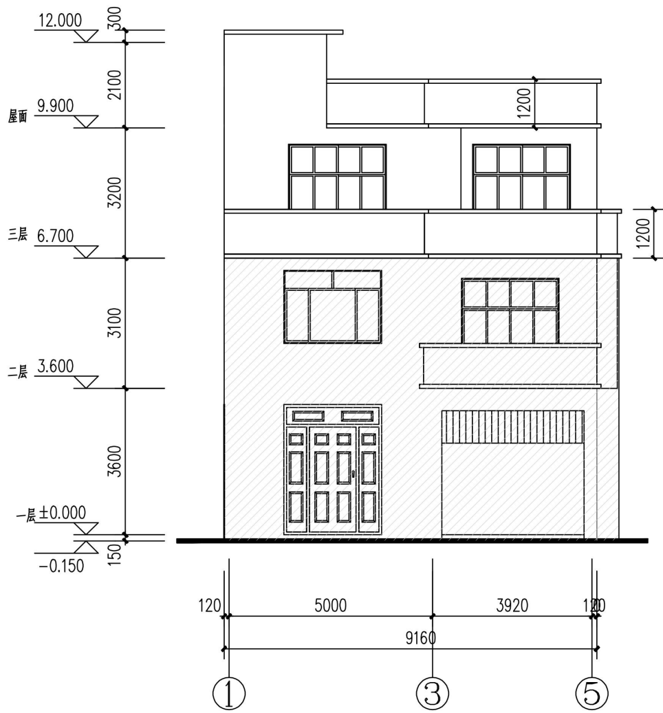
①~⑤轴立面图 1:100 (拟建)
