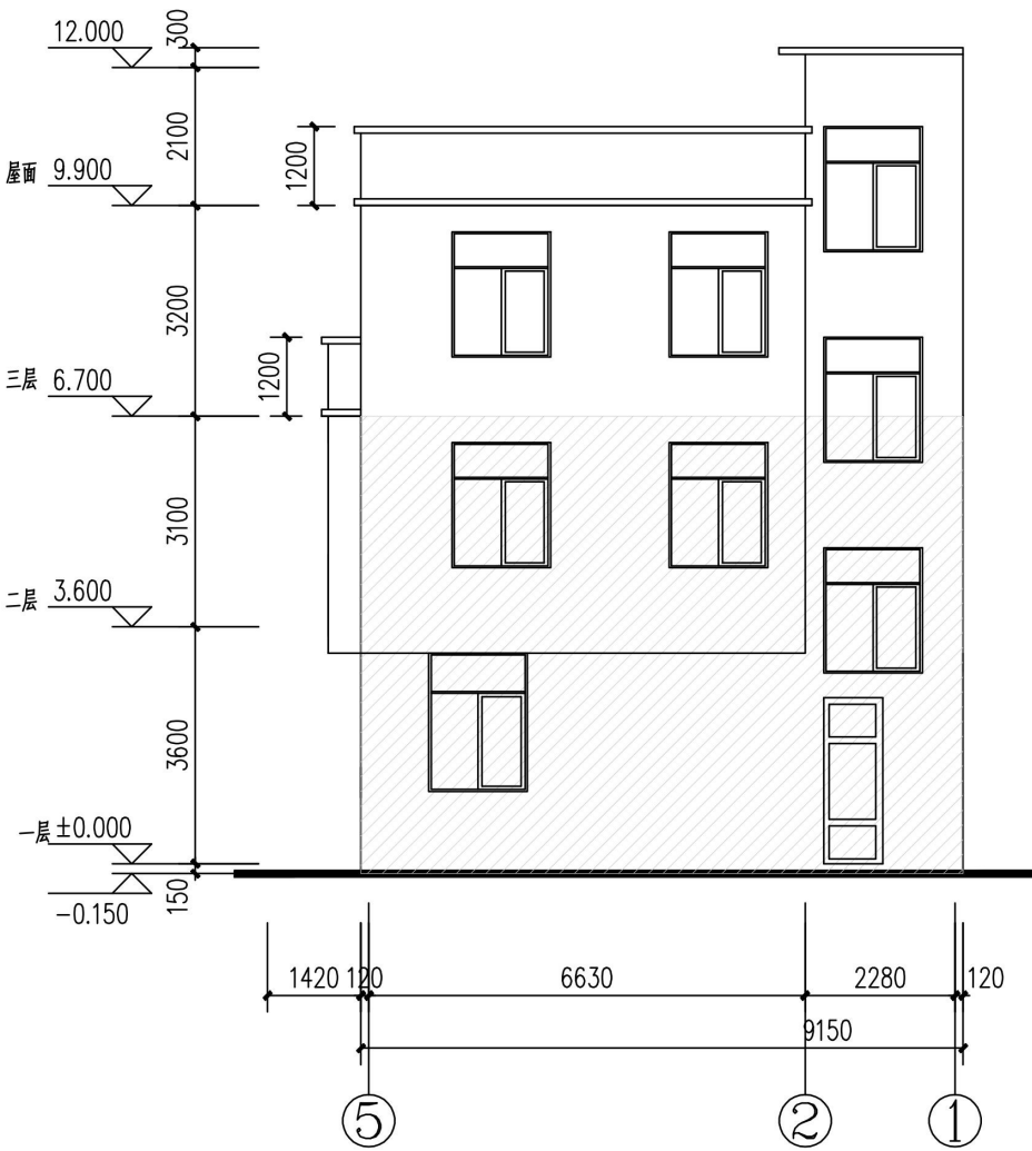
⑤~①轴立面图 1:100 (拟建)
