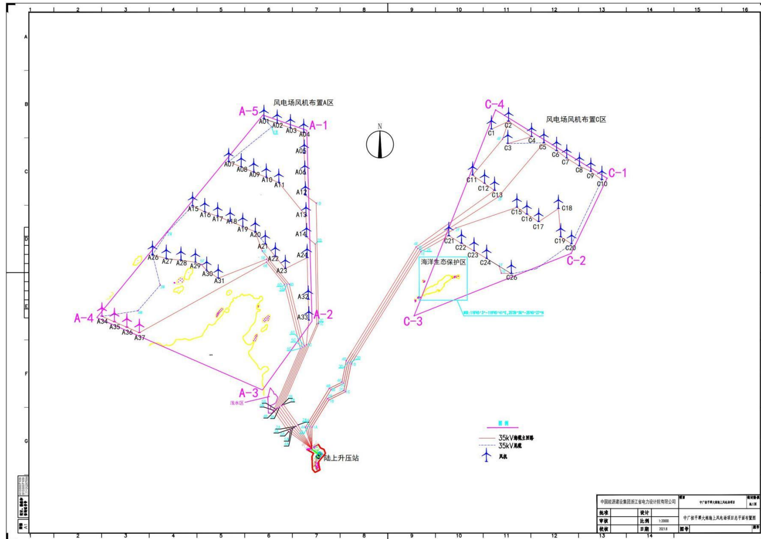
图 2.2-1 本项目用海情况第二次变更后平面布置图
