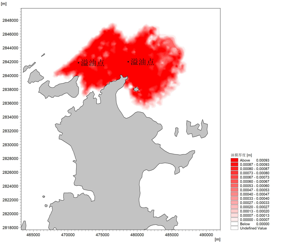
图 4.5-2 高潮时 SSW 风作用下 72h 溢油扫海包络图
