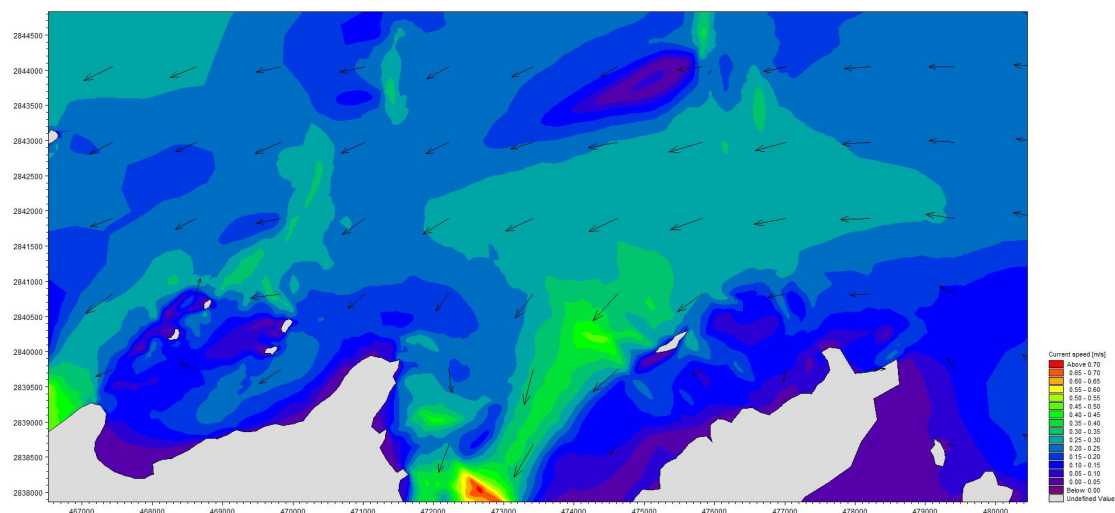
图 4.1-10 大潮期工程附近海域高潮时刻潮流场（工程前）
