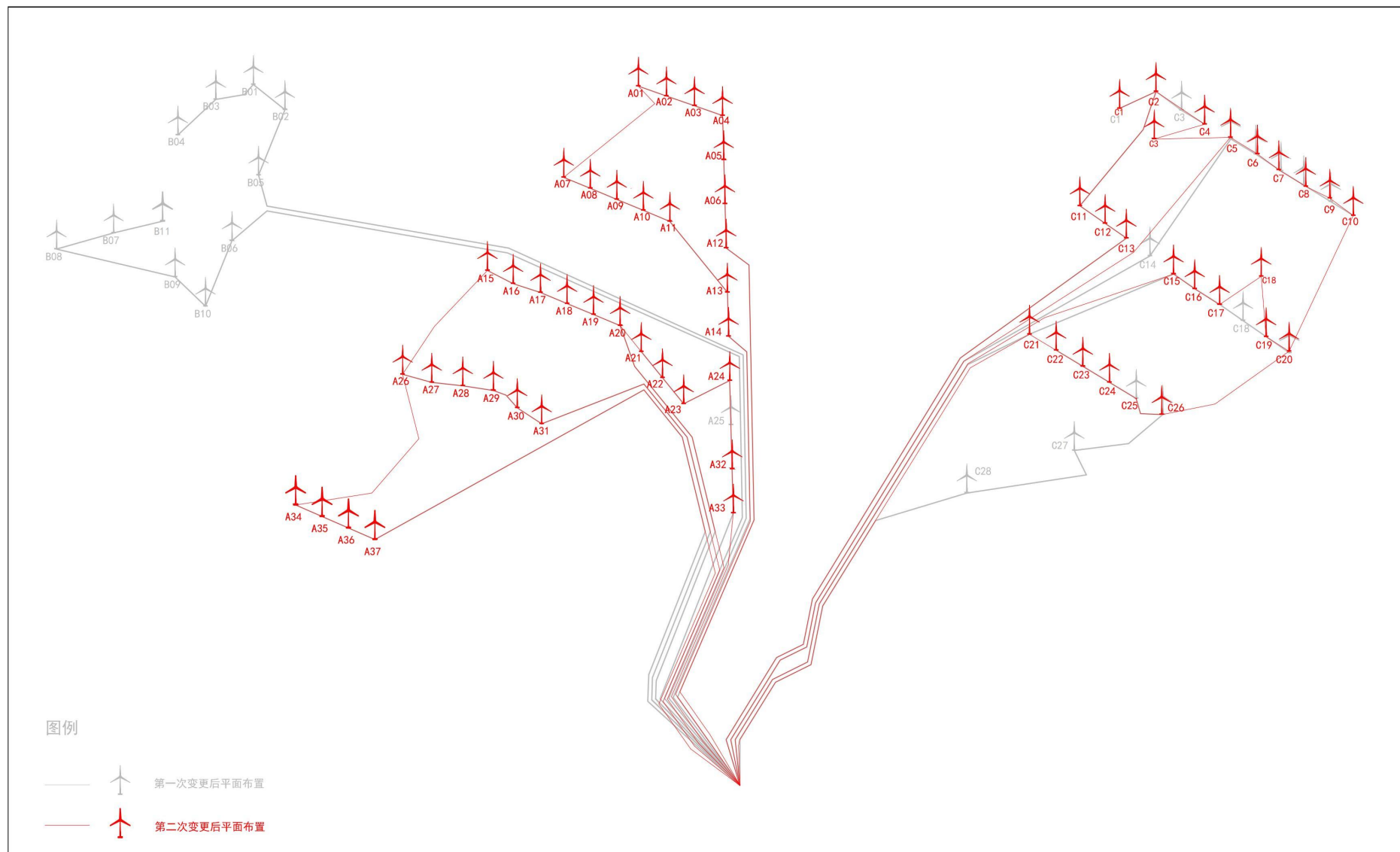
图 1.1-2 本项目用海情况第二次变更前后总平面布置对比图
