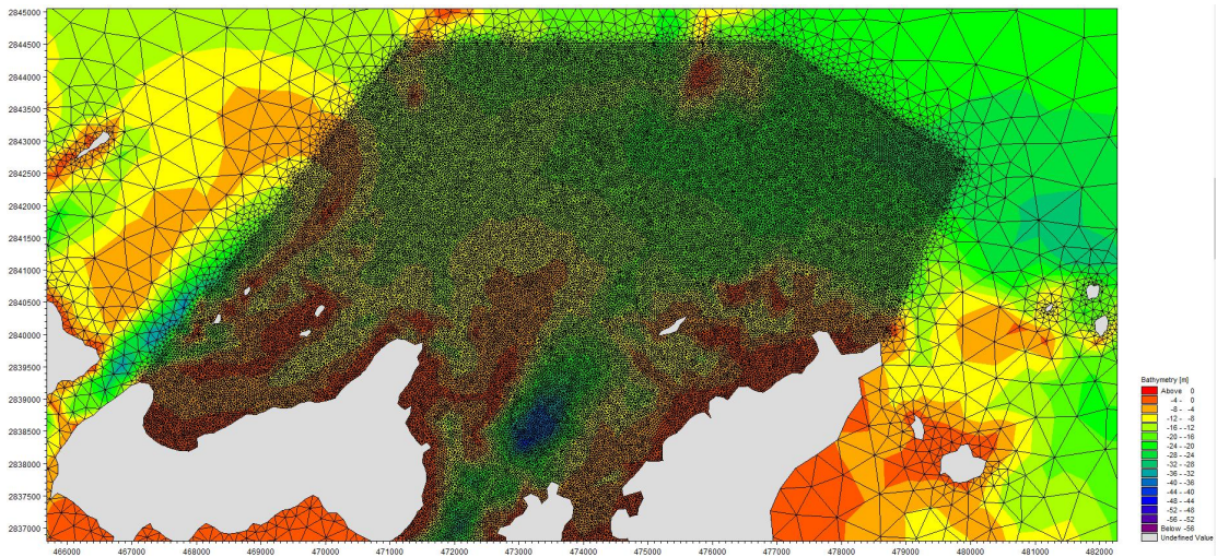
图 4.1-2 风电场附近海域网格及水深图
