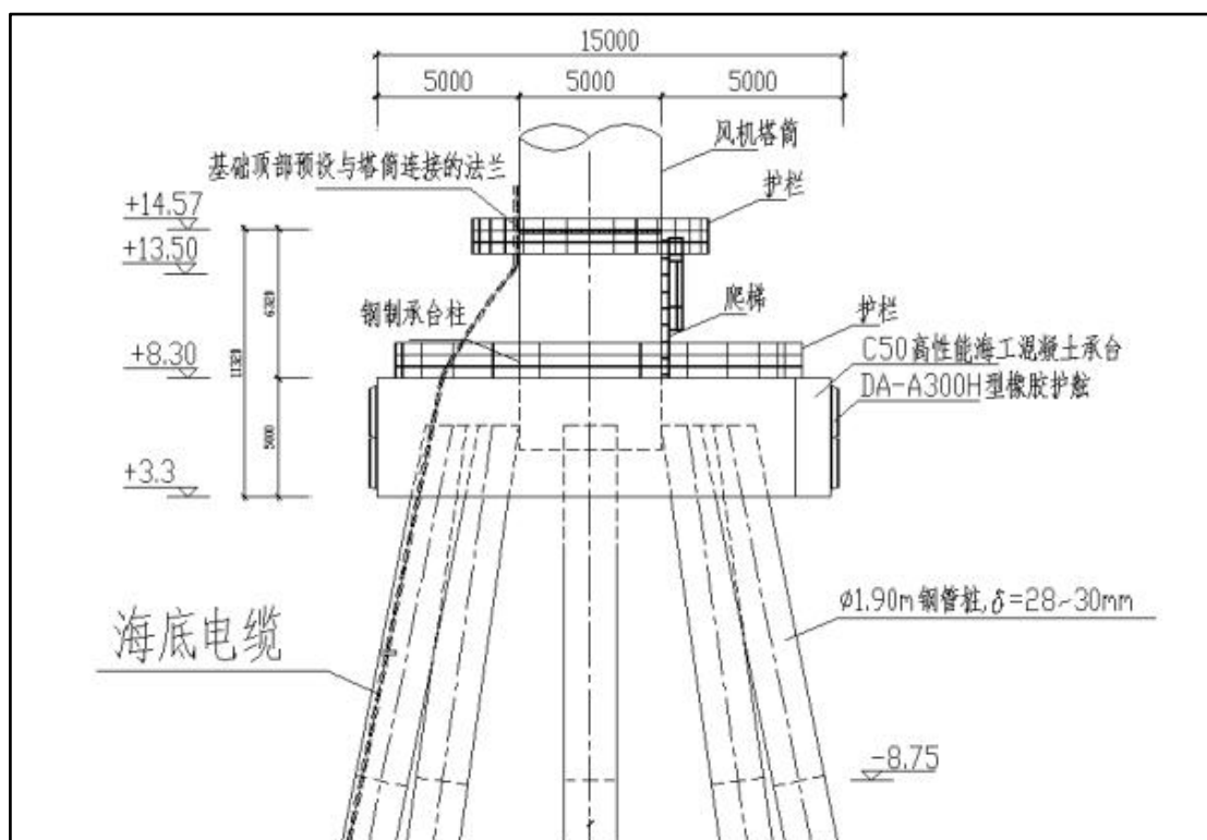
图 2.2-4 8 斜高桩承台基础结构图
