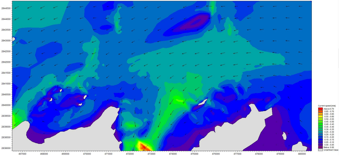
图 4.1-14 大潮期工程附近海域高潮时刻潮流场（工程后）
