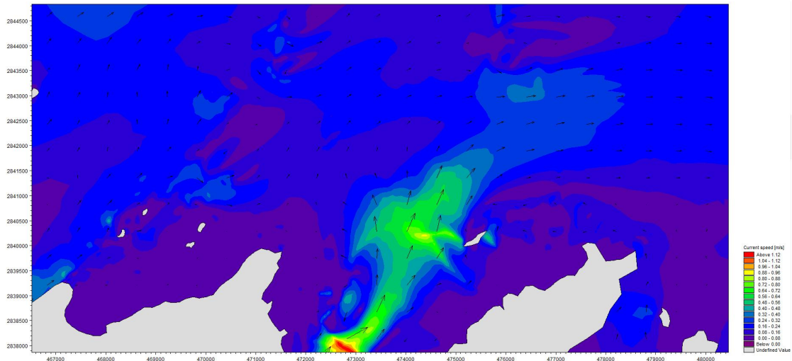
图 4.1-16 大潮期工程附近海域低潮时刻潮流场（工程后）
