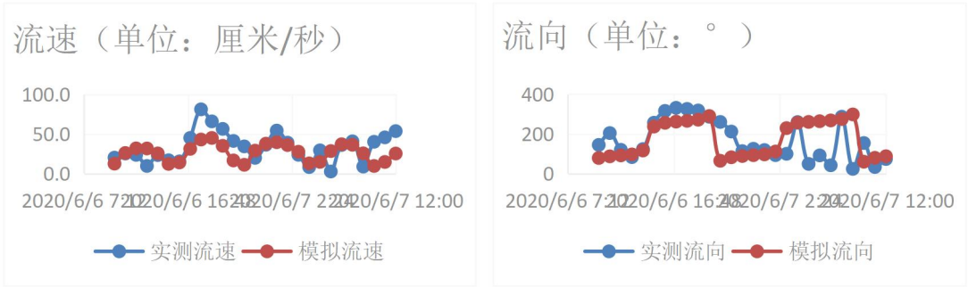
图 4.1-4f L6 站流速流向验证图
