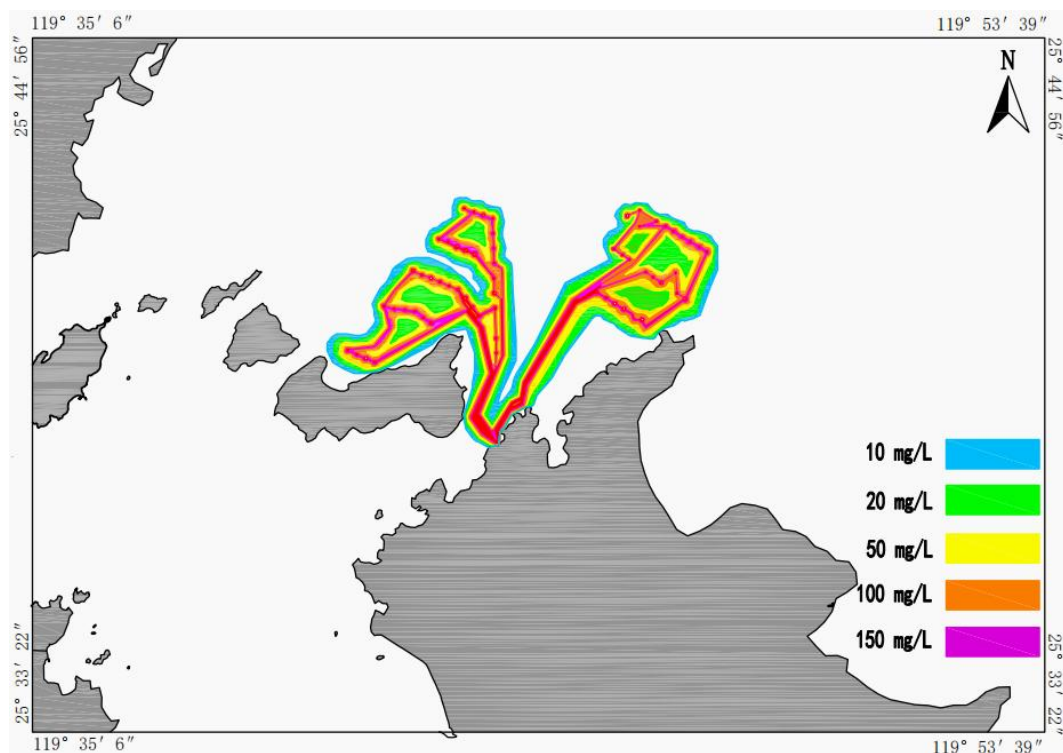
图 4.1-24 悬浮泥沙增量浓度最大影响范围包络线图
