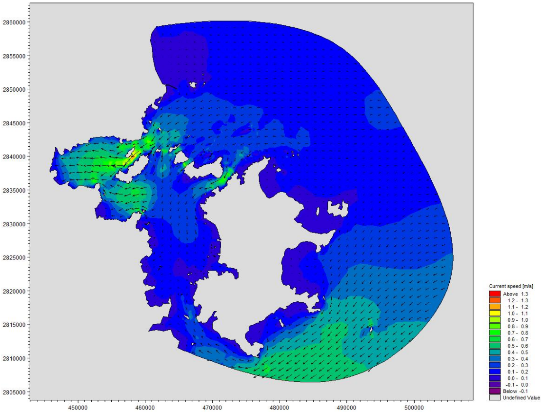
图 4.1-7 大潮期计算海域高潮时刻潮流场（工程前）
