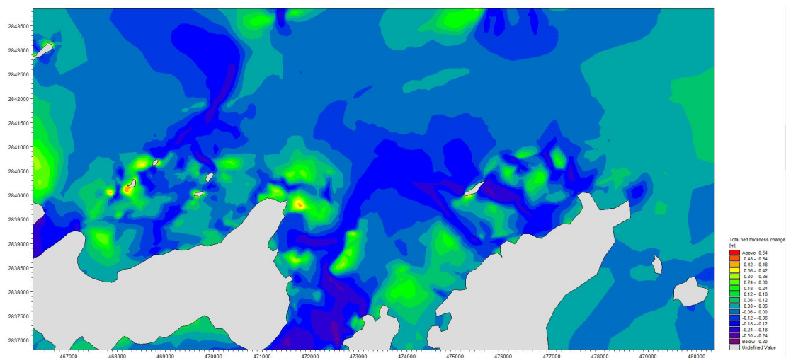
图 4.1.20 工程建设前工程周边海域年冲淤厚度图（单位：m/a）
