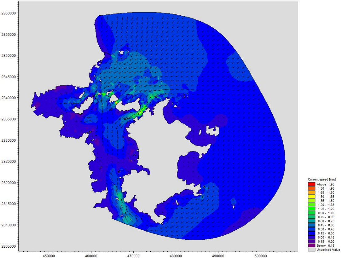
图 4.1-5 大潮期计算海域低潮时刻潮流场（工程前）
