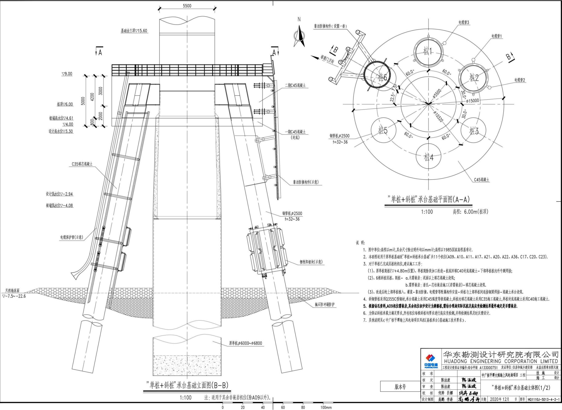
图 2.2-5 1 单桩+6 斜桩复合承台基础结构图
