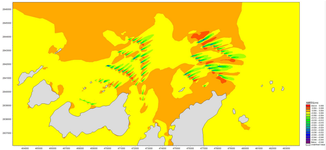
图 4.1-18 工程前后大潮落急流速变化（单位：m/s）
