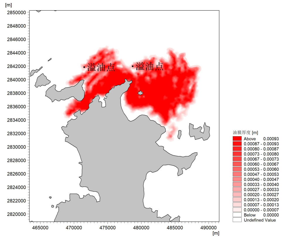
图 4.5-3 低潮时 NNE 风作用下 72h 溢油扫海包络图
