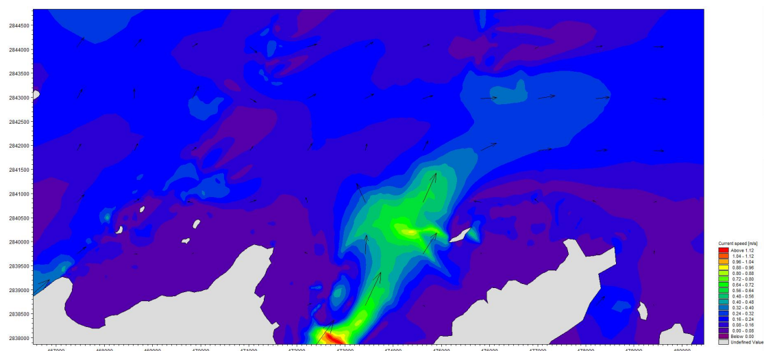
图 4.1-11 大潮期工程附近海域落急时刻潮流场（工程前）
