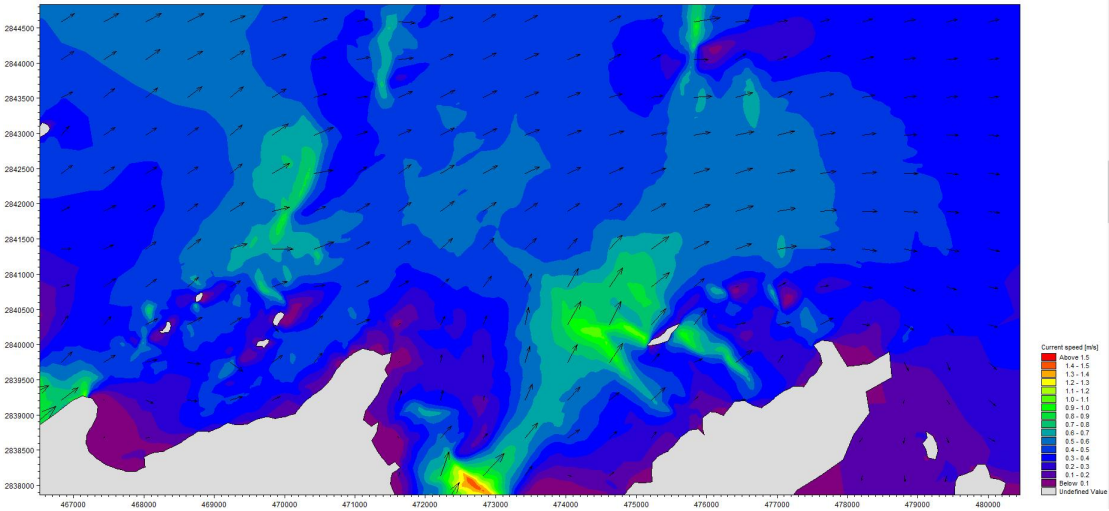
图 4.1-15 大潮期工程附近海域落急时刻潮流场（工程后）
