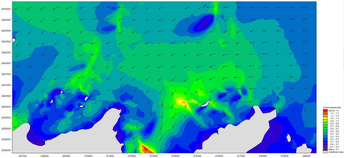
图 4.1-13 大潮期工程附近海域涨急时刻潮流场（工程后）
