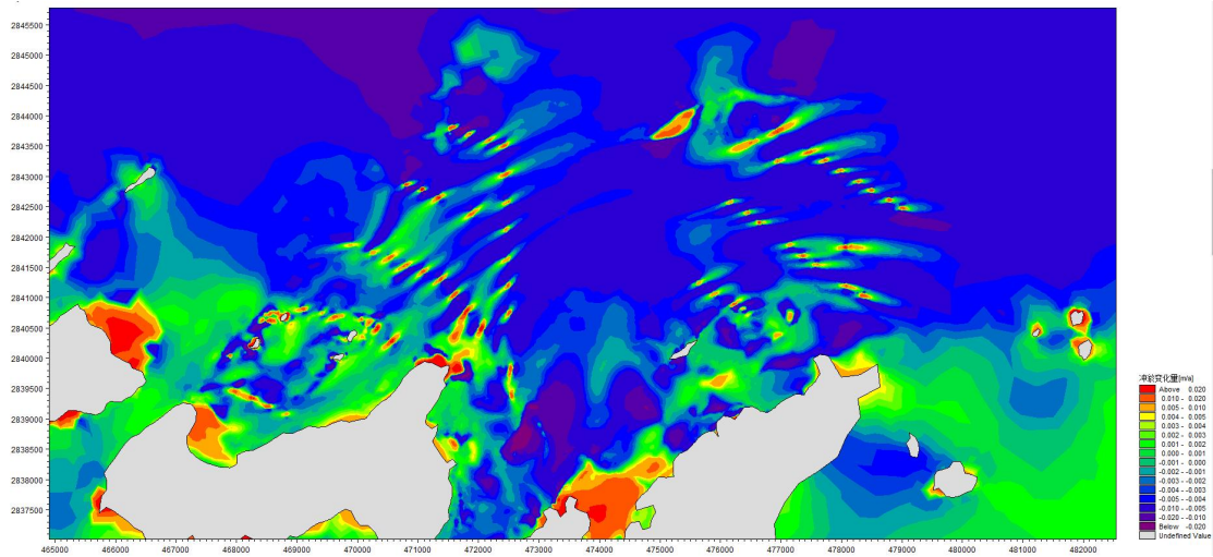
图 4.1-22 风电场附近年冲淤变化图（单位：m/a）
