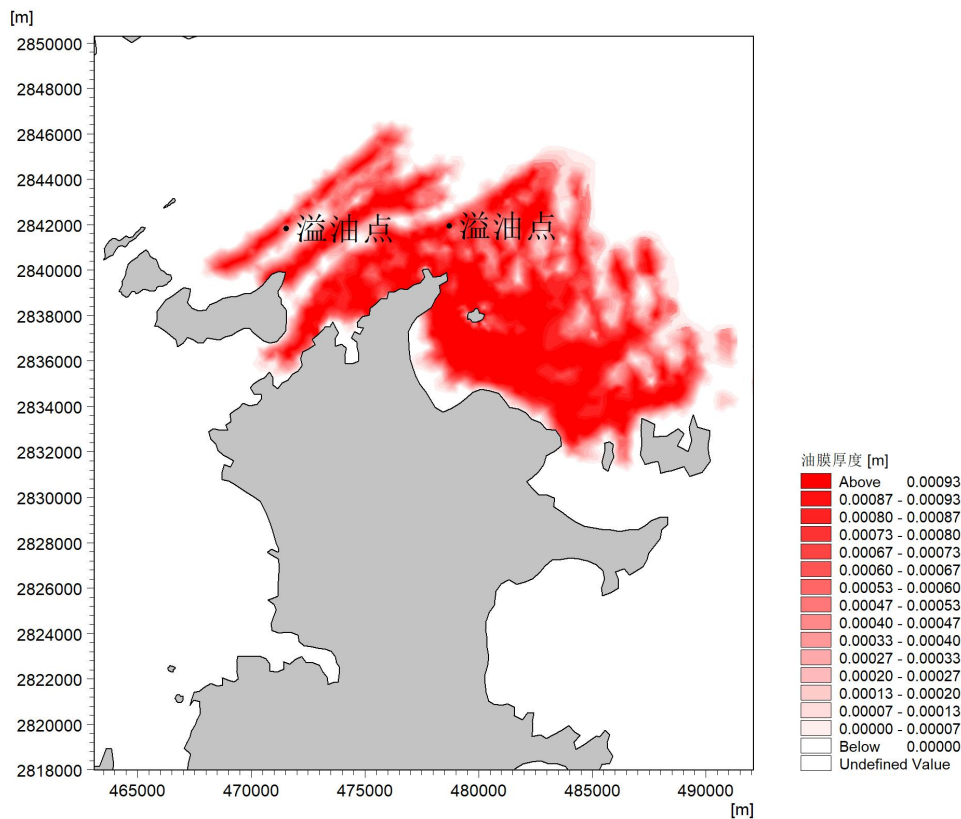
图 4.5-6 高潮时 NW 风作用下 72h 溢油扫海包络图
