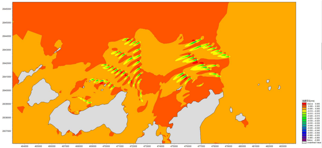
图 4.1-17 工程前后大潮涨急流速变化（单位：m/s）
