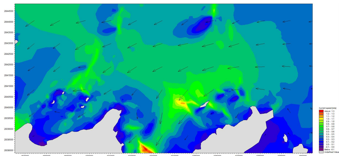
图 4.1-9 大潮期工程附近海域涨急时刻潮流场（工程前）
