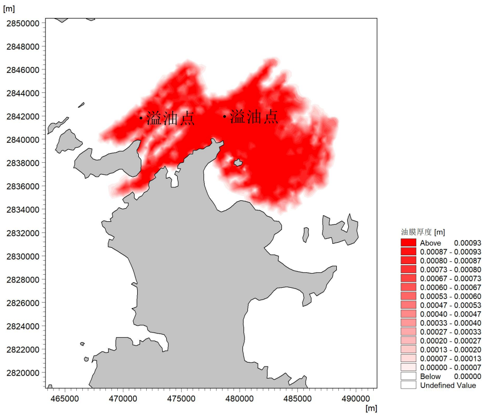
图 4.5-4 高潮时 NNE 风作用下 72h 溢油扫海包络图
