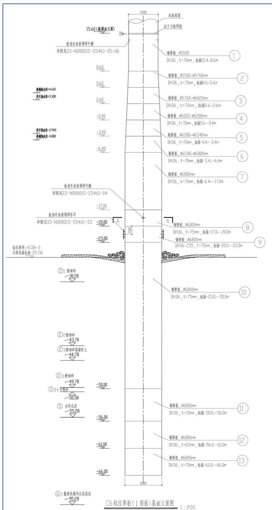
图 2.2-3 单桩基础结构图
