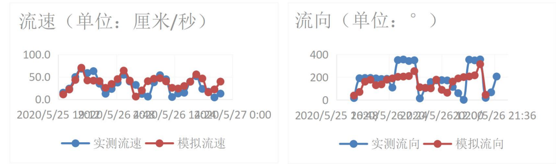
图 4.1-4a L1 站流速流向验证图
