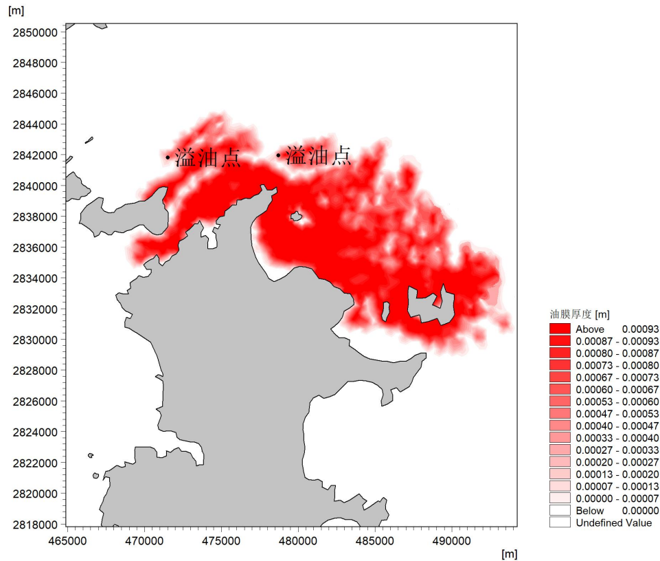
图 4.5-5 低潮时 NW 风作用下 72h 溢油扫海包络图
