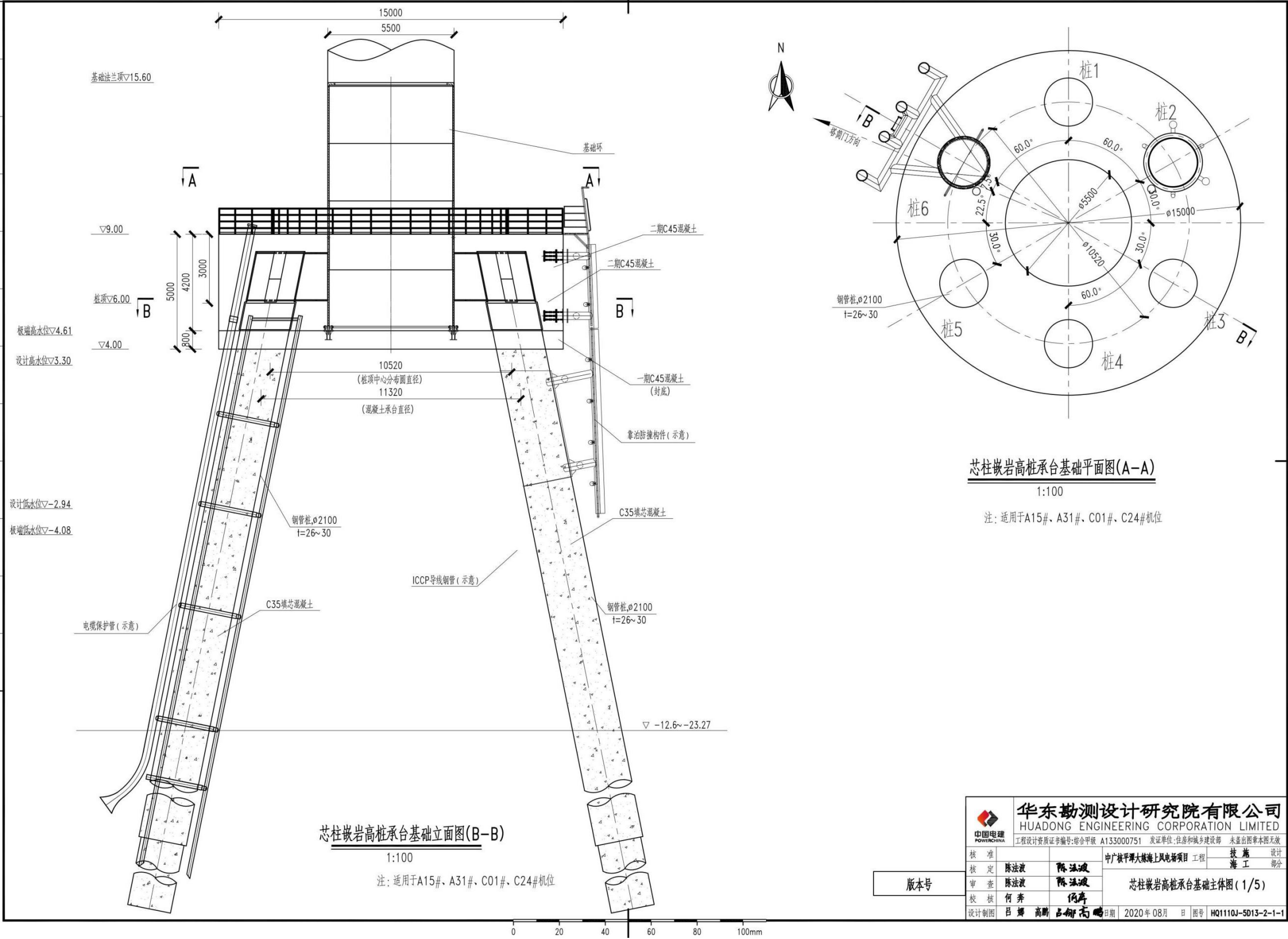
图 2.2-6 6 斜高桩承台基础结构图
