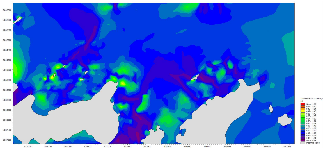
图 4.1.21 工程建设后工程周边海域年冲淤厚度图（单位：m/a）
