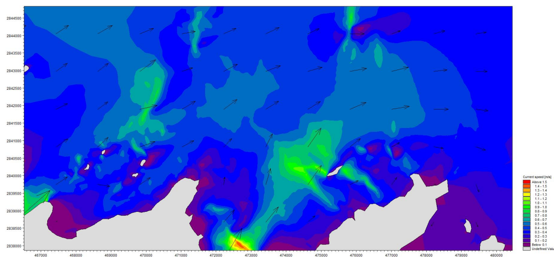
图 4.1-12 大潮期工程附近海域低潮时刻潮流场（工程前）
