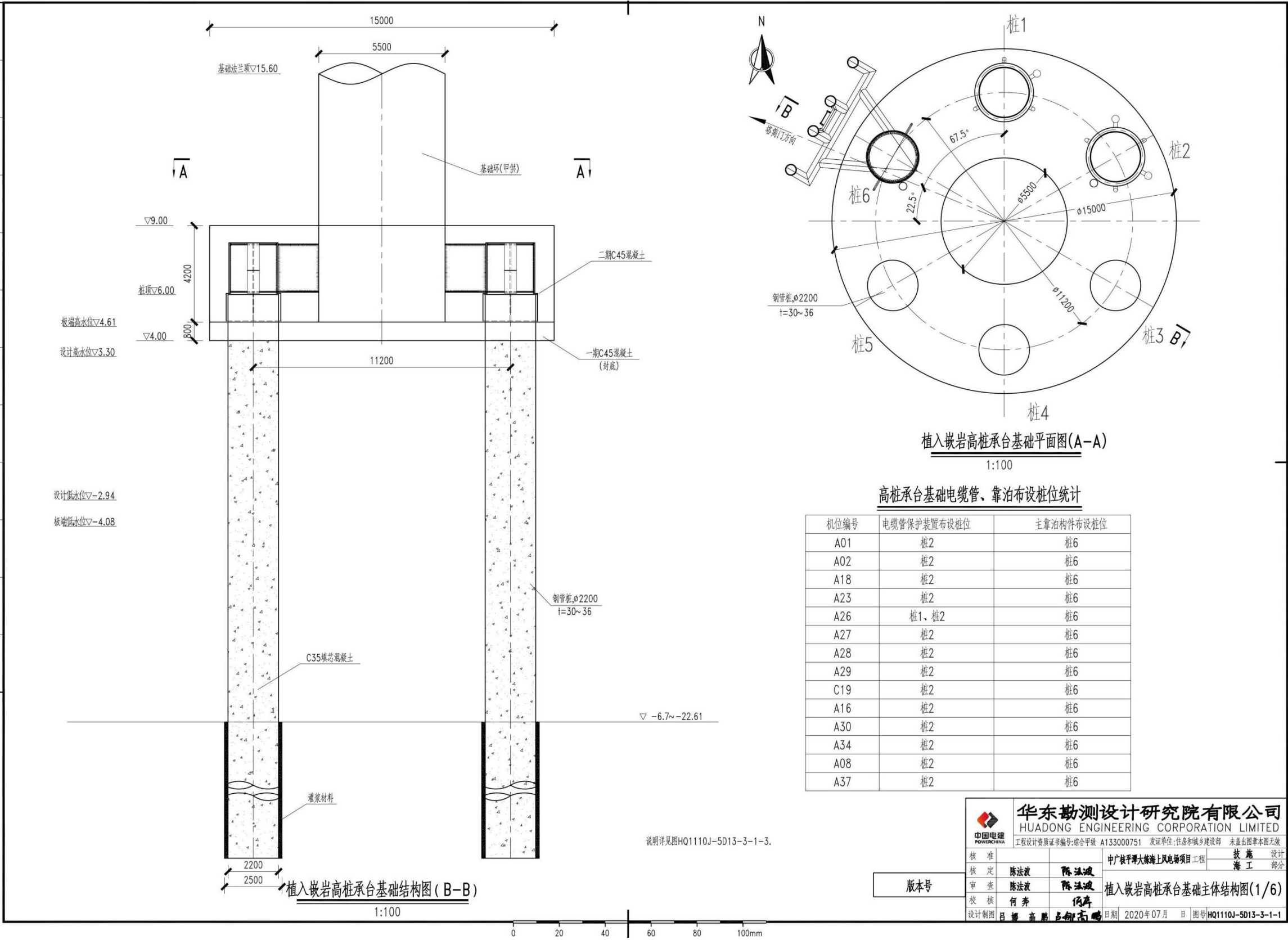
图 2.2-7 6直高桩承台基础结构图
