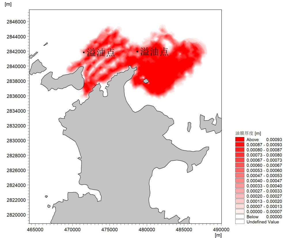
图 4.5-1 低潮时 SSW 风作用下 72h 溢油扫海包络图
