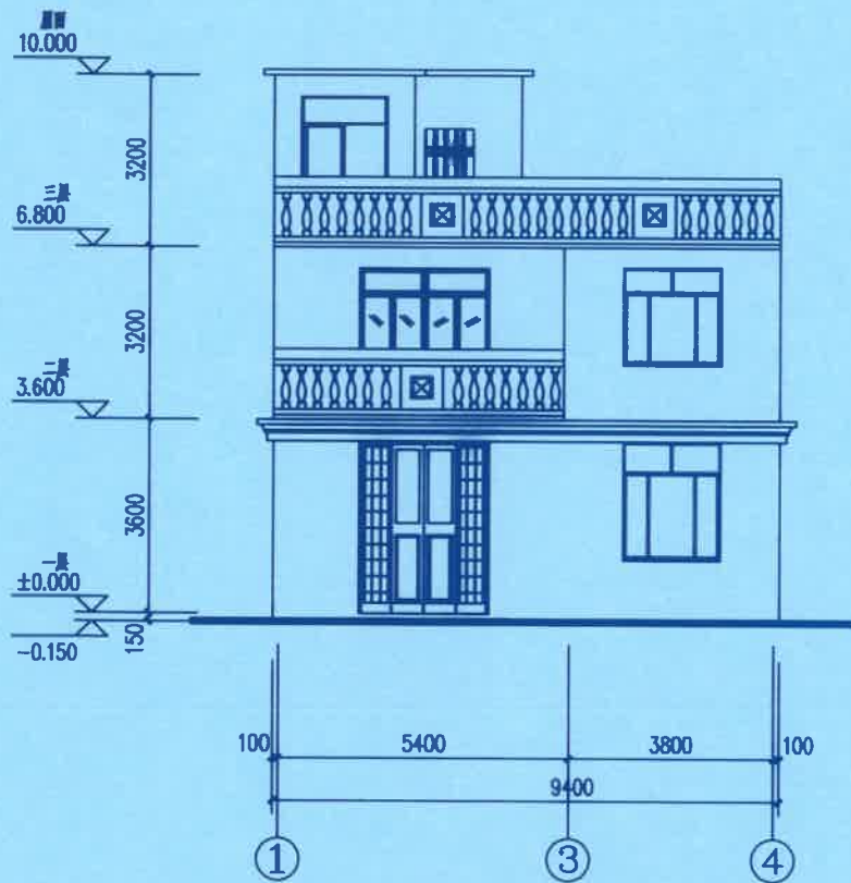
① - ④ 轴立面图 1:100
