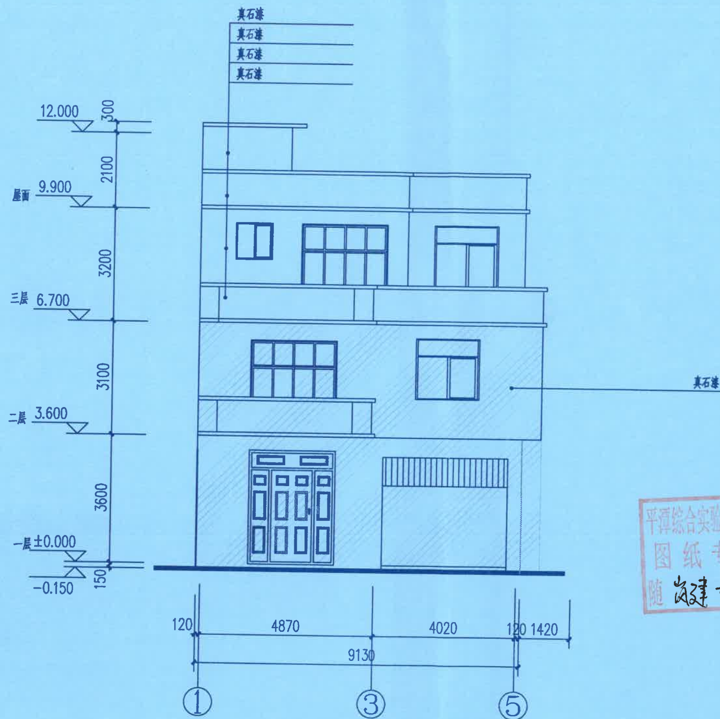
①~⑤轴立面图 1:100 (拟建)
