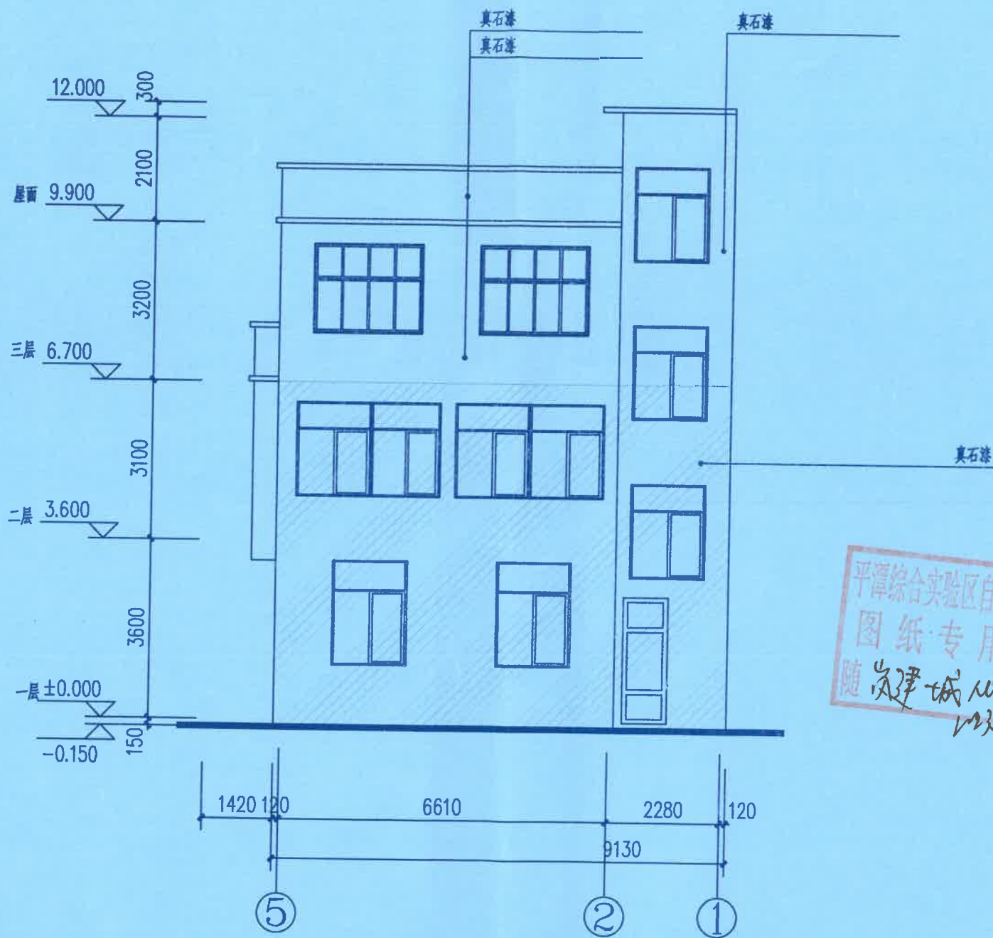
⑤~①轴立面图 1:100 (拟建)
