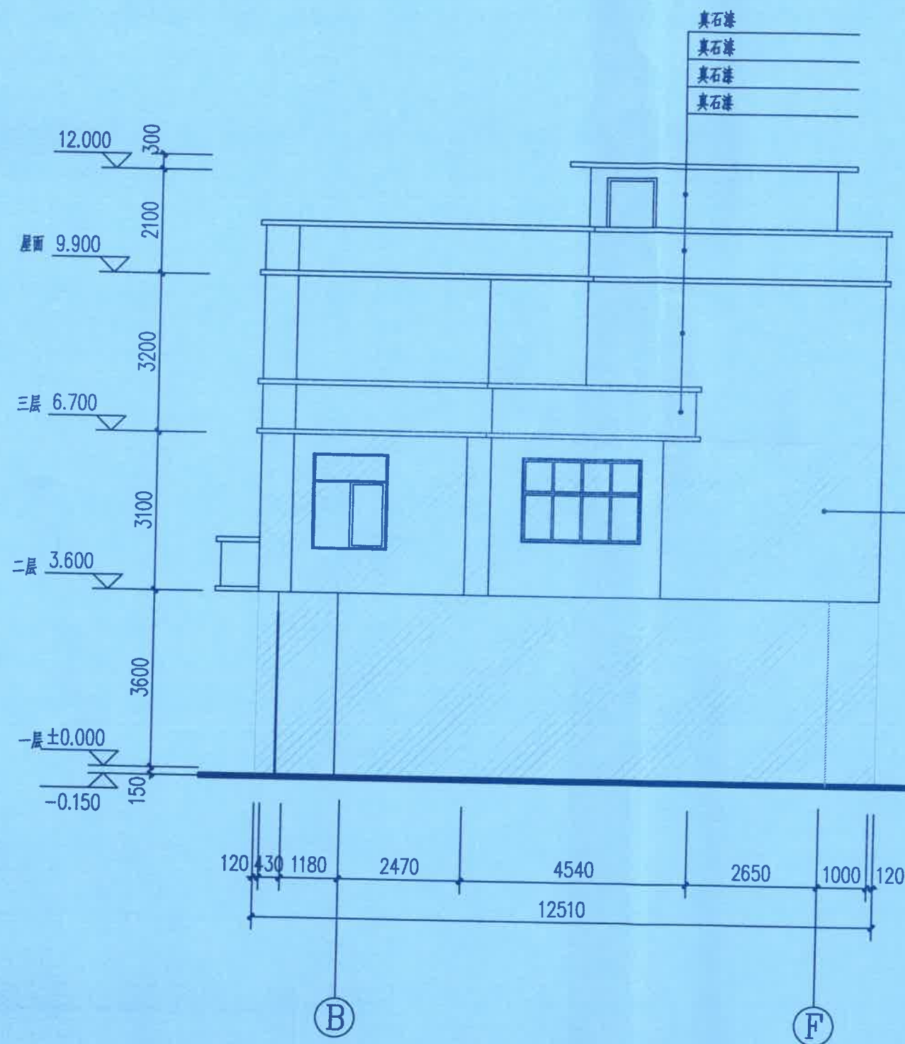
B~F轴立面图 1:100 (拟建)
