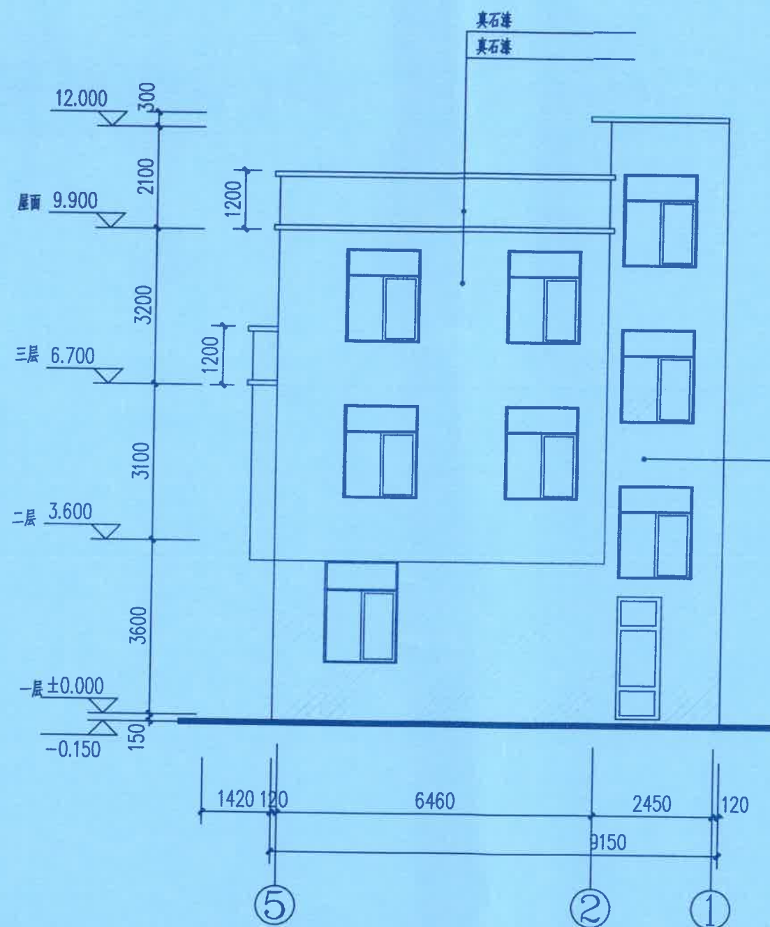
⑤~①轴立面图 1:100 (拟建)
