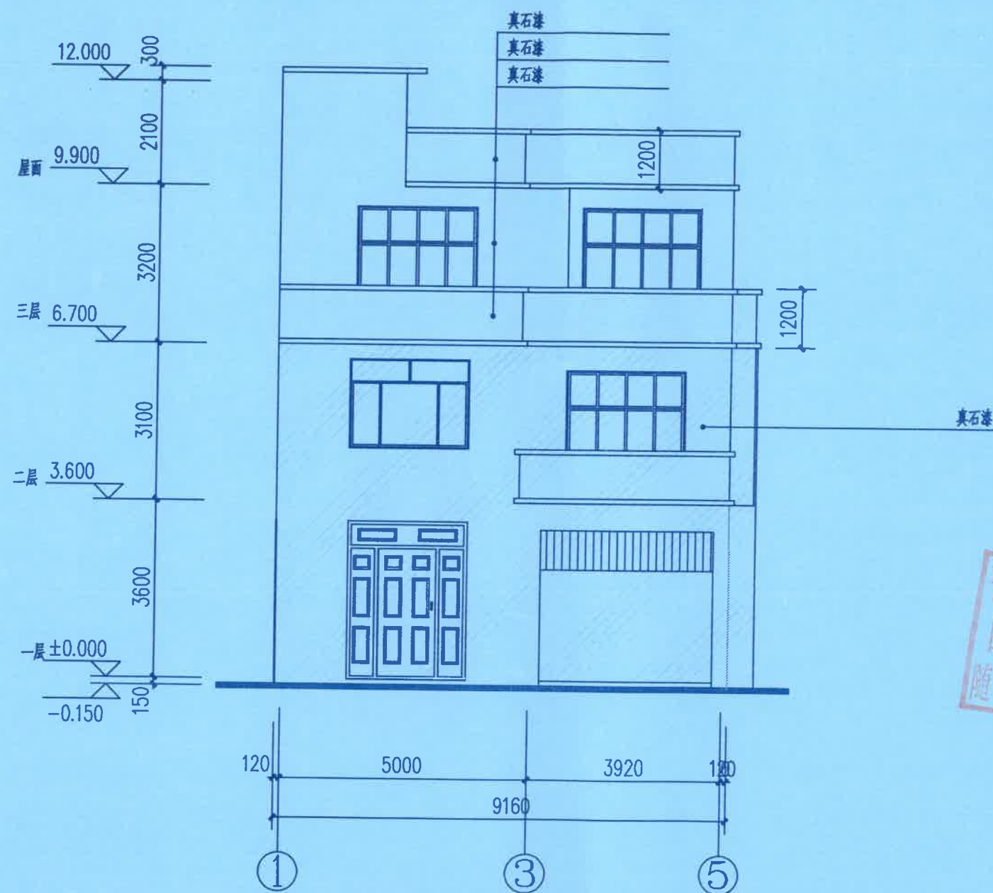
①~⑤轴立面图 1:100 (拟建)
