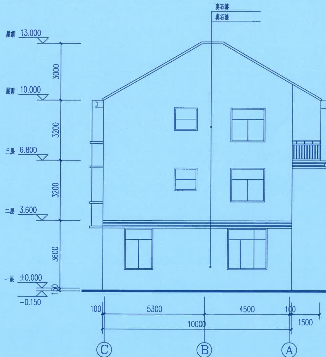
西立面图 1:100
