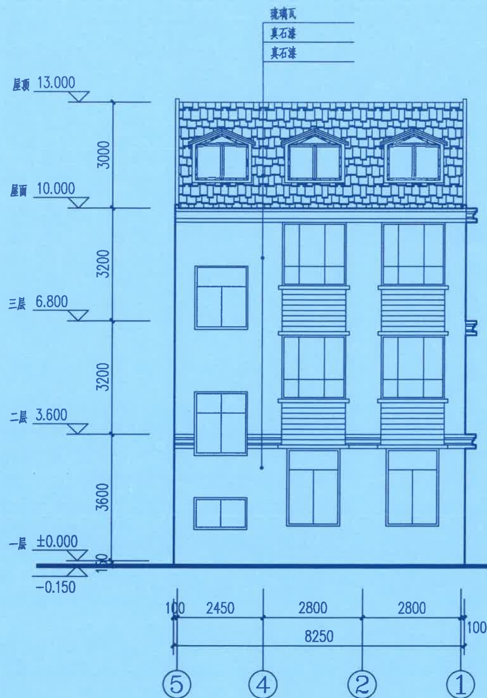
北立面图 1:100
