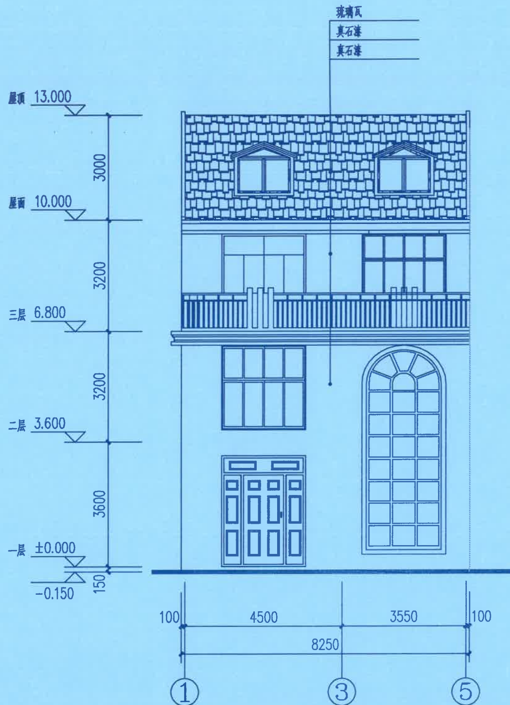
南立面图 1:100
