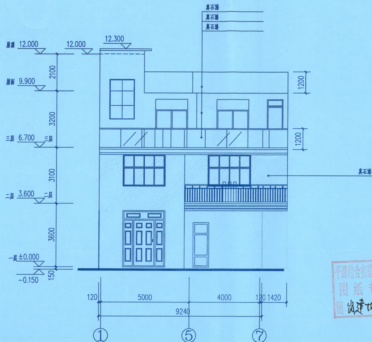
①~⑦轴立面图 1:100 (拟建)
