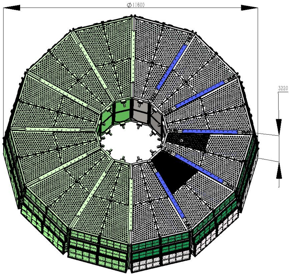
图 1.1-6 自动升降网箱结构图
