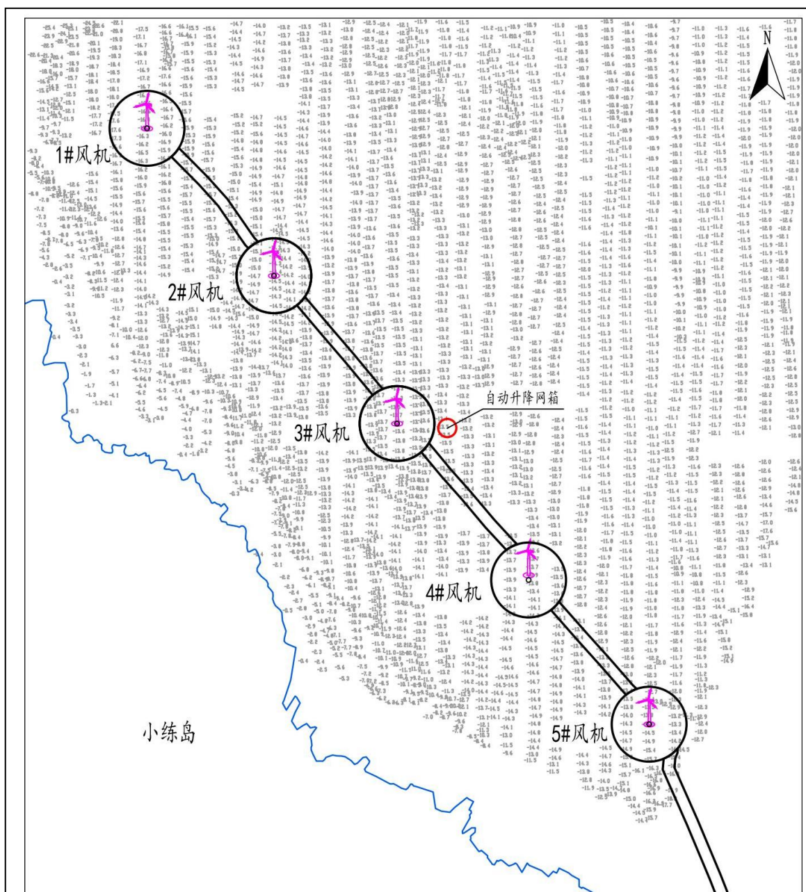
图 1.1-3 本项目附近海域水深地形图
