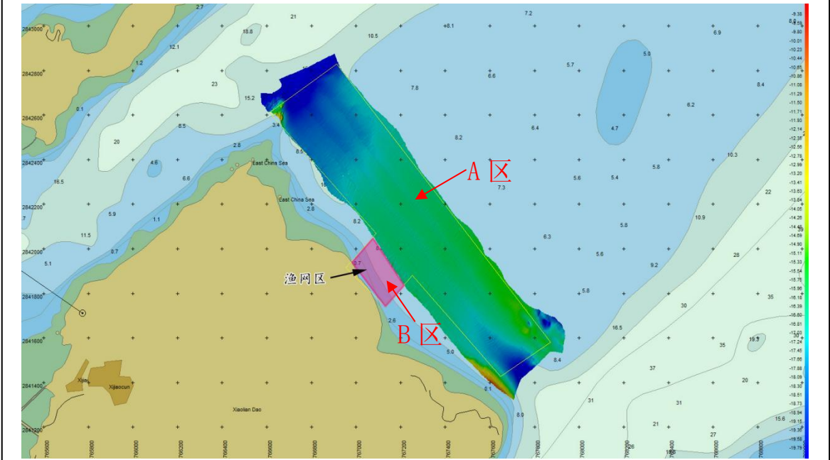
图5.2-5 多波束测深系统扫测图
