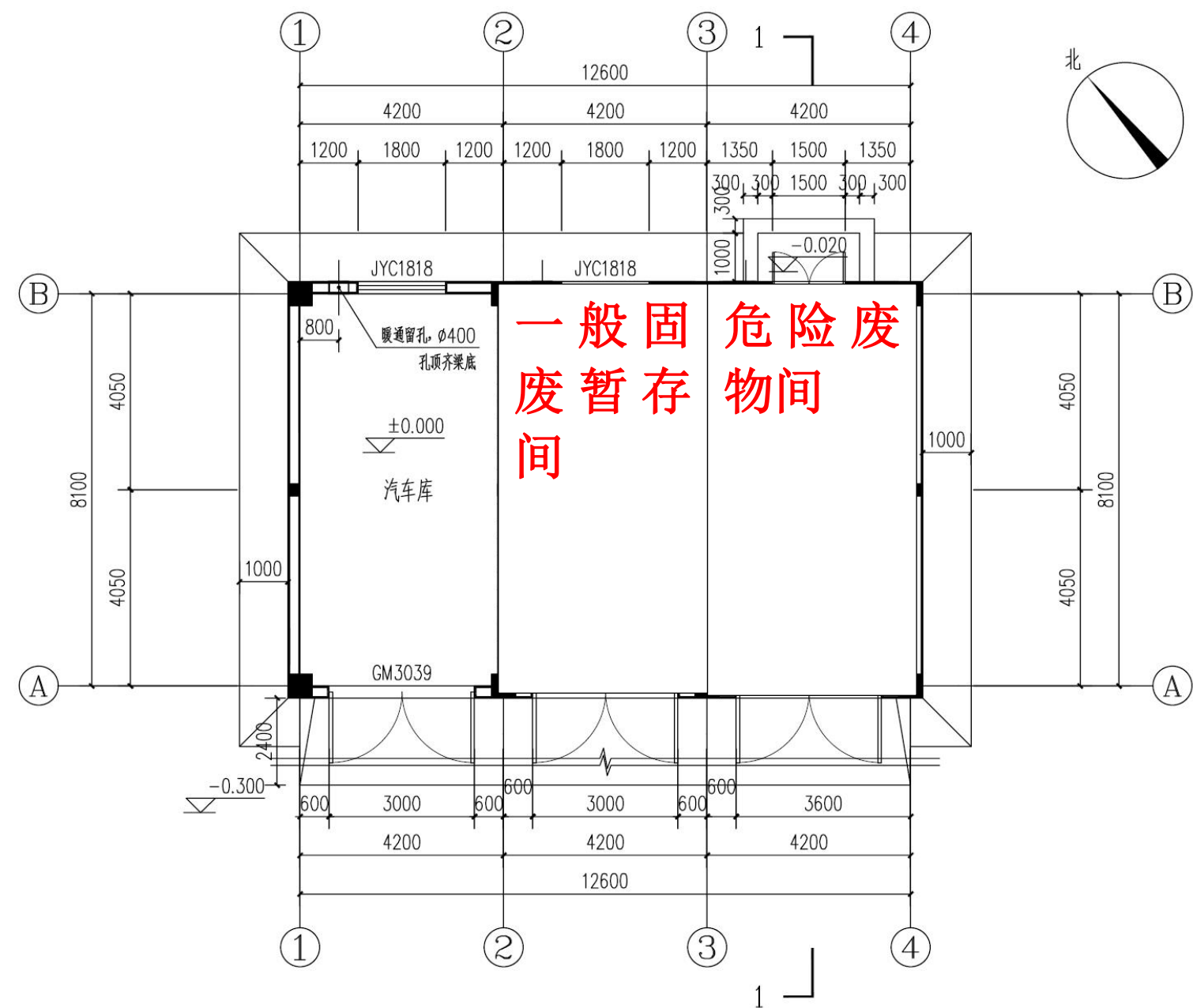
辅助用房一层平面图 1:100
