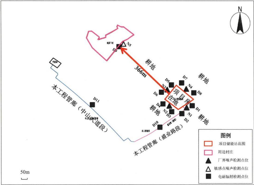
5.2 检测点位示意图
