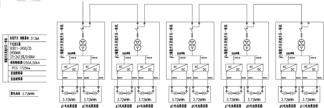
图 2-2 电池连接线示意图
