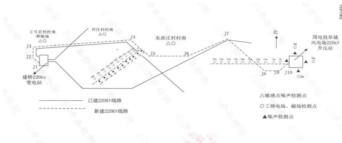
图 3-1 类比项目监测点位图
