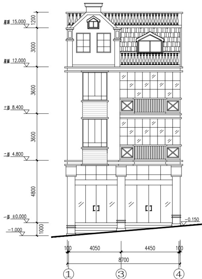
①-④ 轴立面图(变更前)
