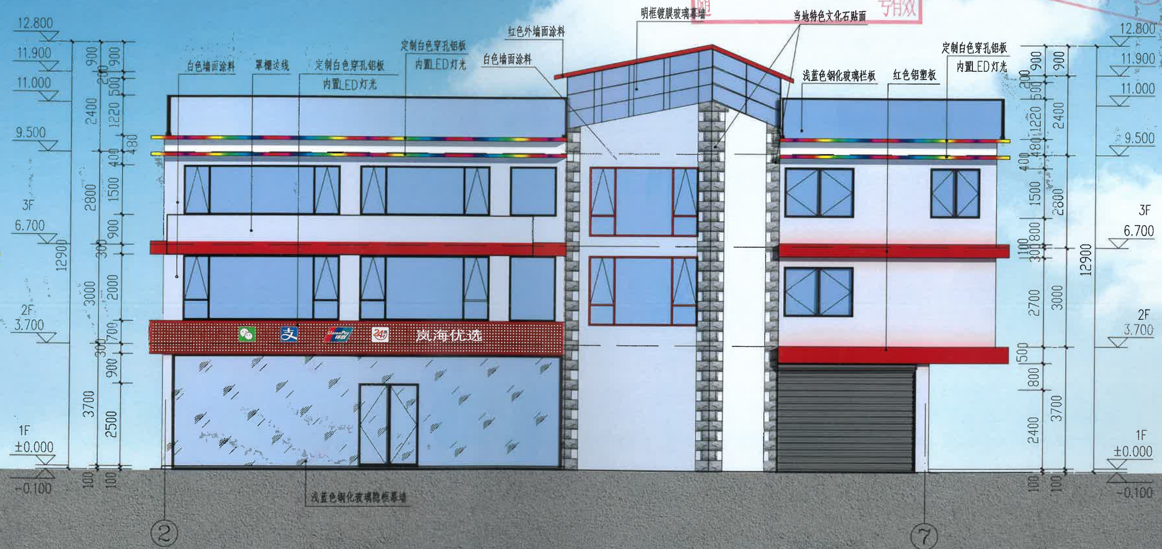
站房②-⑦展开立面图 1:100
