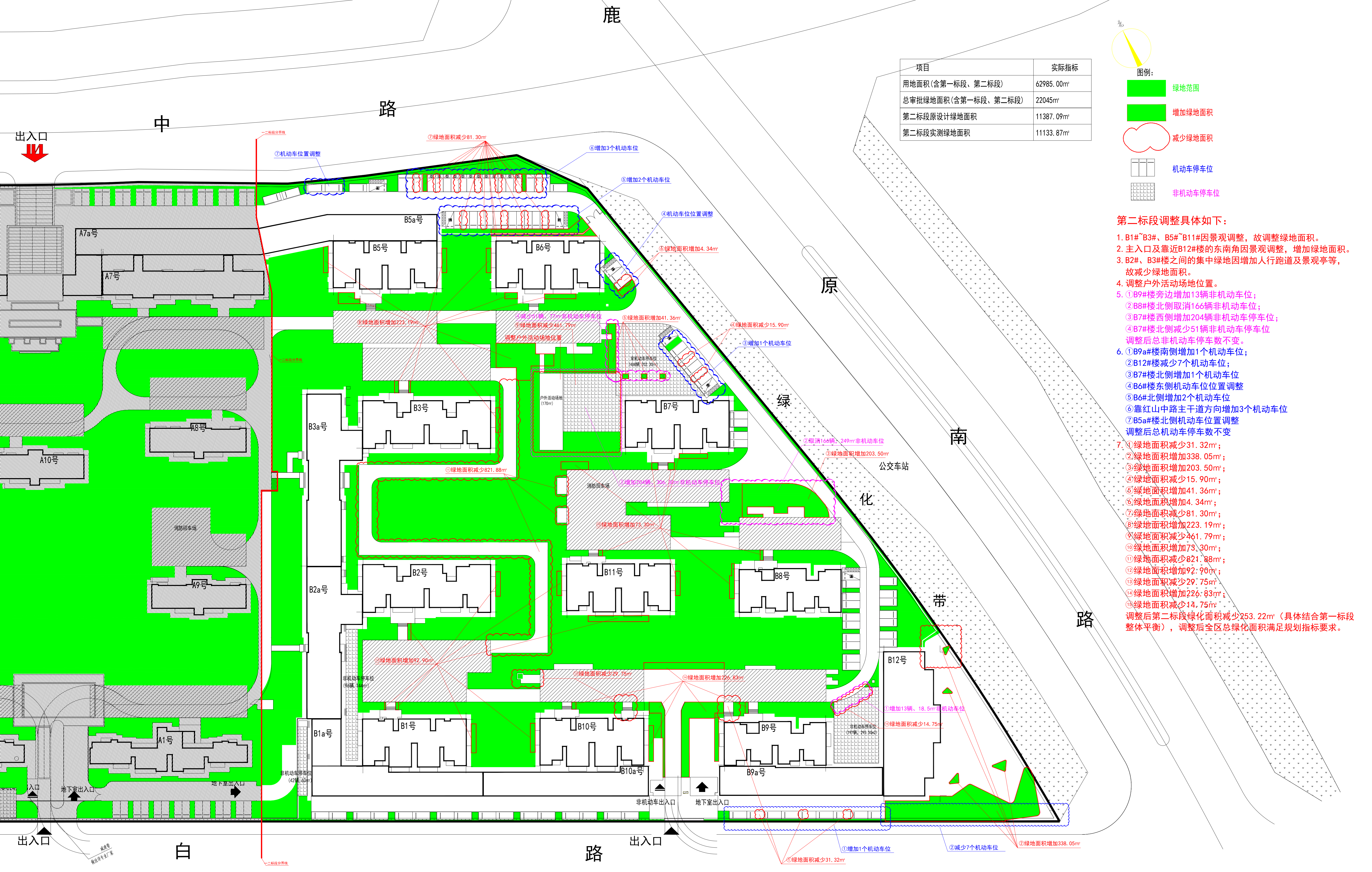
滨海鼎新崇文府第二标段调整后总平面图
