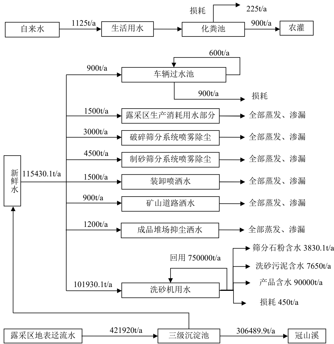
图 3.5-1 项目水平衡图
