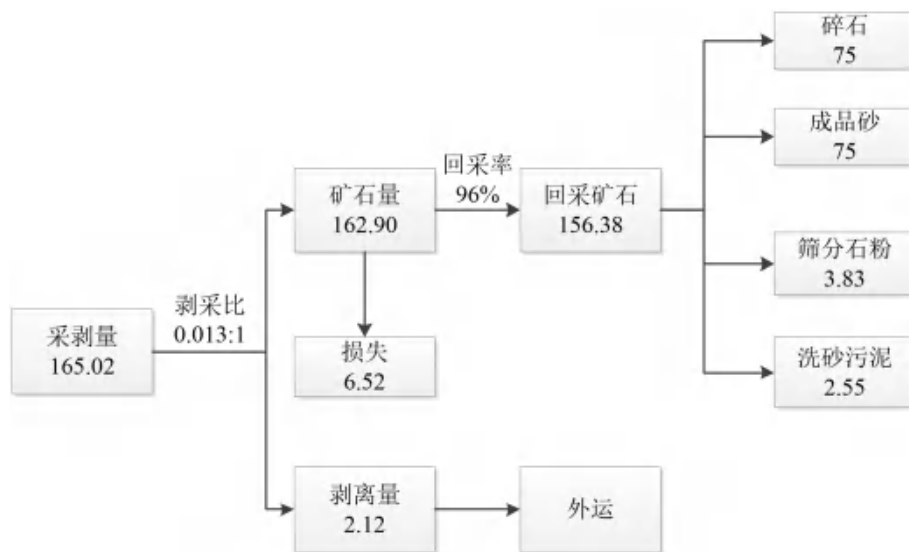
图 3.4-2 项目物料平衡图（单位：万 t/a）
