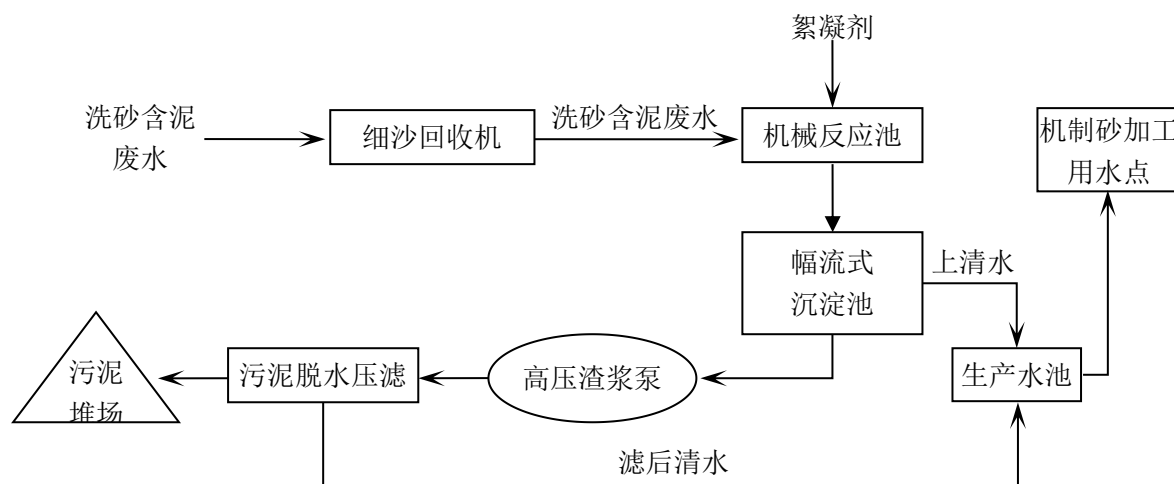
图 8.2-1 洗砂含泥废水处理工艺流程图
