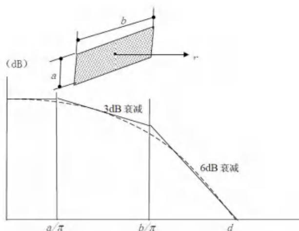
图 6.2-10 长方形面声源中心轴线上的衰减特性
