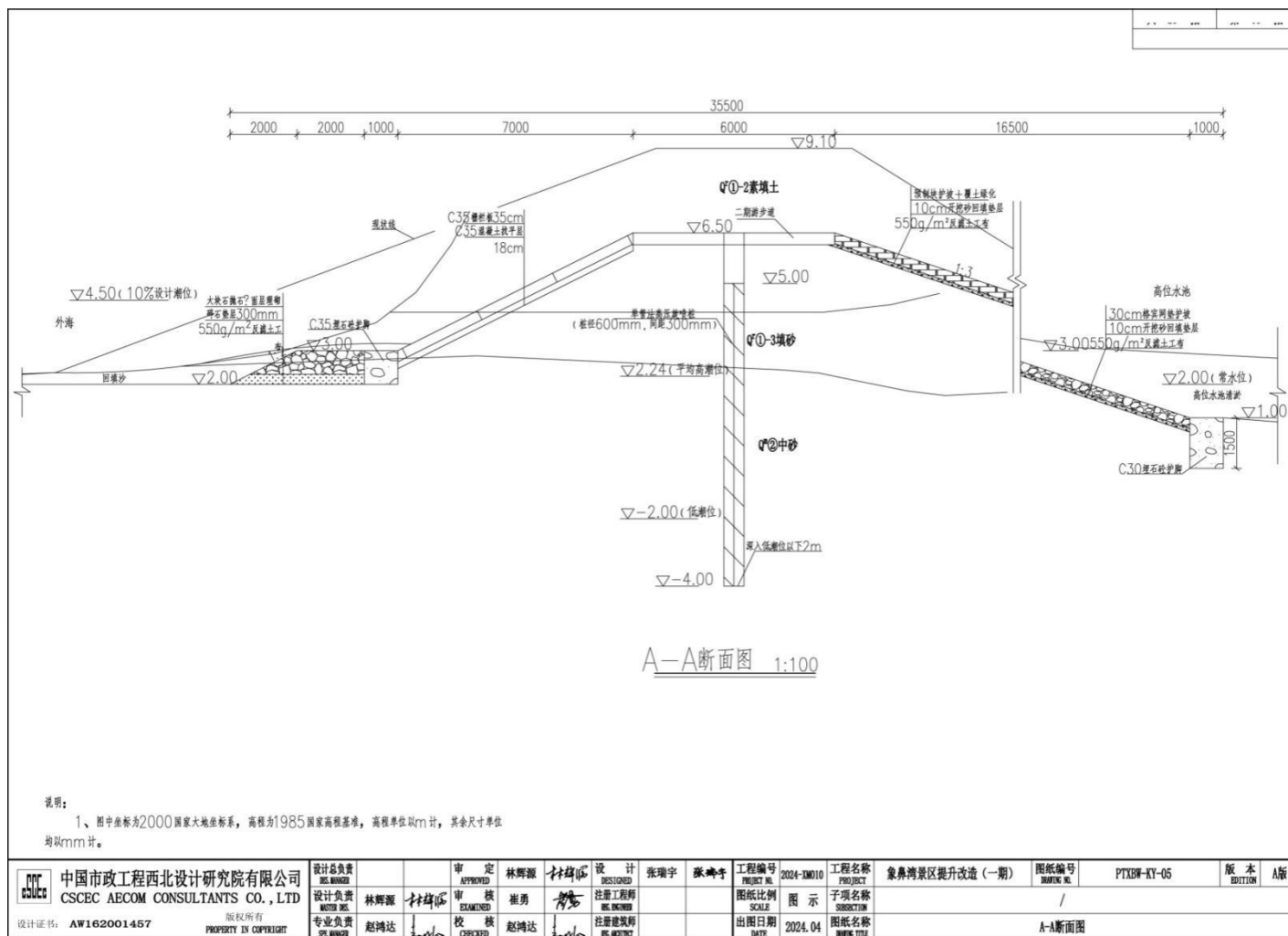
附图 9a 护岸加固断面结构图 (A-A 断面)
