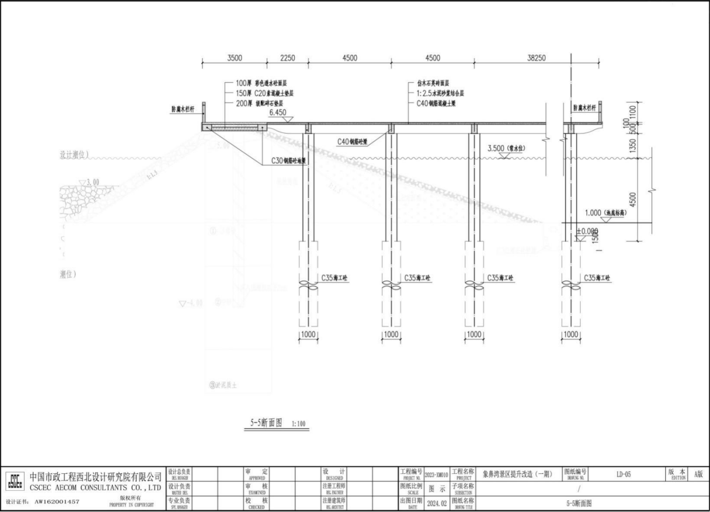
附图 8c 水上栈道典型断面结构图（5-5 断面）
