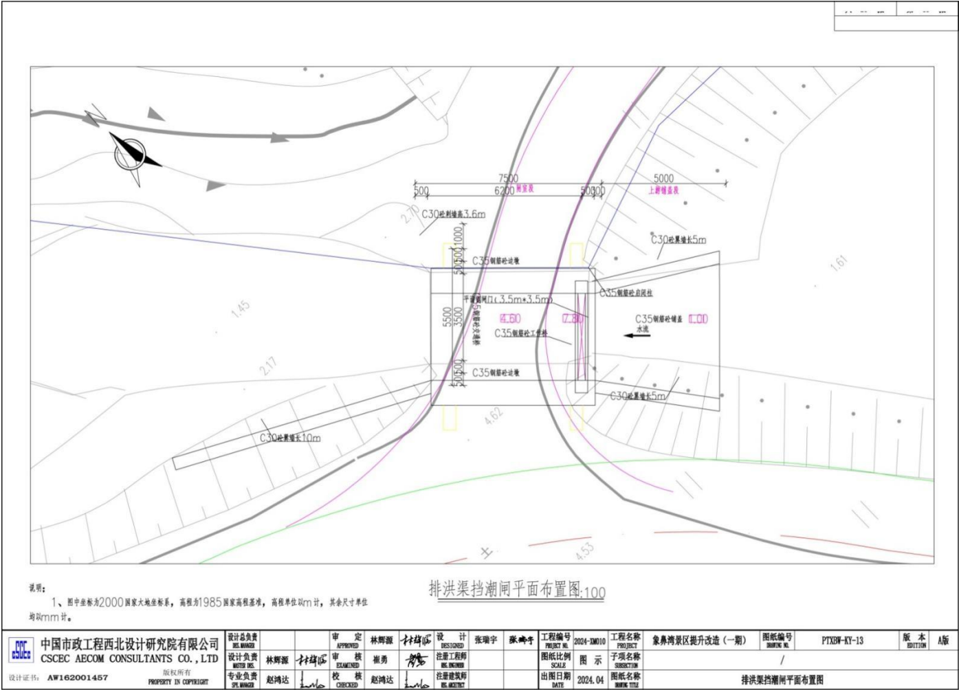
附图 12 排洪渠挡潮闸平面布置图
