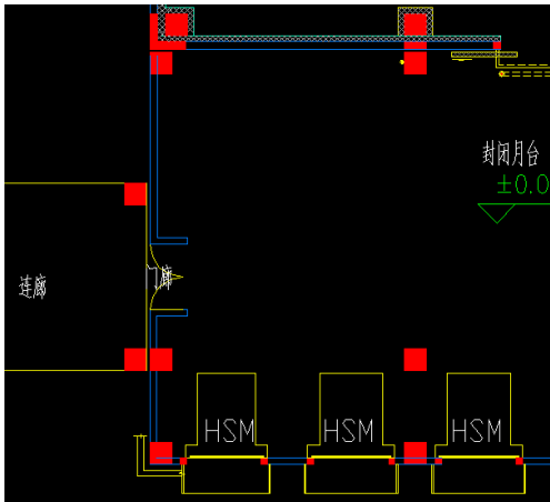
实地建设图纸：
