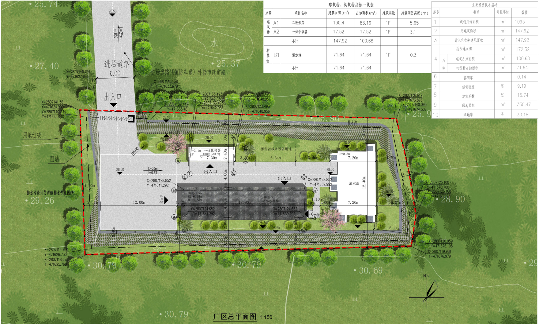
总平面图
