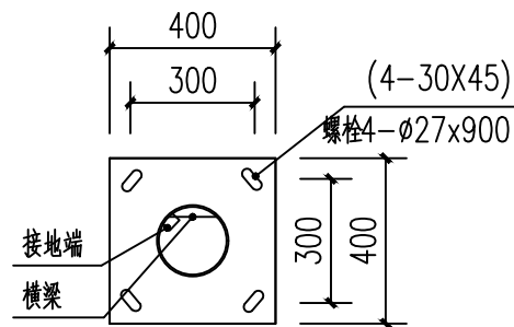
底座法兰平面图
