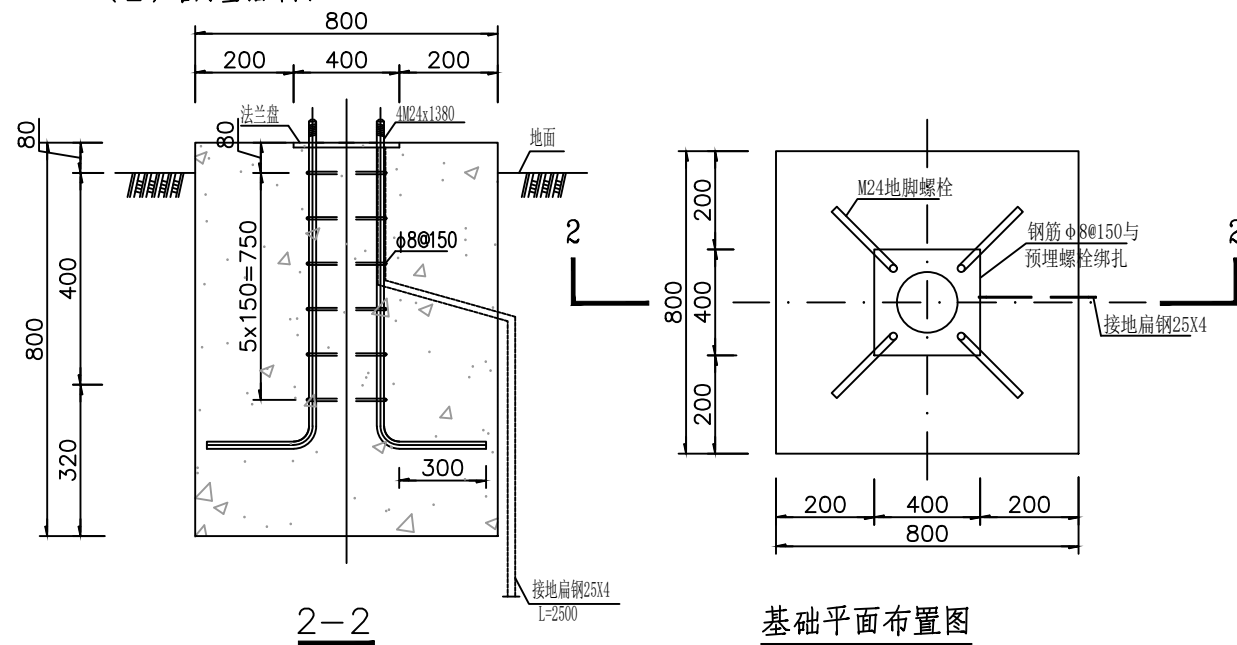
(2) 路灯基础详图
