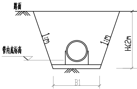
单槽开挖断面
