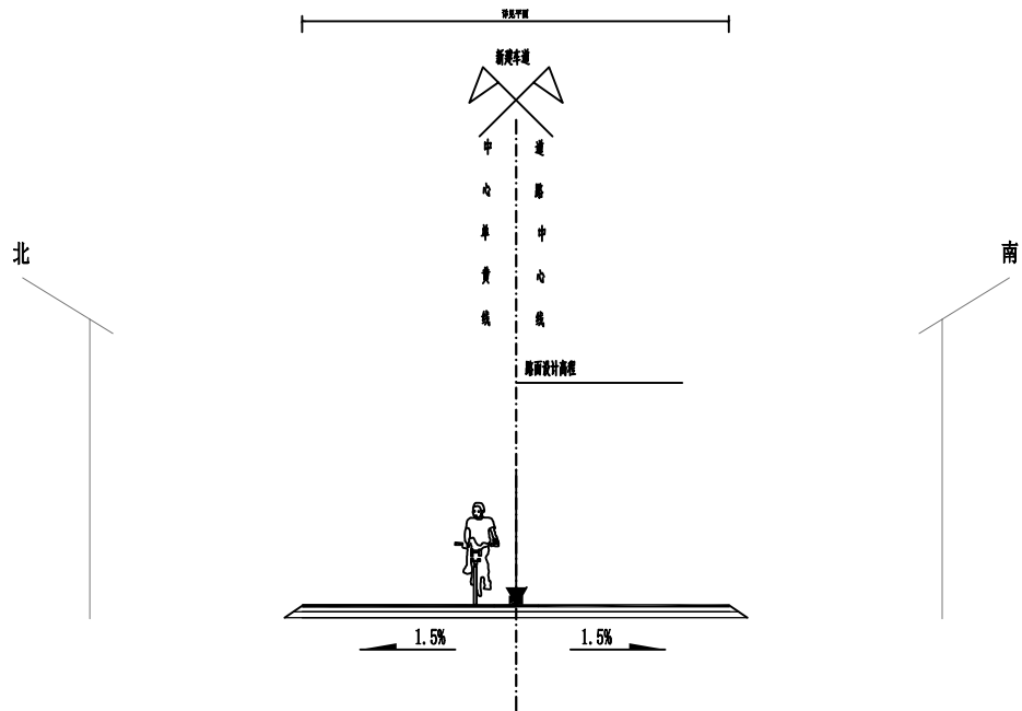
旧路环境提升标准横断面设计图
