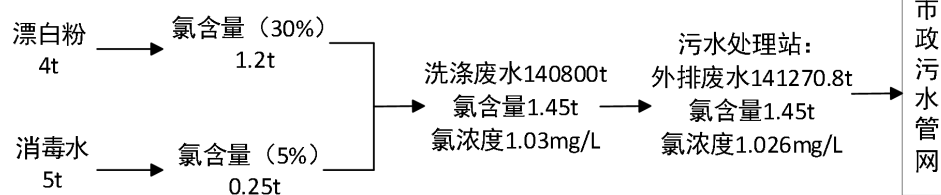
图 2.7-2 项目氯平衡图 (t/a)
