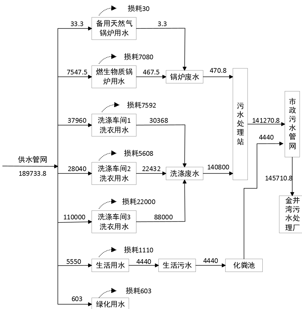
图 2.7-1 项目水平衡图（t/a）
