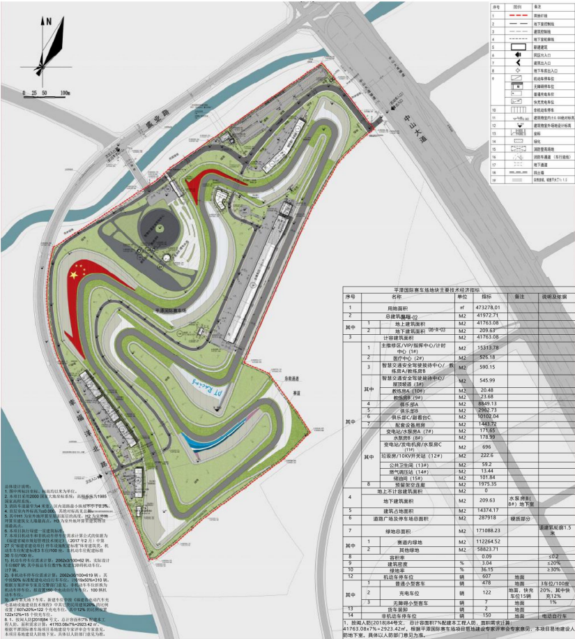
变更前报批总平
