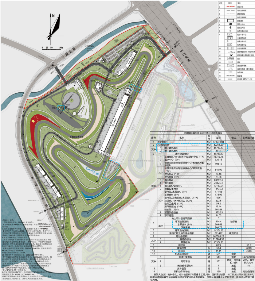
变更后报批总平
