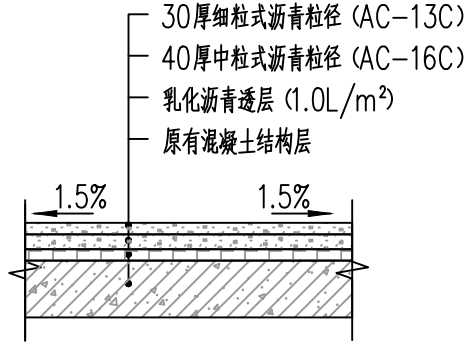
2 车行透水沥青道路做法二 1:20
