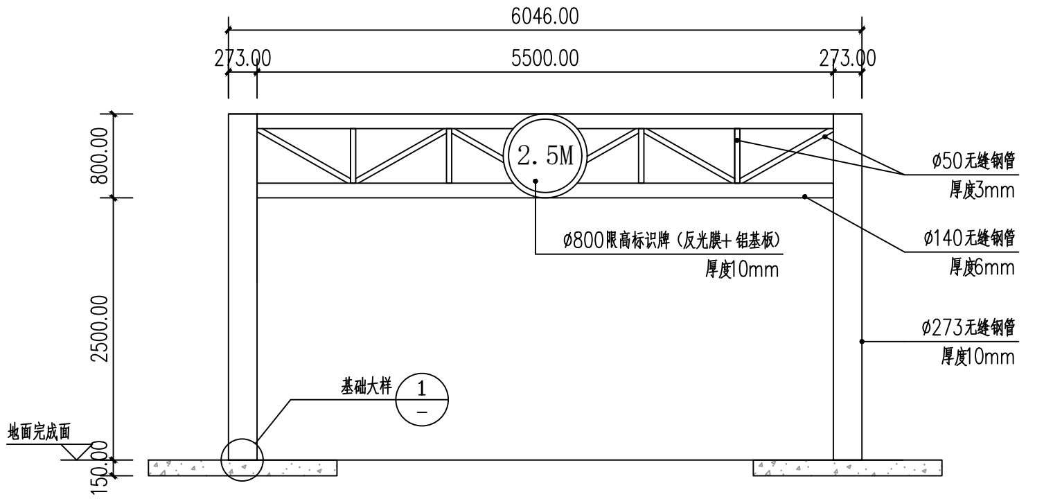
限高杆示意图 1:50
