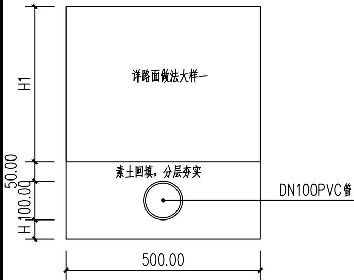
4 管道预埋断面 1:10
