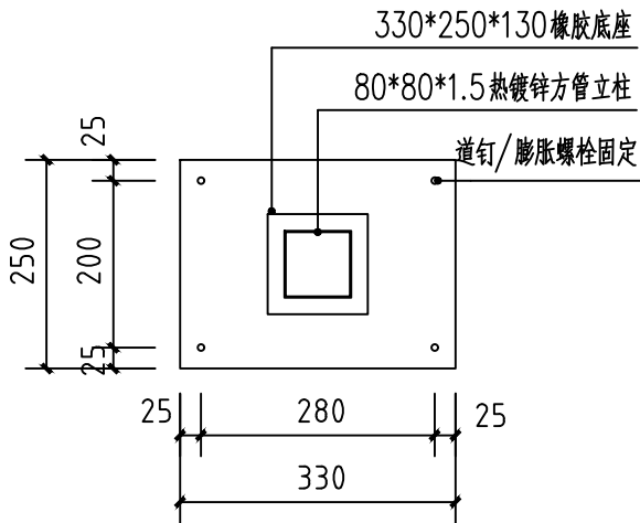
橡胶底座示意图 1:5
