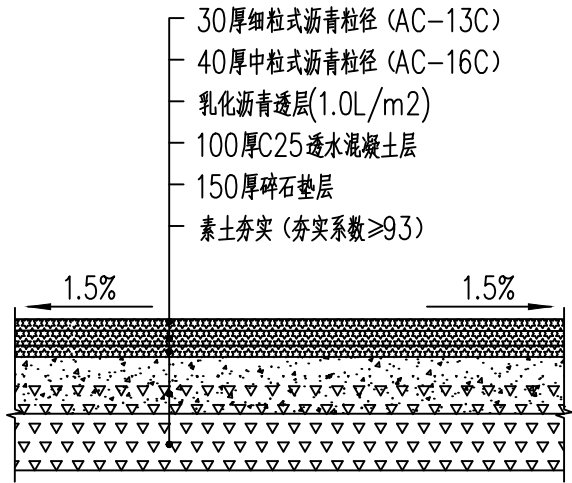
1 车行透水沥青道路做法一 1:20
