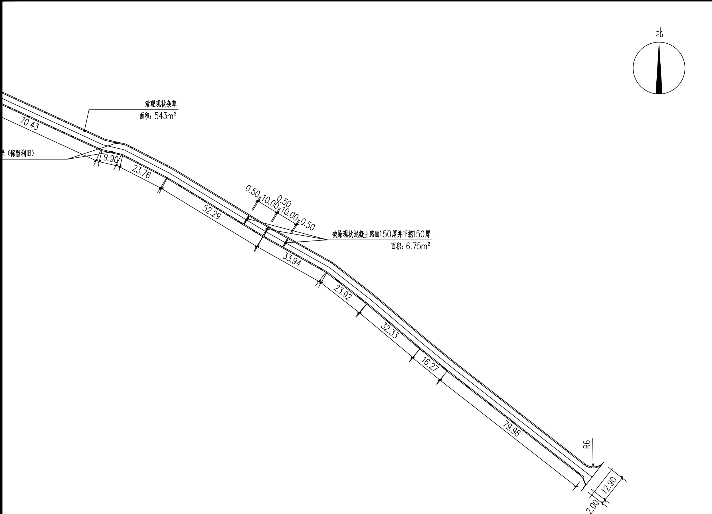
现状总平面图二
