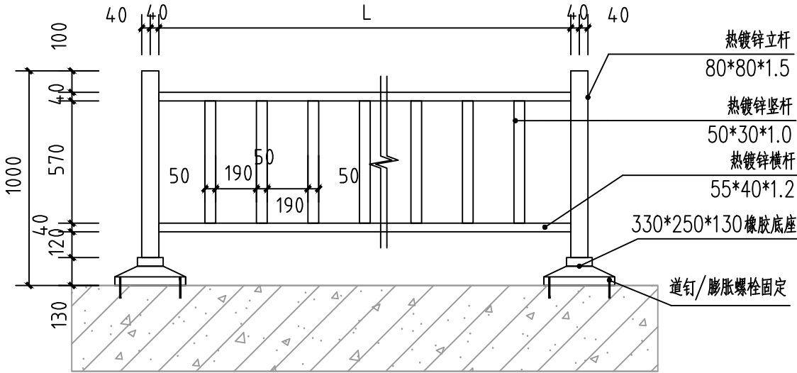
2 — 行车道路护栏大样 1:25
