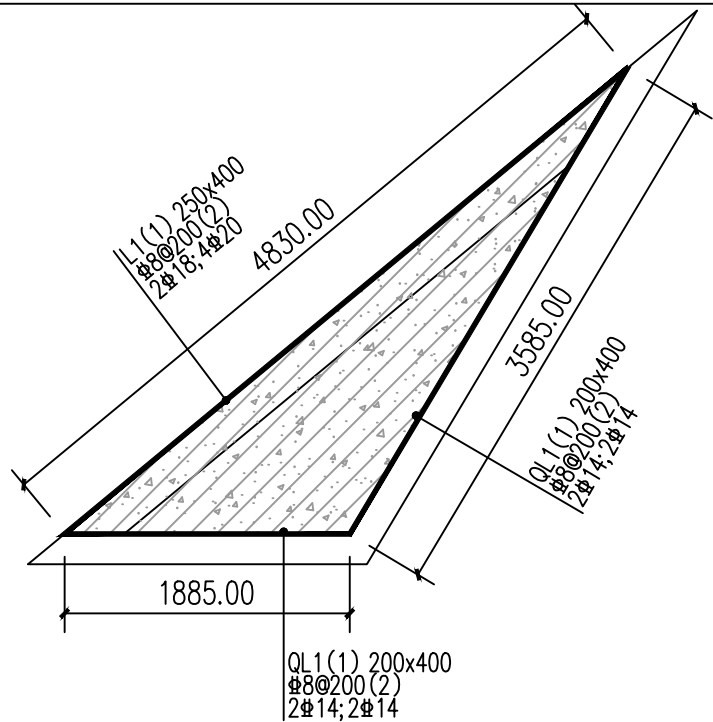
1 — 混凝土板配筋大样 1:50
