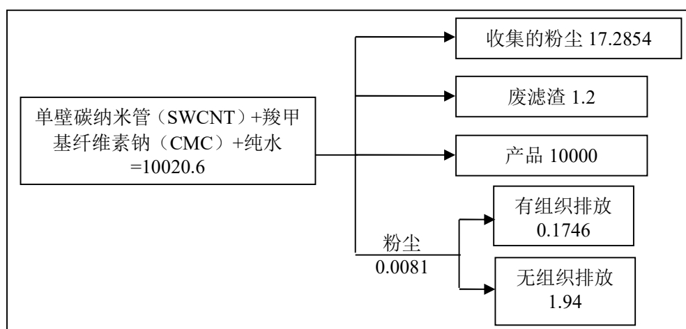
图 2-2 物料平衡图（单位：t/a）
