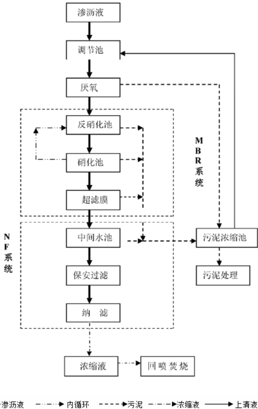
图 2.2-4 垃圾渗滤液处理工艺流程图
