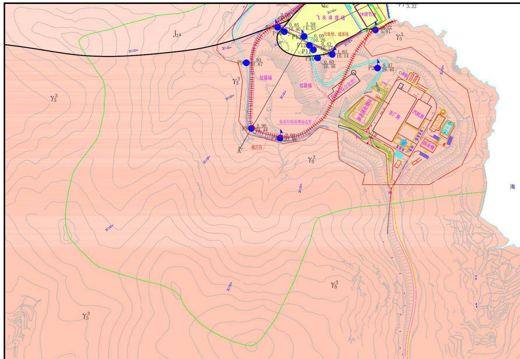
图 3.3-3 场地水文地质图
