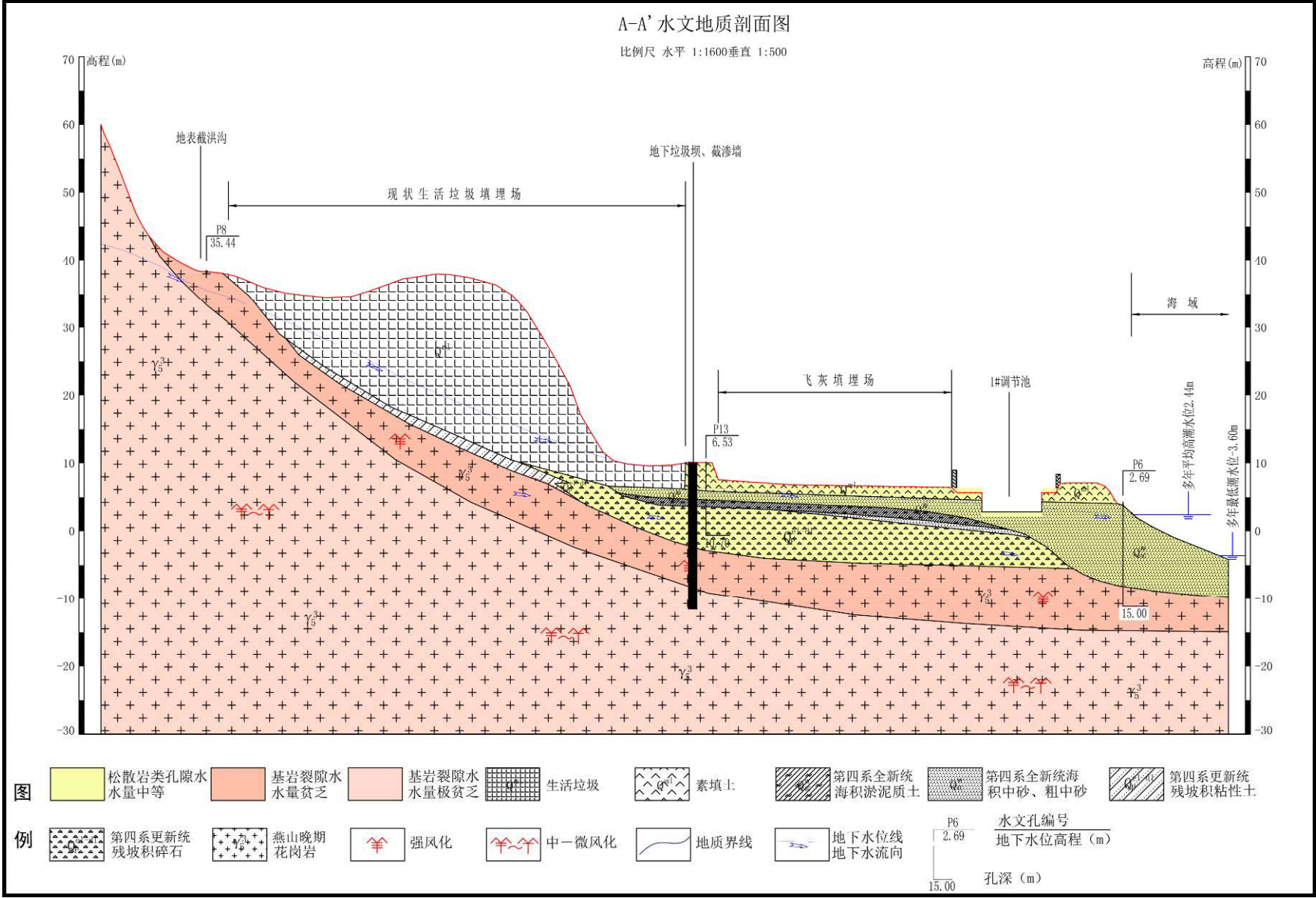
图 3.3-4 场地水文地质剖面图
