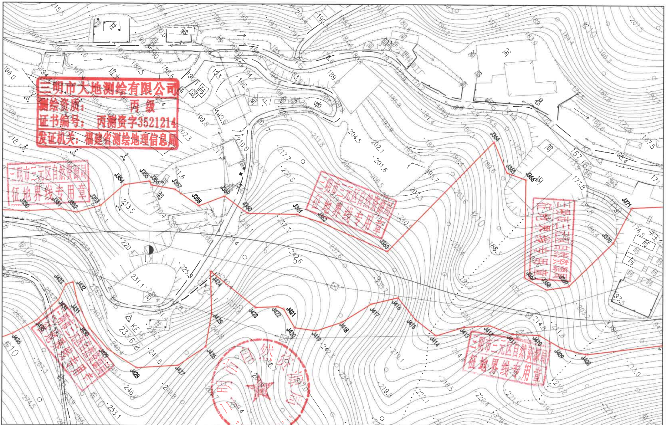
国道534（横六线）三元区村头至荆东二期工程勘测定界图
