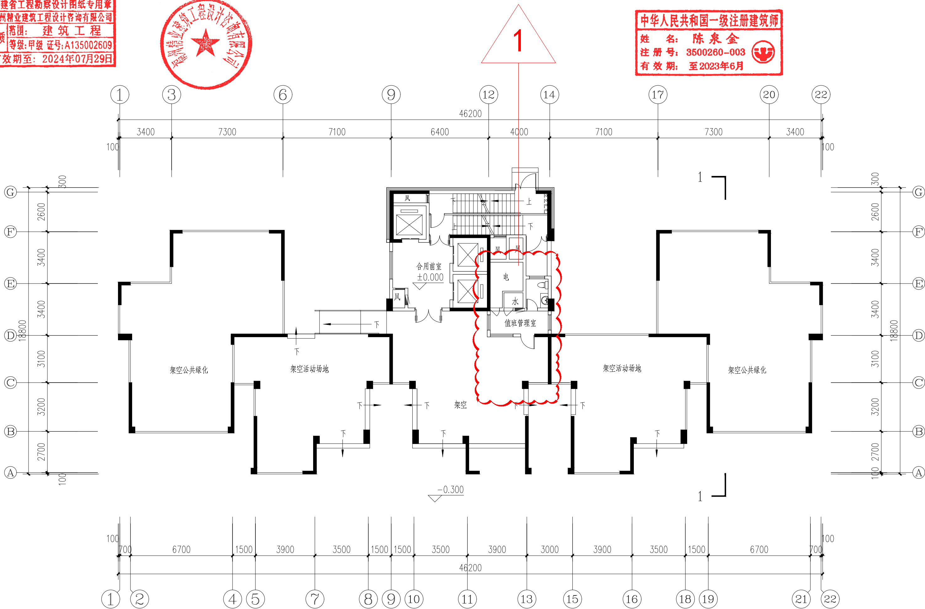
一层平面图
