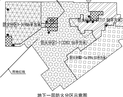
地下一层防火分区示意图
