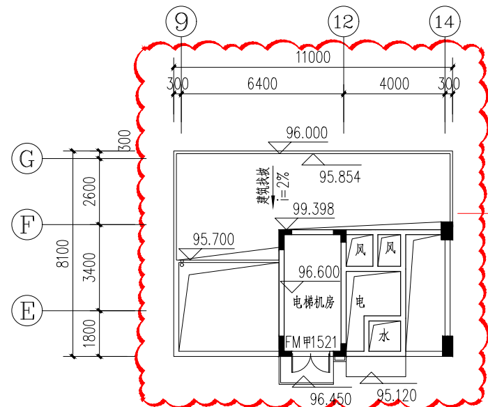
楼梯间屋面平面图
