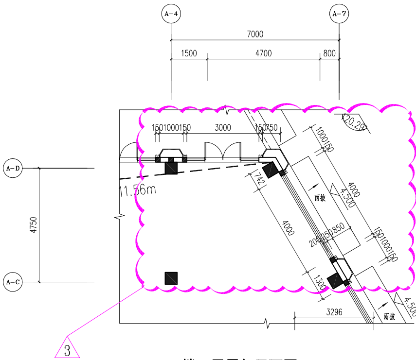
2-1#楼二层局部平面图一 (变更前)
