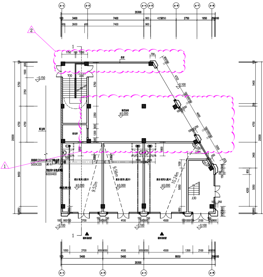
2-1#楼一层平面图 (变更前)
