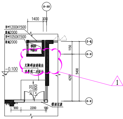
2#楼一层局部平面图一 (变更前)
