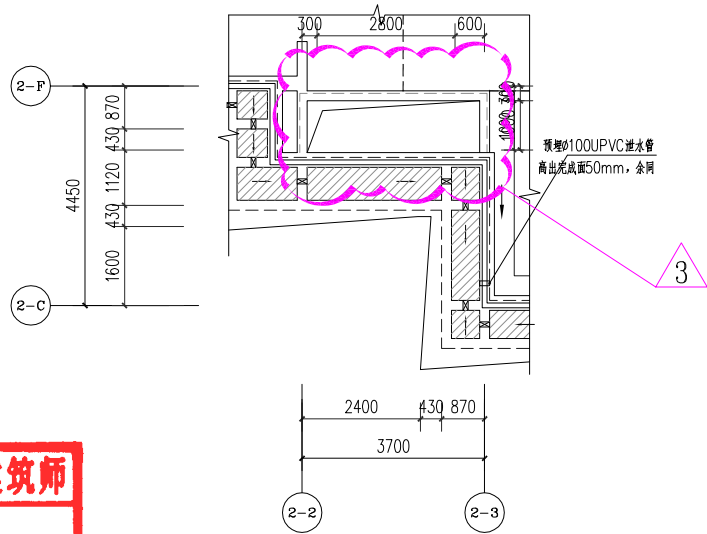
2#楼屋面层局部平面图一 (变更后)
