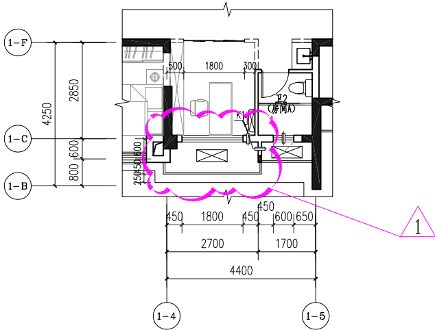
1#楼二至二十四层局部平面图一 (变更后)
