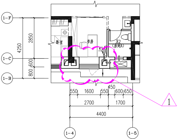
1#楼二至二十四层局部平面图一 (变更前)
