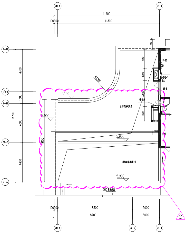
2#楼二层局部平面图一 (变更前)
