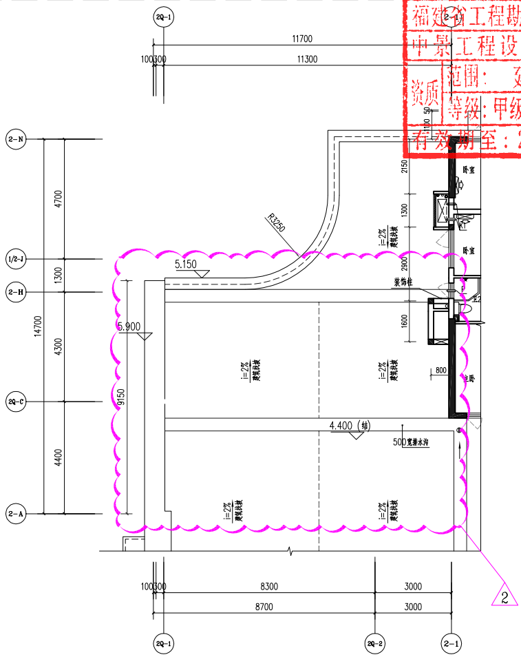
2#楼二层局部平面图一 (变更后)
