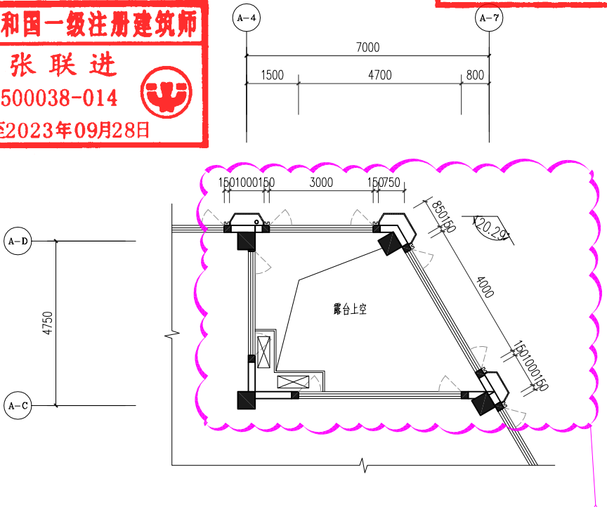
2-1#楼三层局部平面图一 (变更后)
