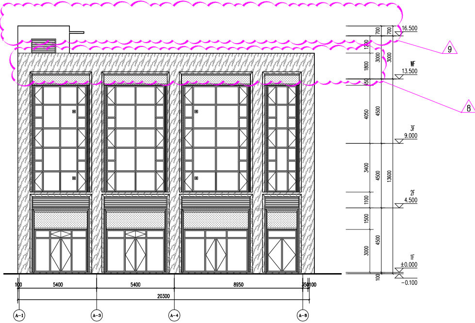
A-1~A-8轴立面图 (变更后)
