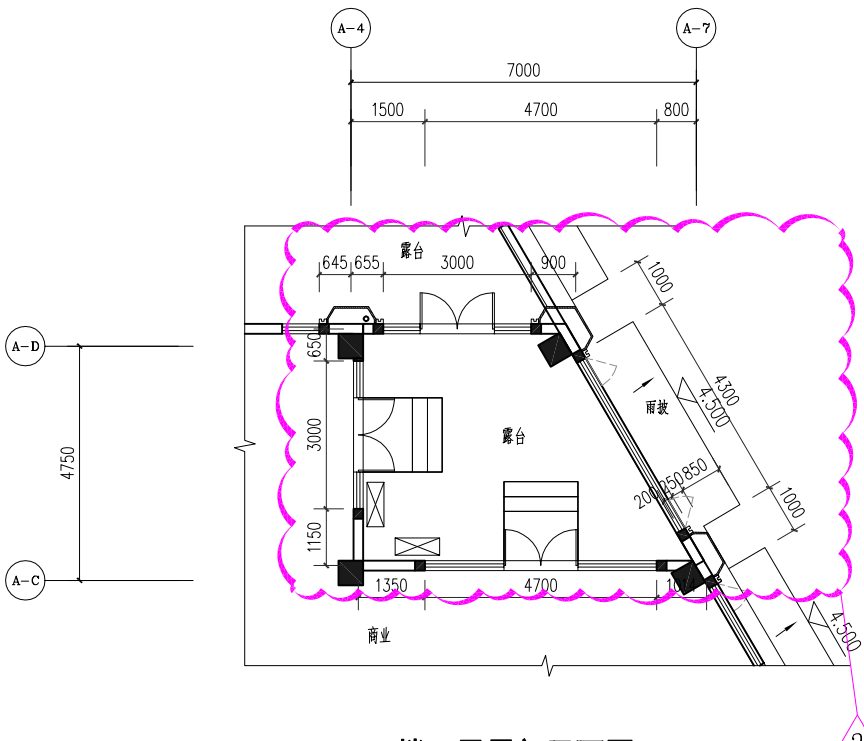
2-1#楼二层局部平面图一 (变更后)
