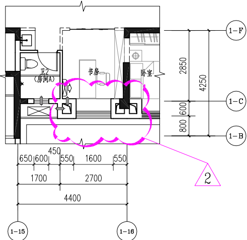
1#楼二至二十四层局部平面图二 (变更前)
