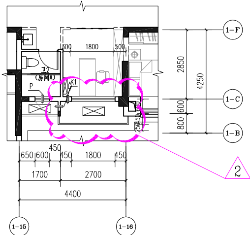
1#楼二至二十四层局部平面图二 (变更后)
