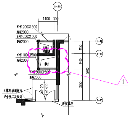
2#楼一层局部平面图一 (变更后)
