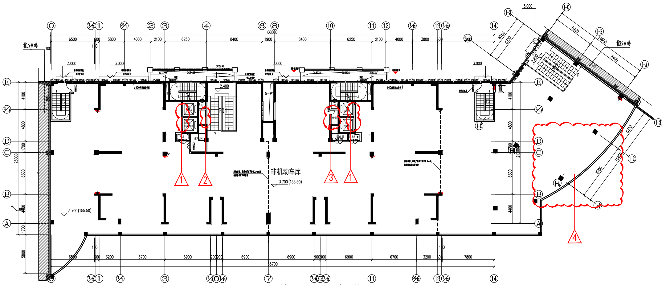
5#楼二层平面图 变更前
