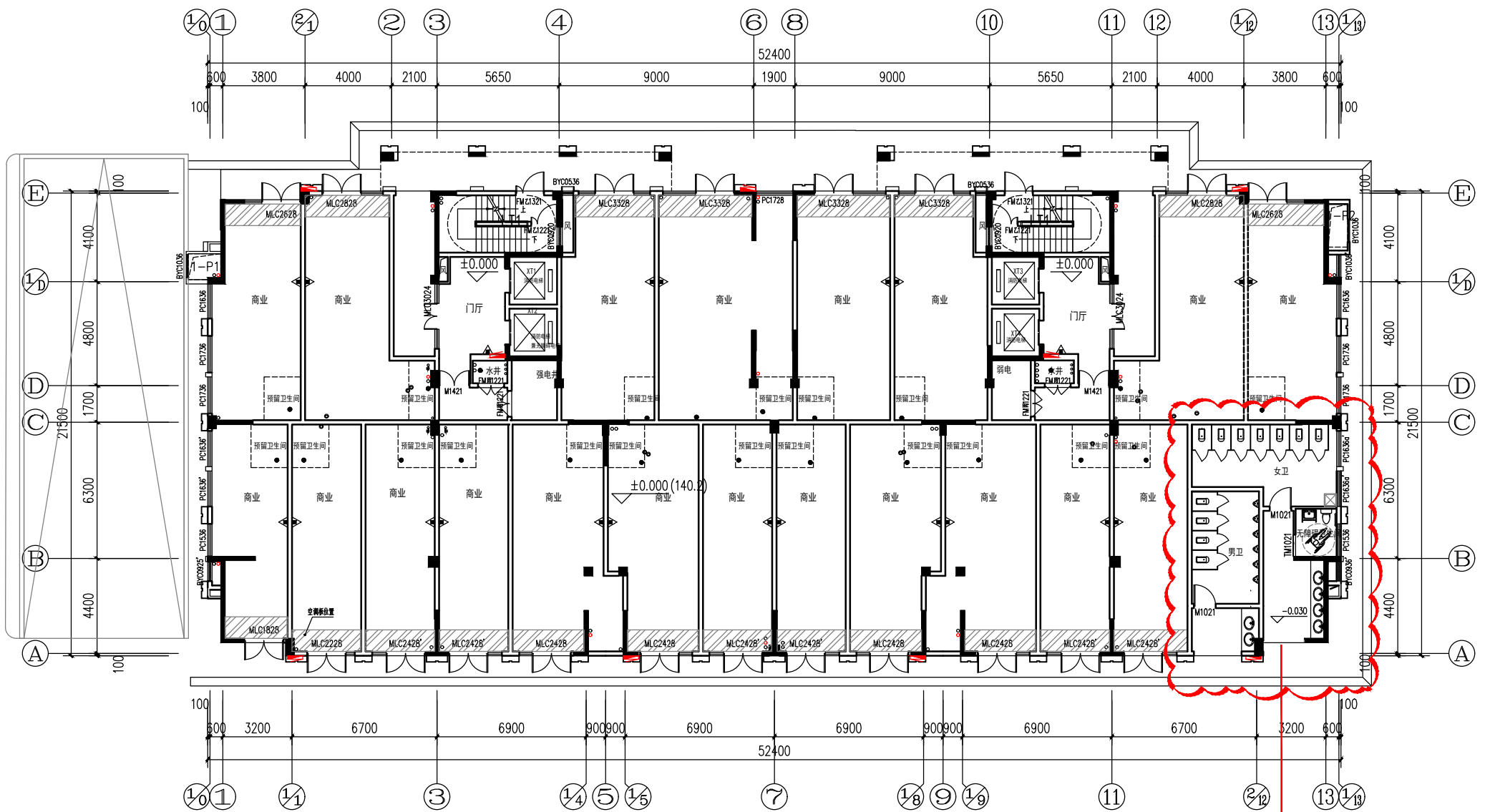
1#楼一层平面图 变更后 阴影部分为商业门口上方空调板位置
