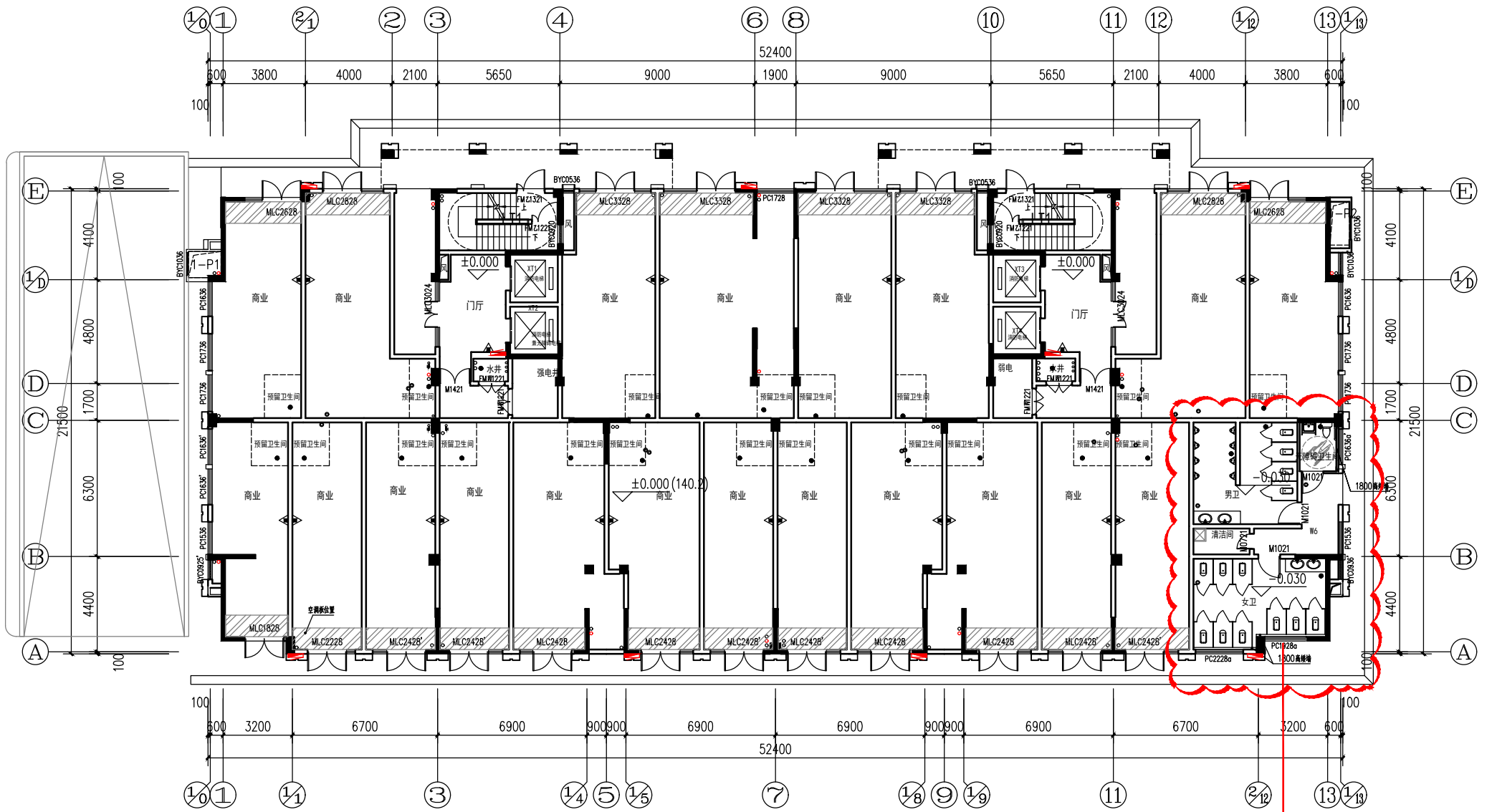
1#楼一层平面图 变更前 阴影部分为商业门口上方空调板位置
