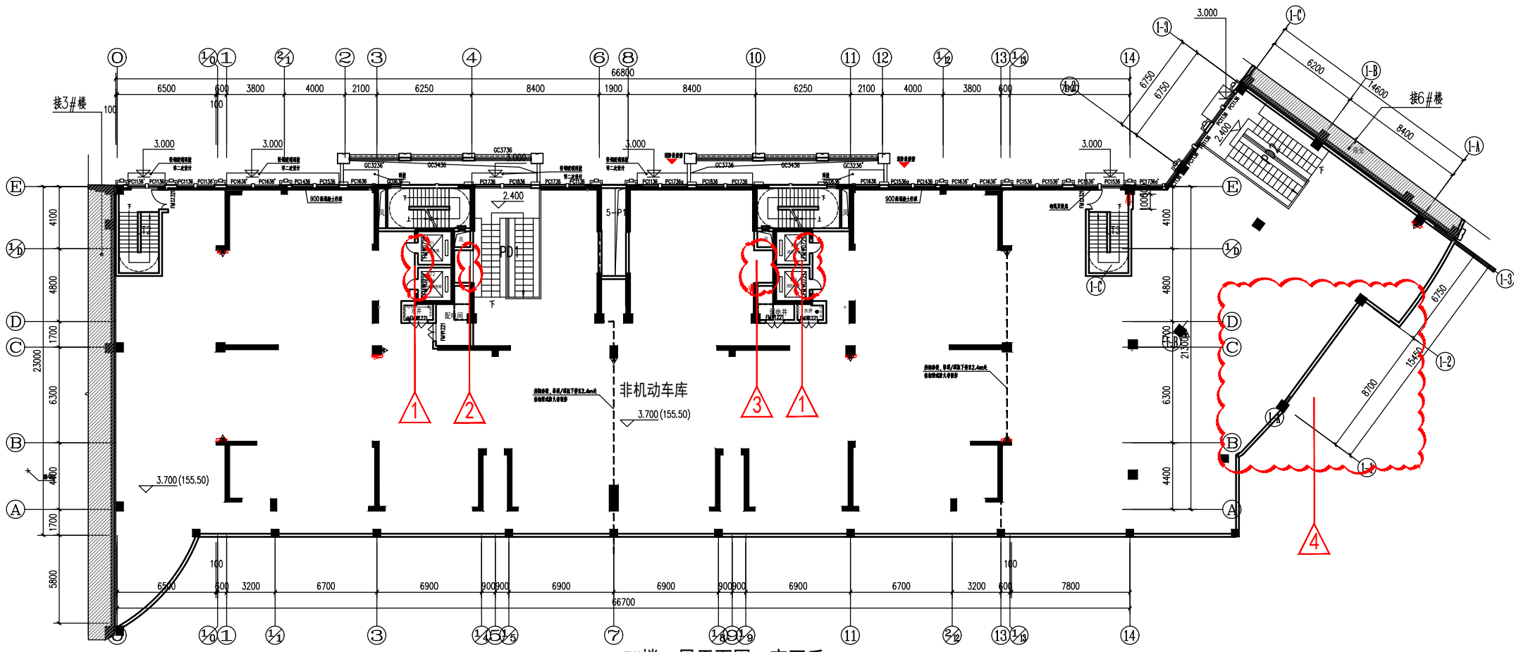
5#楼二层平面图 变更后
