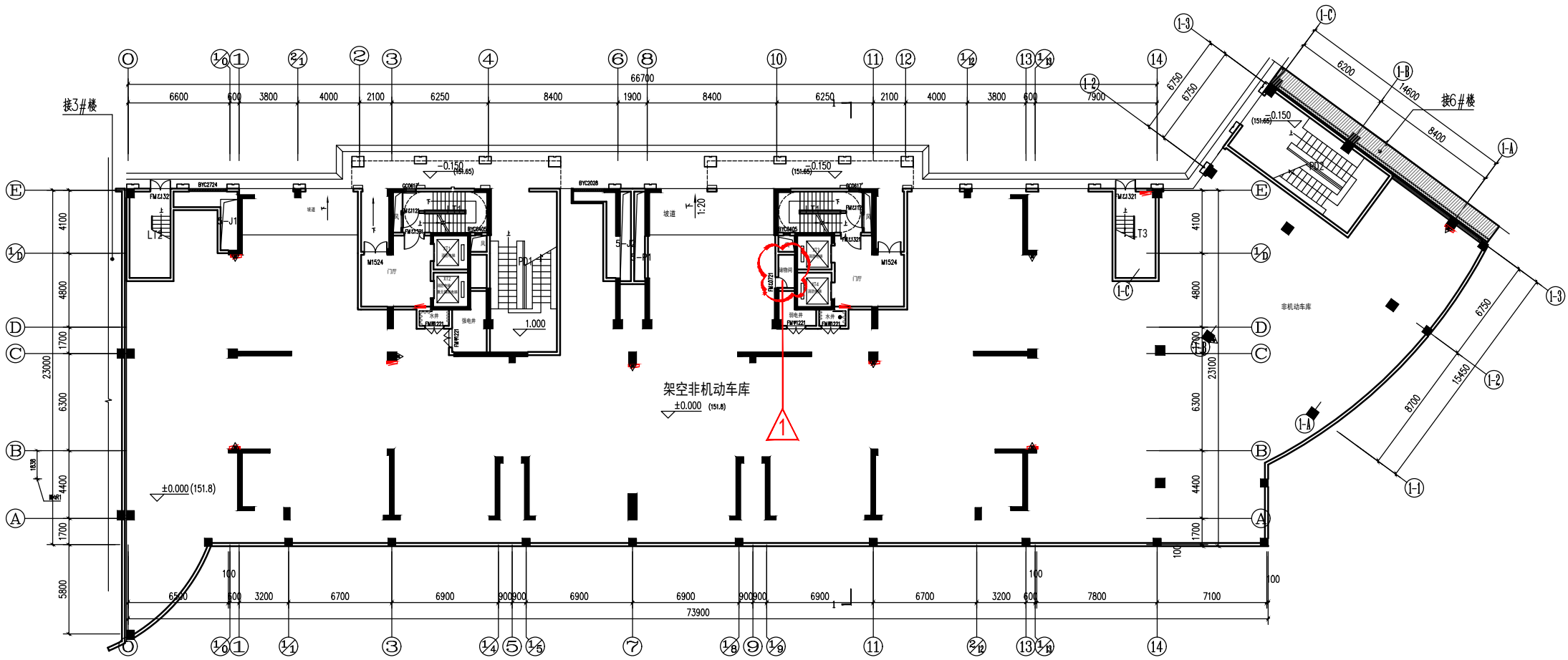
5#楼一层平面图 变更前
