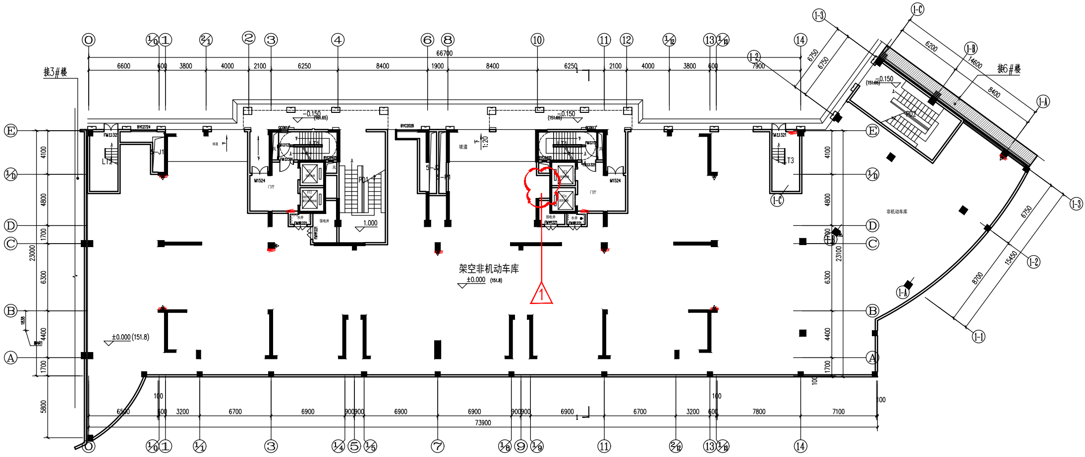
5#楼一层平面图 变更后
