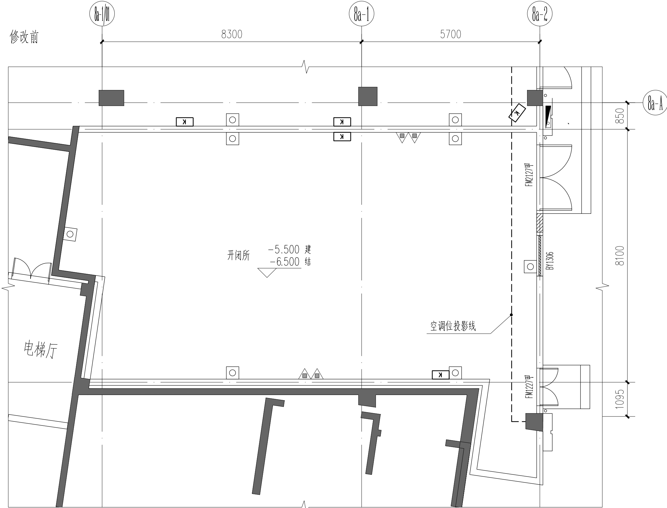
8#楼 标高-5. 500局部平面图 1:100
