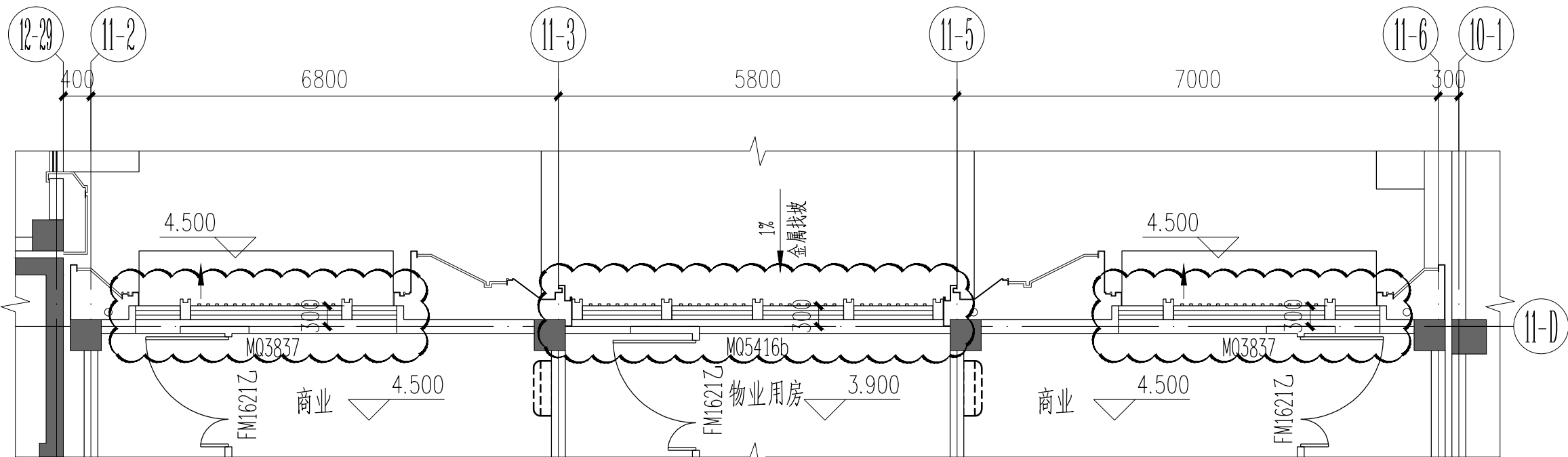
11#楼 二层局部平面图 1:100
