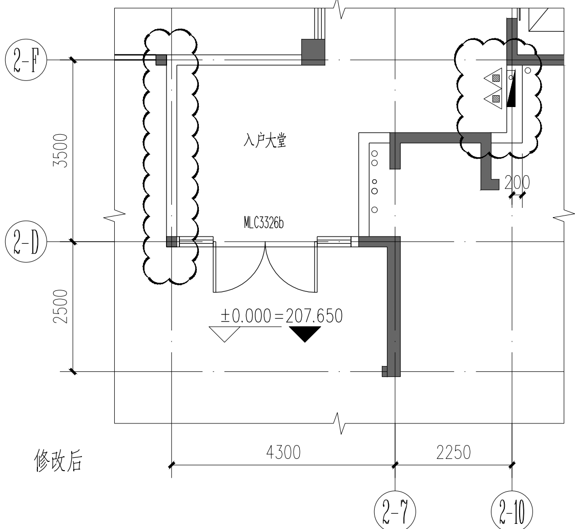
2#楼 一层局部平面图 1:100
