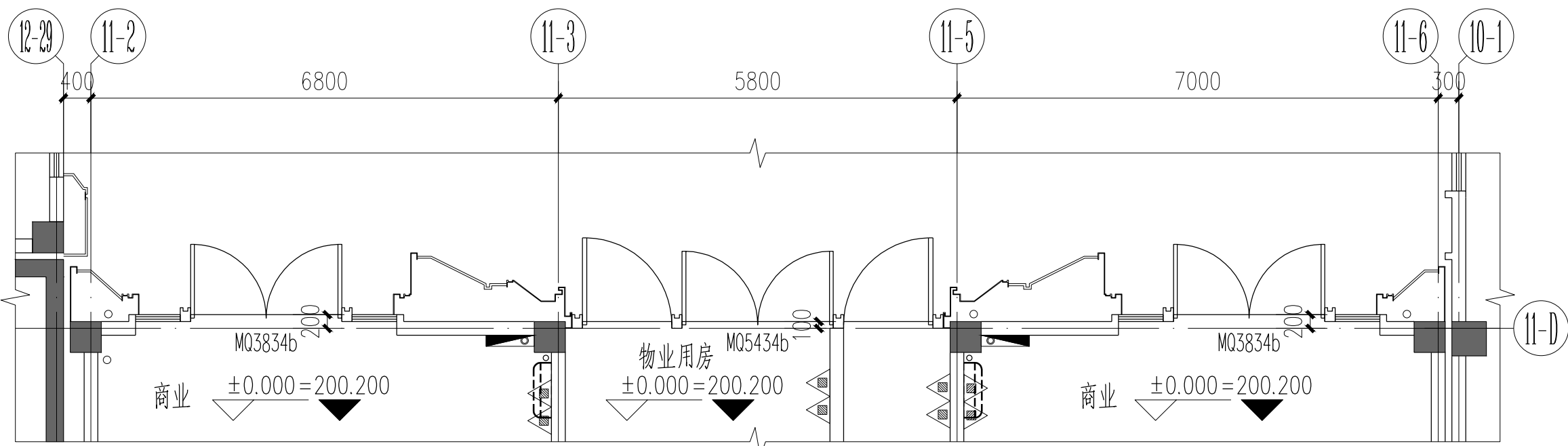
11#楼 一层局部平面图 1:100
