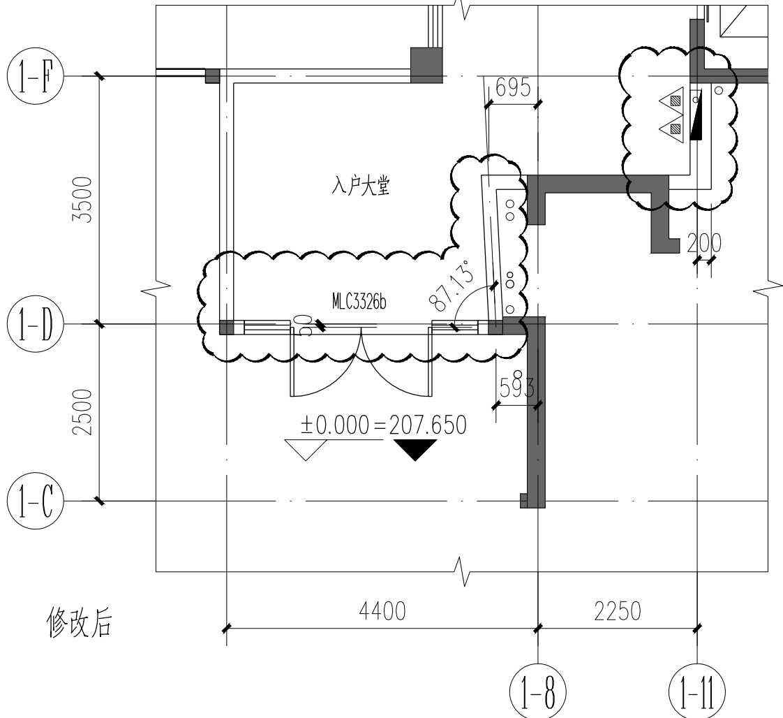
1#楼 一层局部平面图 1:100
