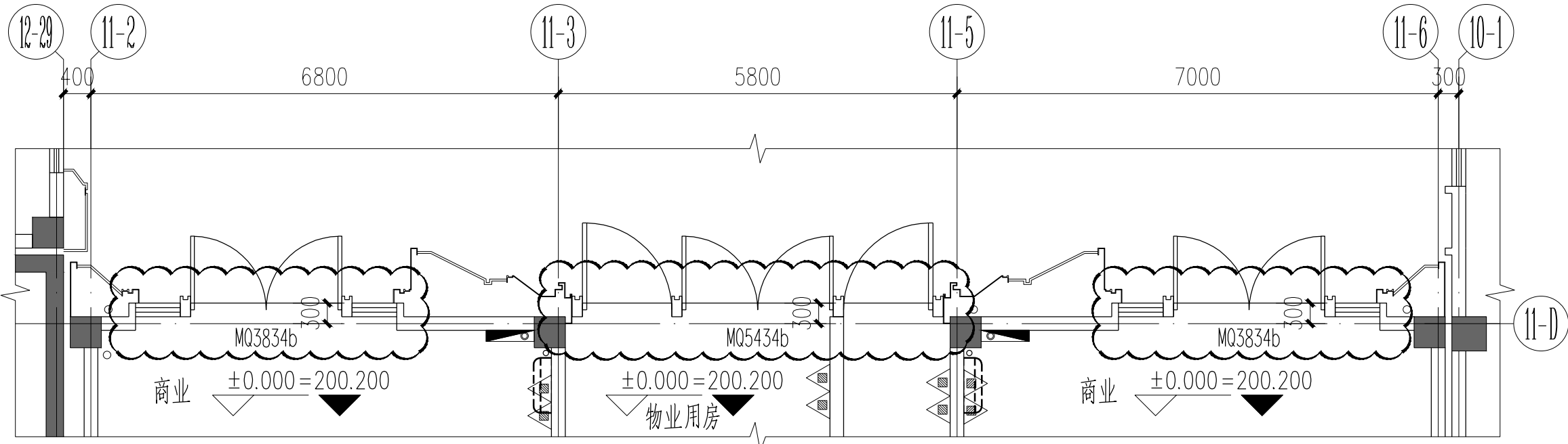
11#楼 一层局部平面图 1:100
