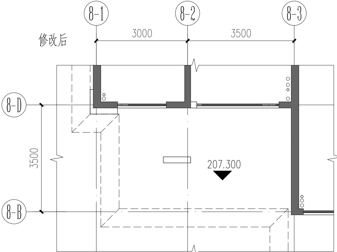
8#楼 一层局部平面图
