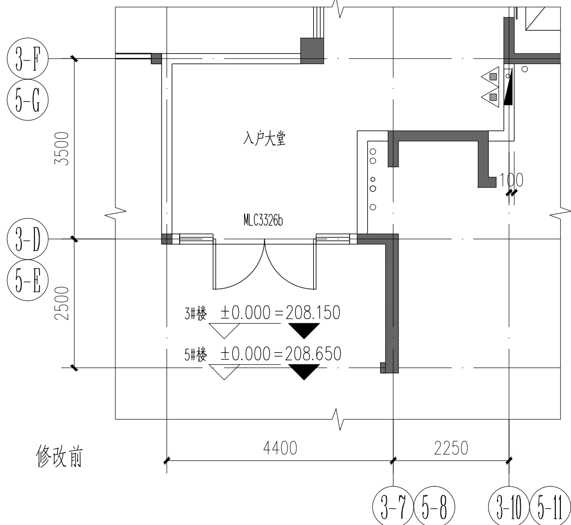
3#、5#楼 一层局部平面图 1:100
