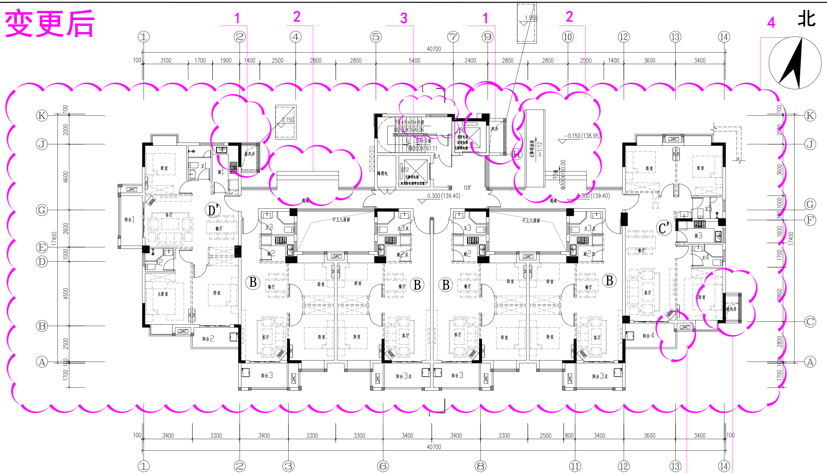
2#楼一层平面图
