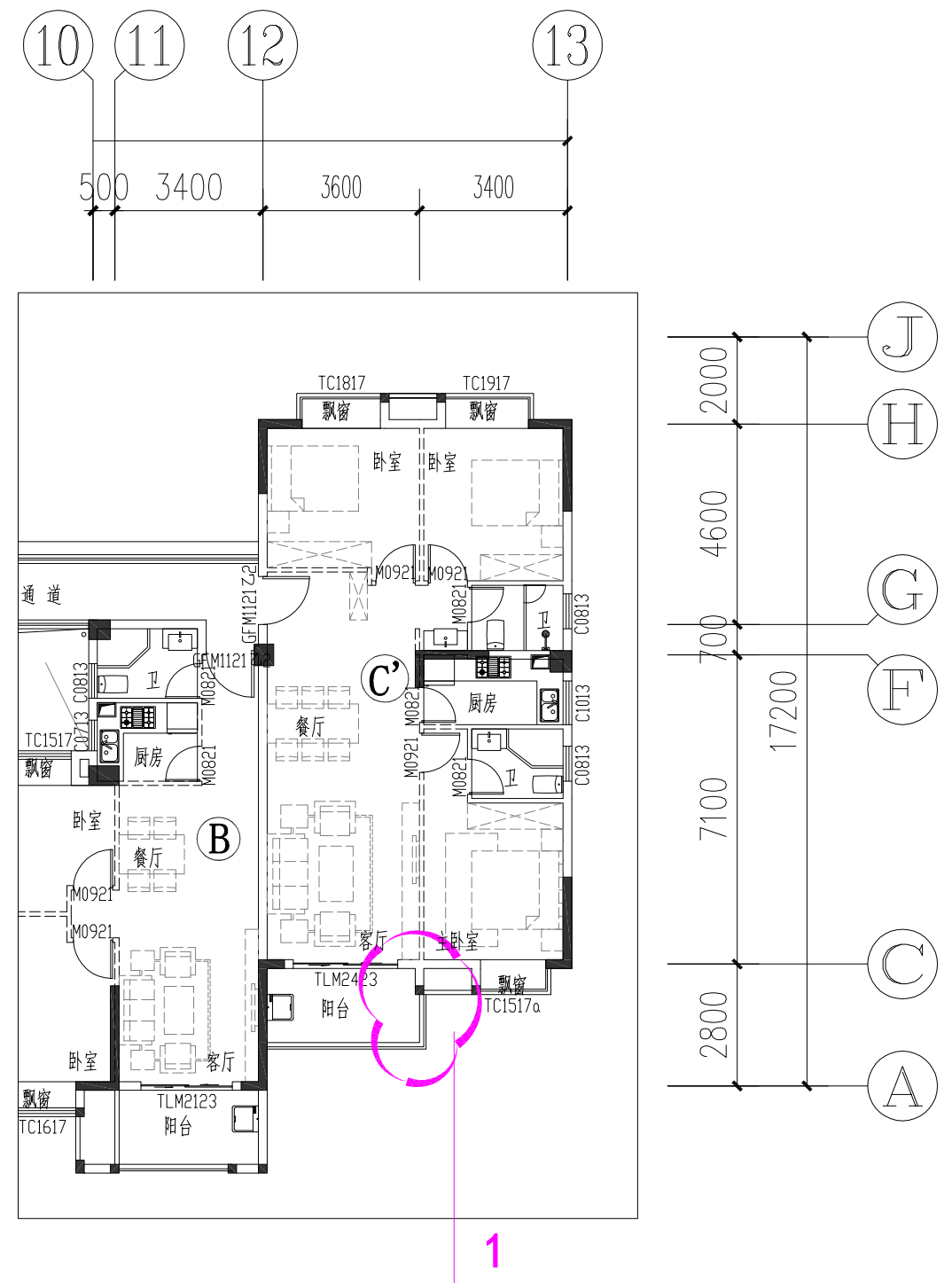
3#楼三~十八层平面图
