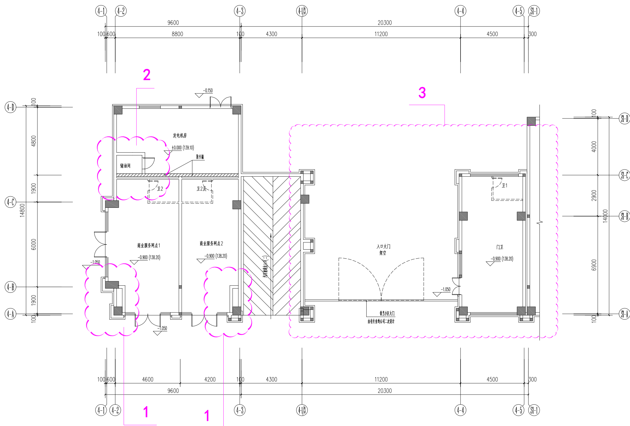
4#楼、门卫一层平面图
