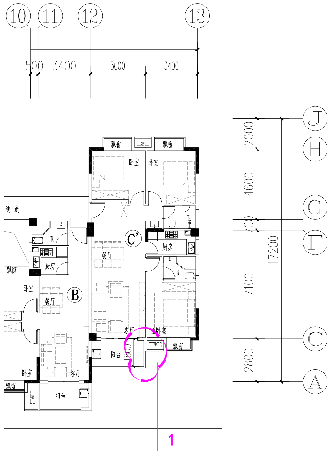
3#楼三~十八层平面图
