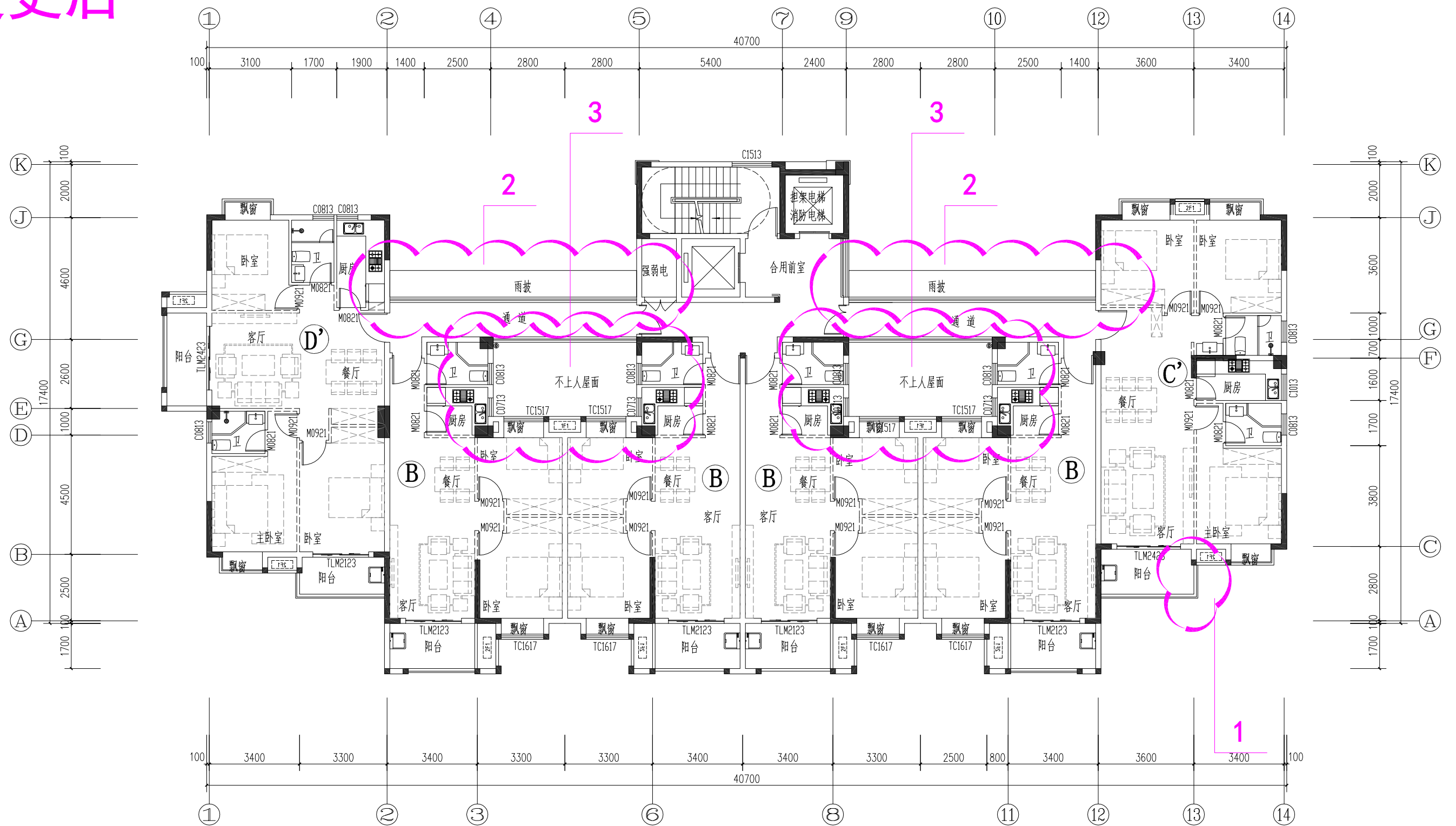
2#楼二层平面图
