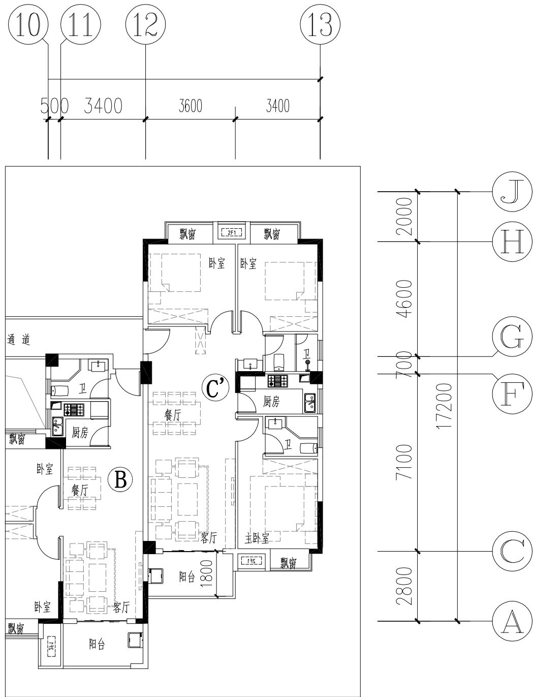
1#楼三~十八层平面图
