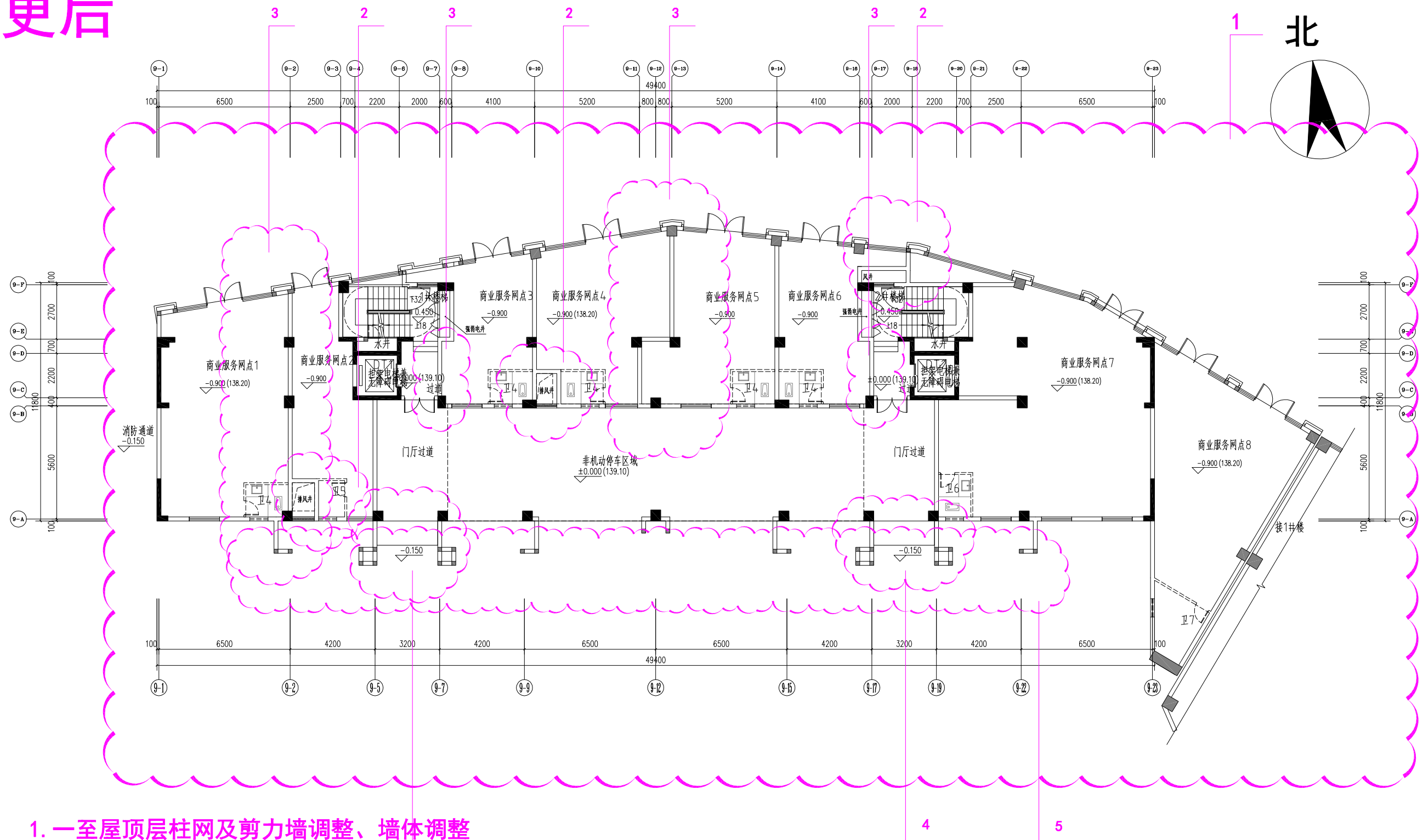
9#楼一层平面图
