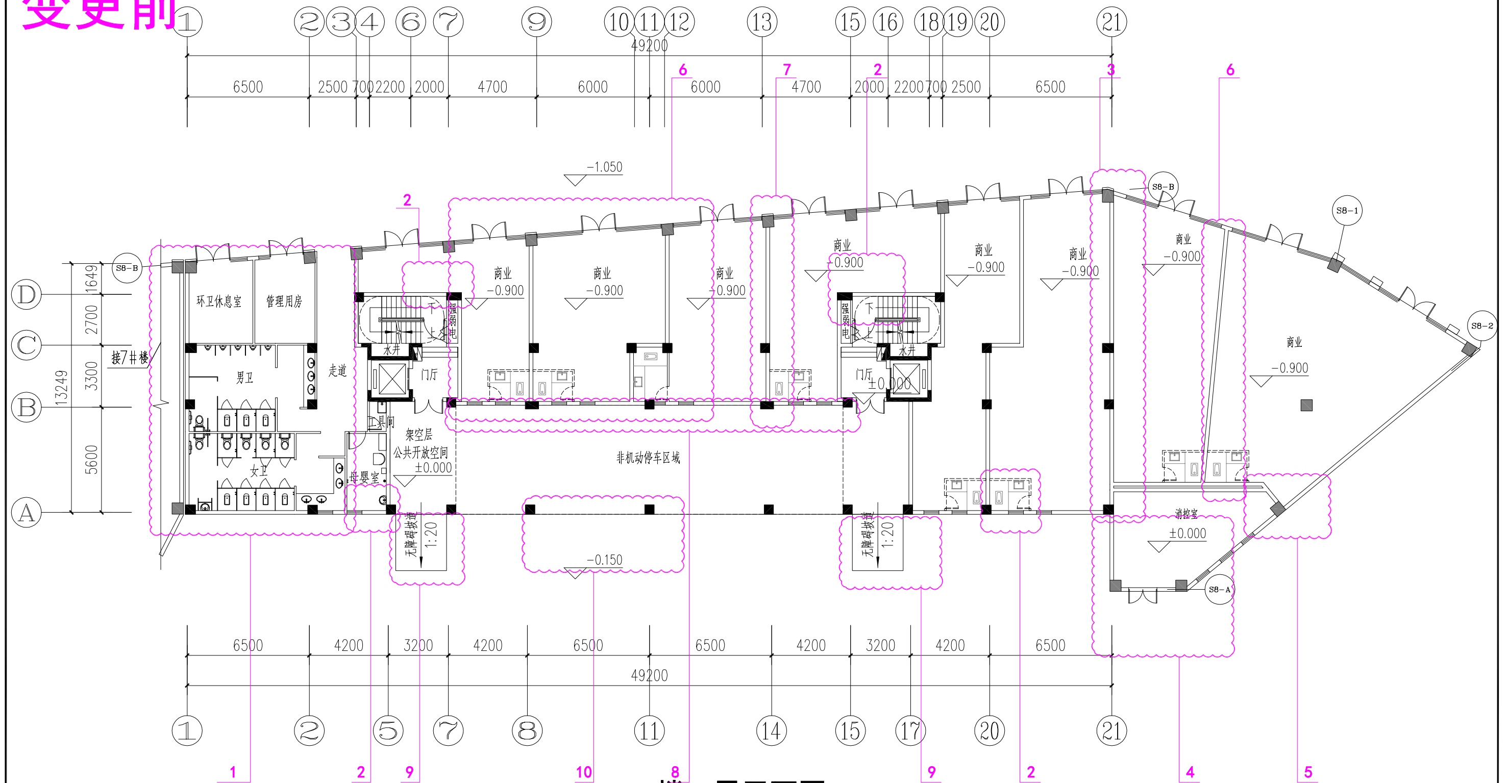
8#楼一层平面图
