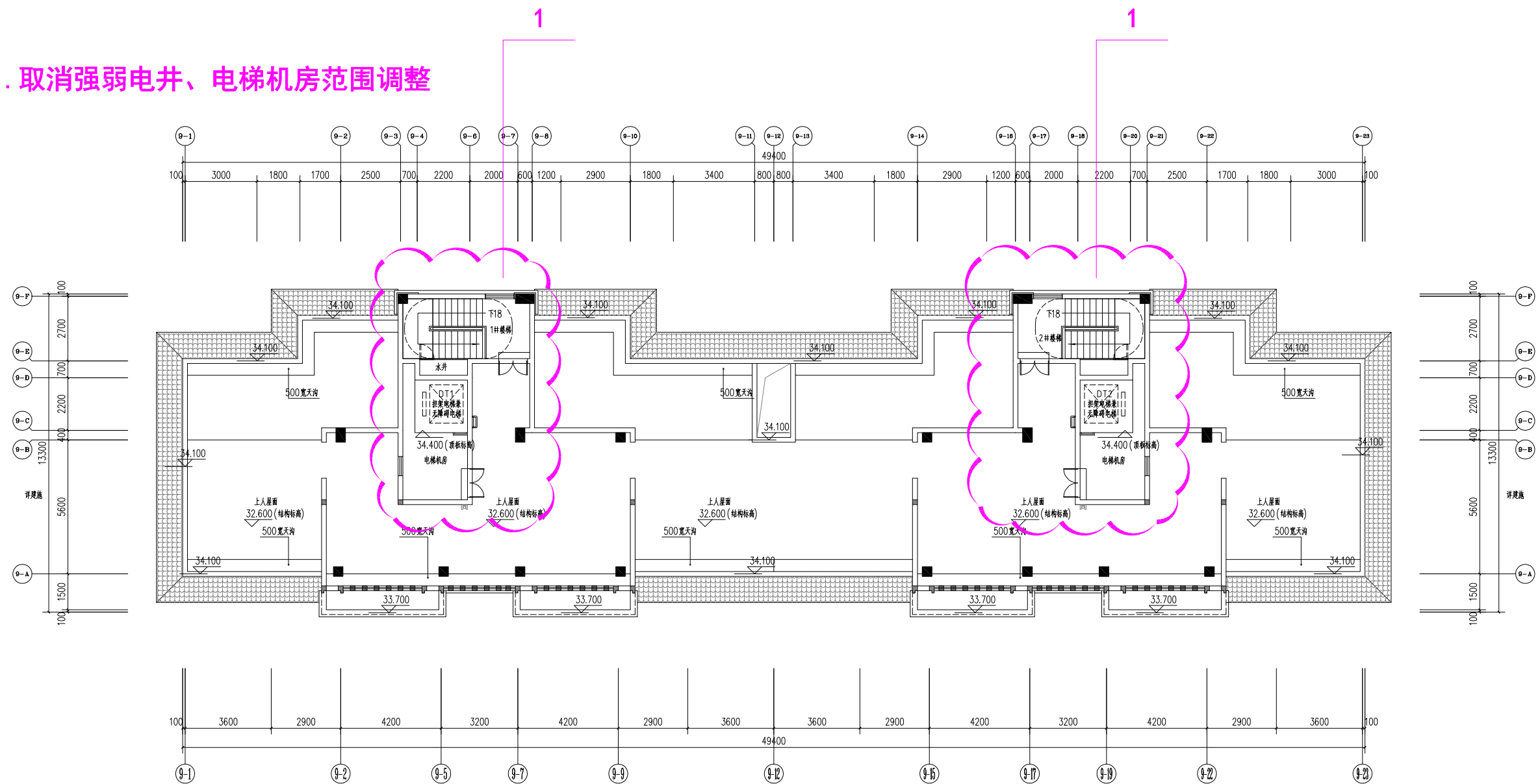
9#楼屋面层平面图
