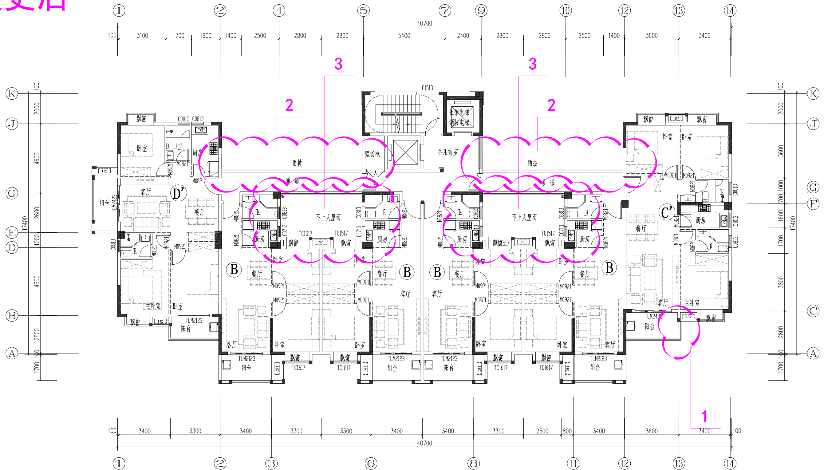
3#楼二层平面图
