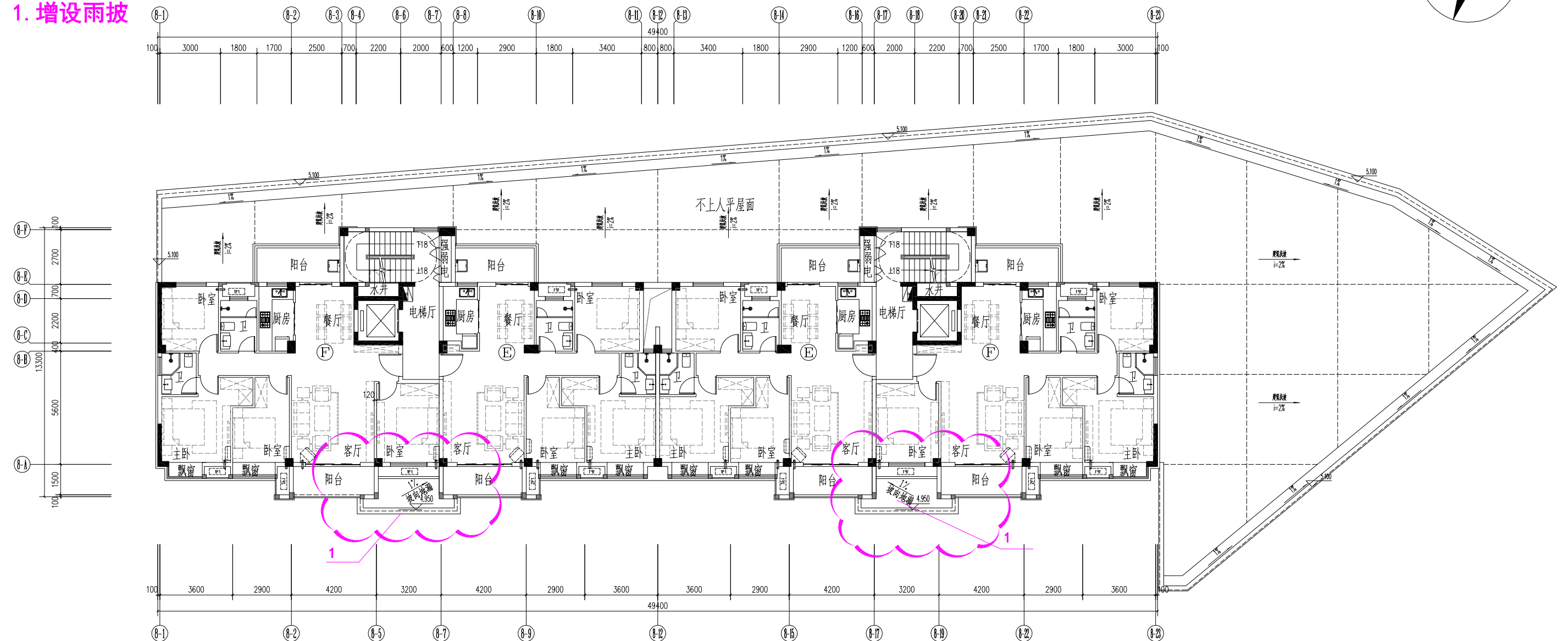
8#楼二层平面图
