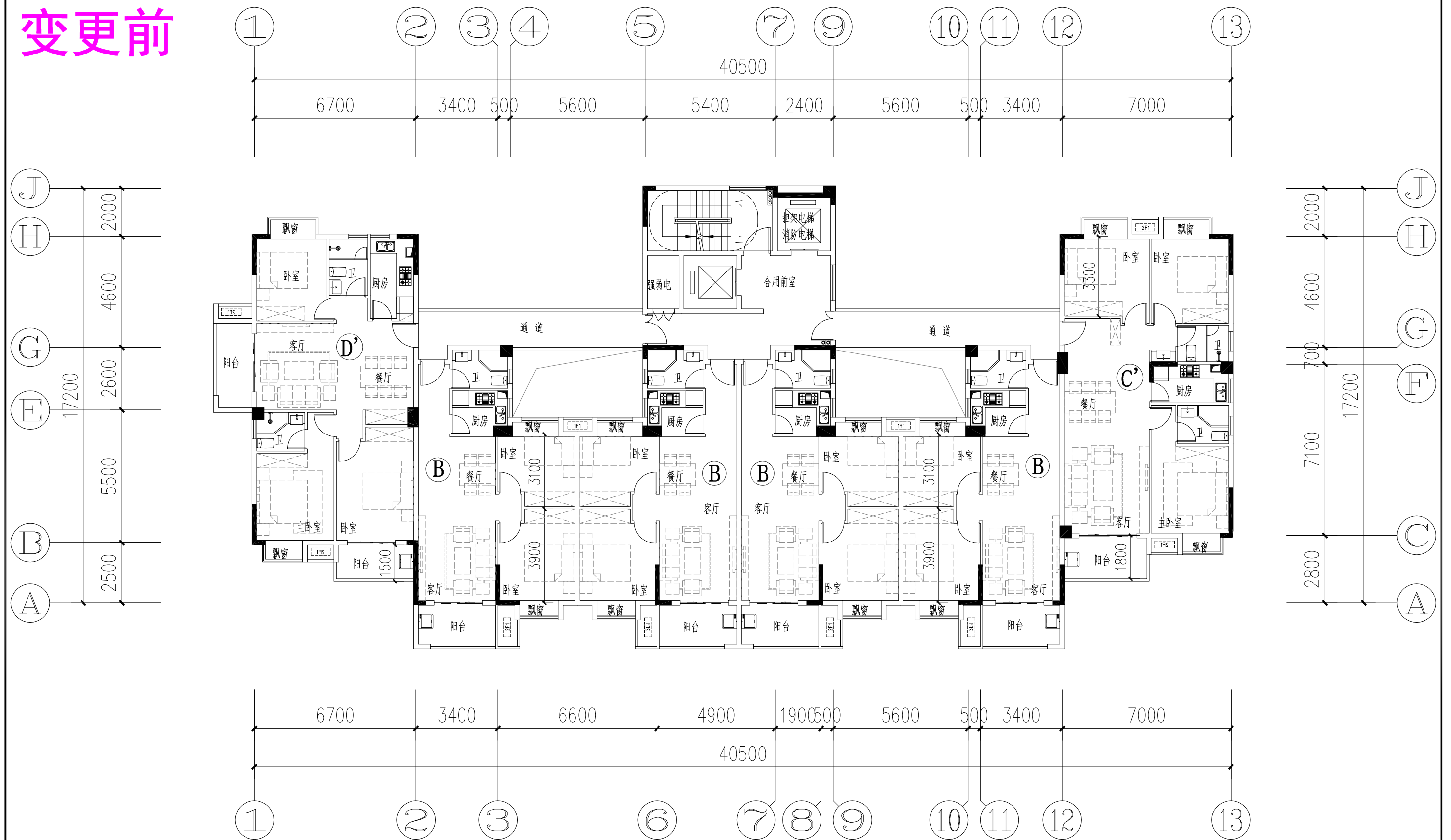
3#楼二~十八层平面图
