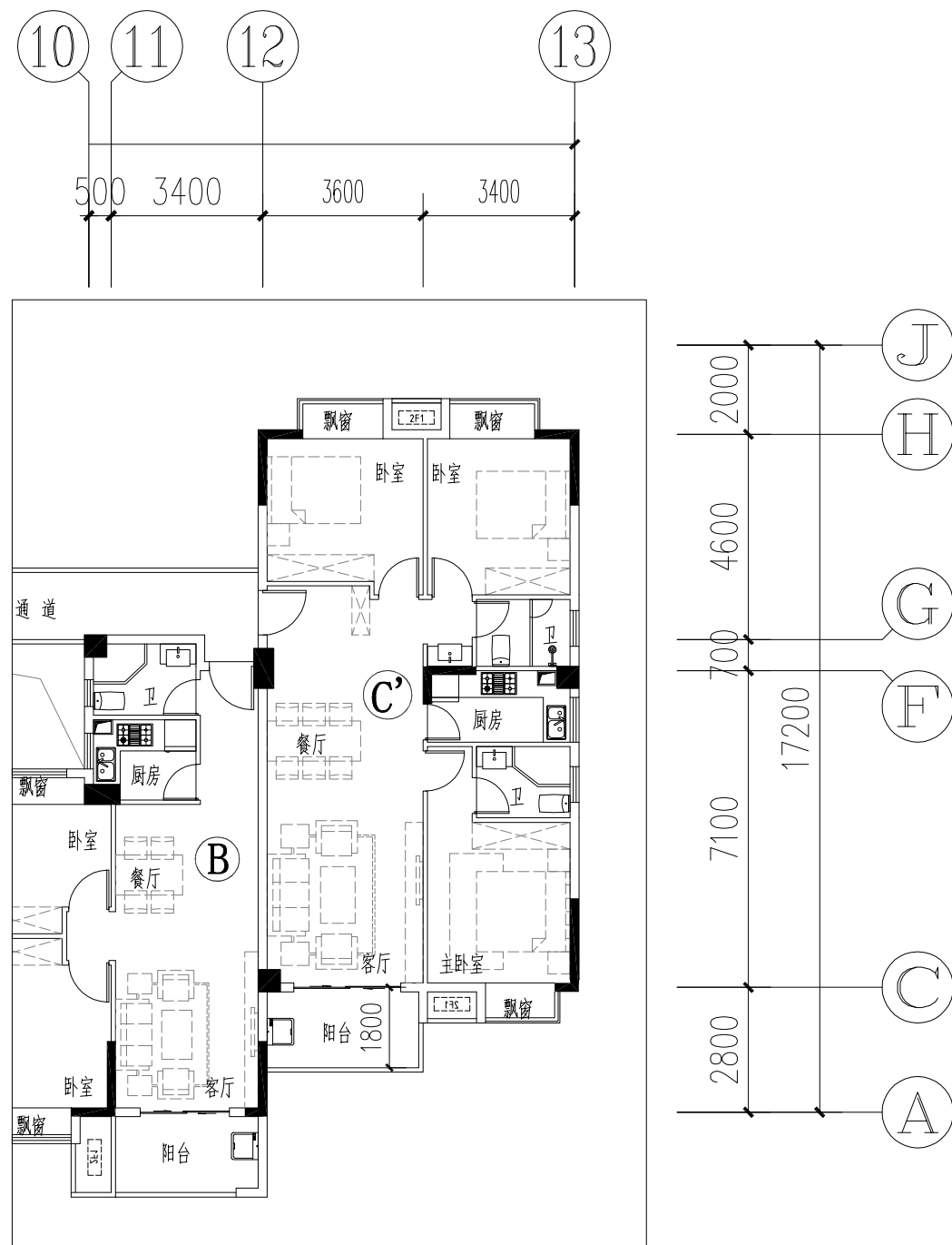
2#楼三~十八层平面图
