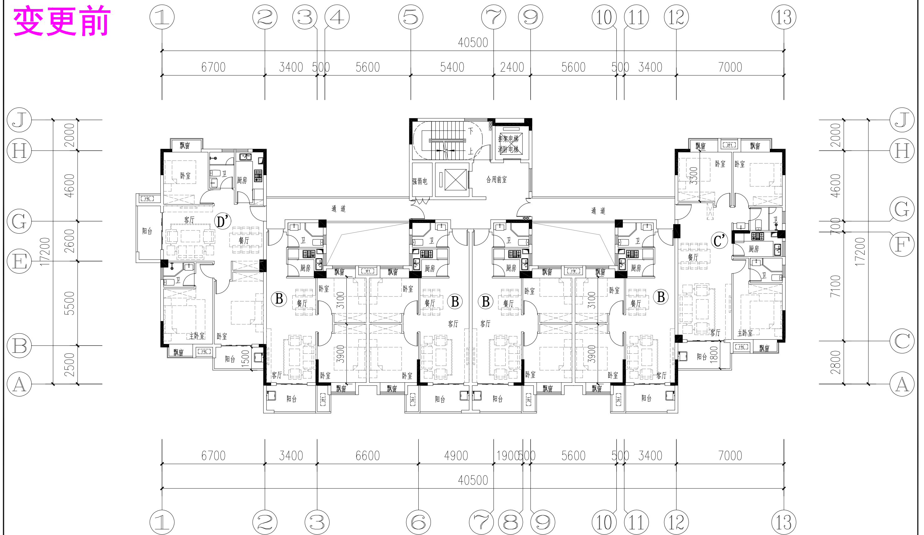
2#楼二~十八层平面图
