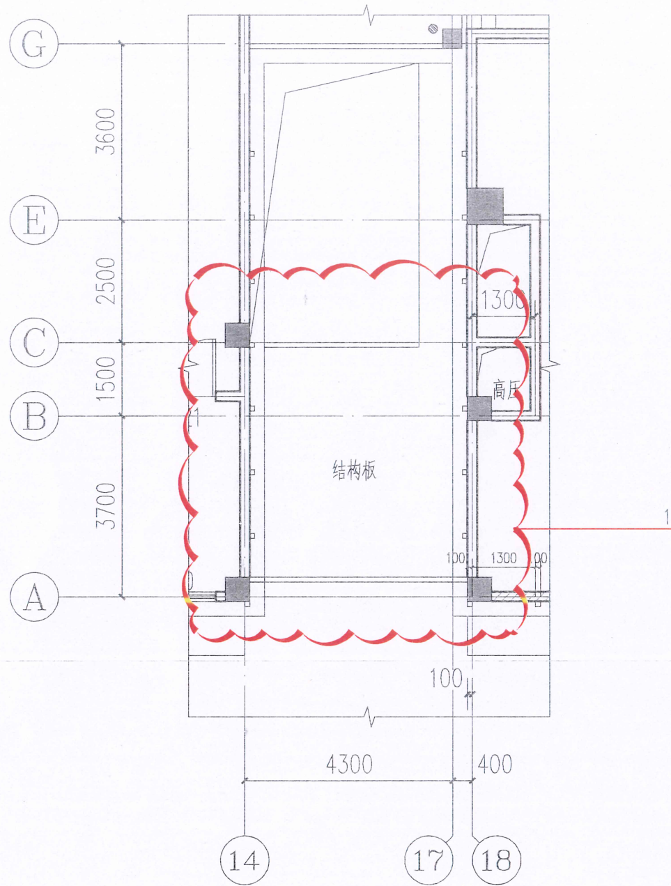
19#楼二层局部平面图 (原审批图)
