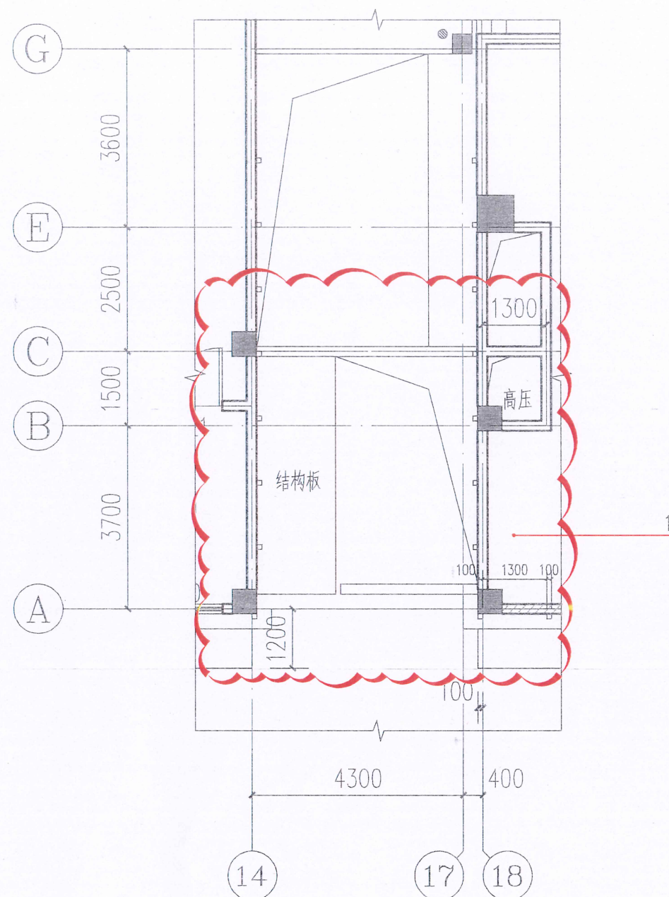
19#楼二层局部平面图 (拟变更图)
