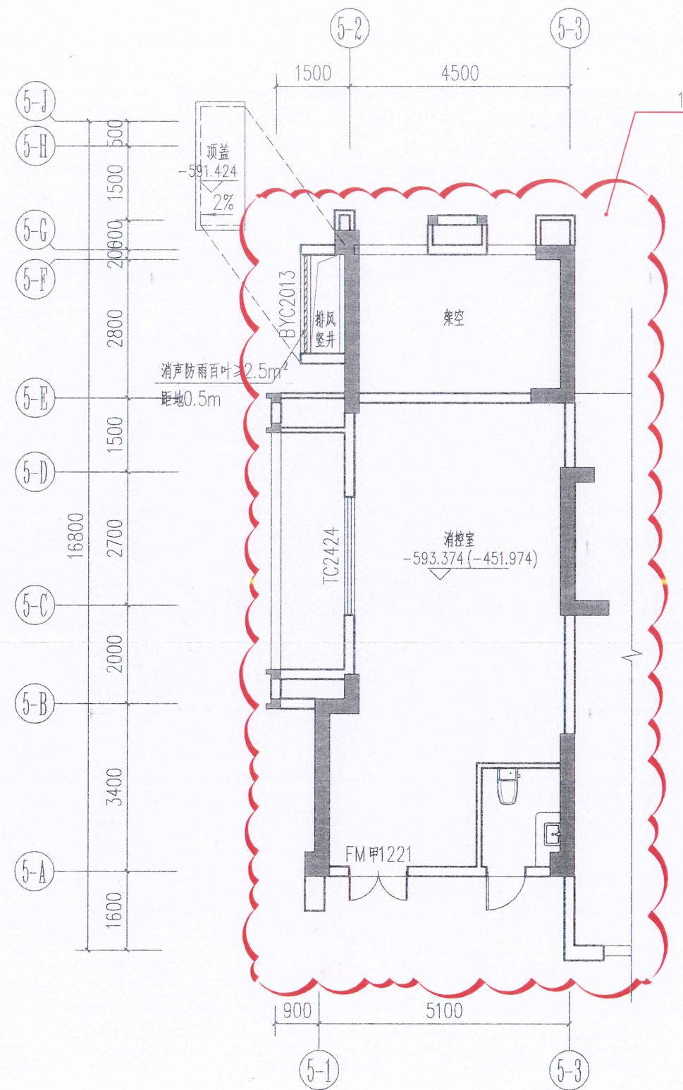
5#一层局部平面图 (原审批图)
