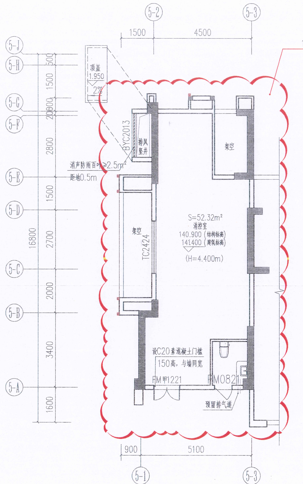
5#一层局部平面图 (拟变更图)
