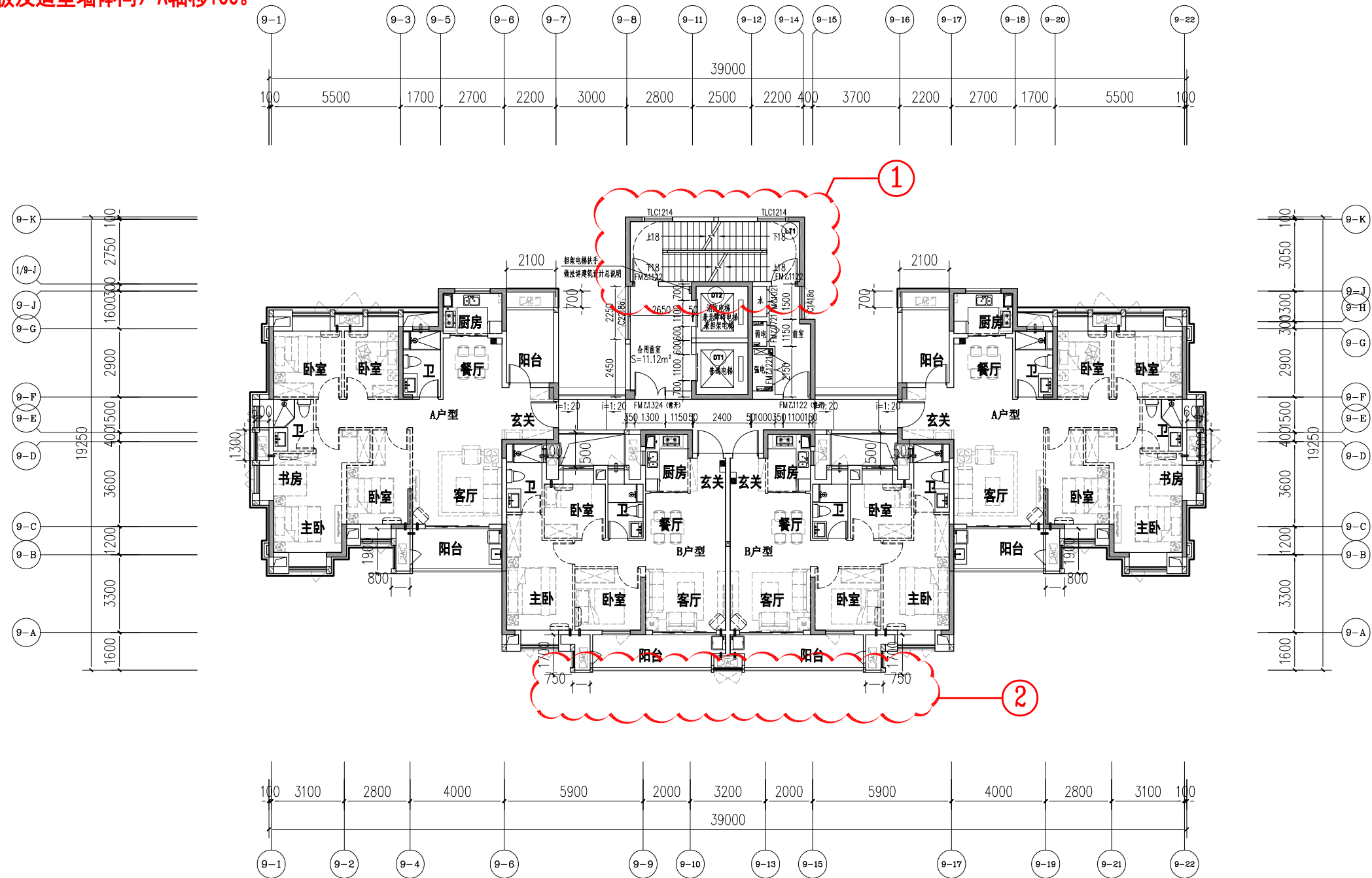
9#楼五至二十三层平面图 1:200
