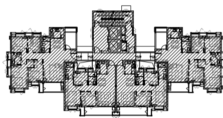
9#结构走向示意图
