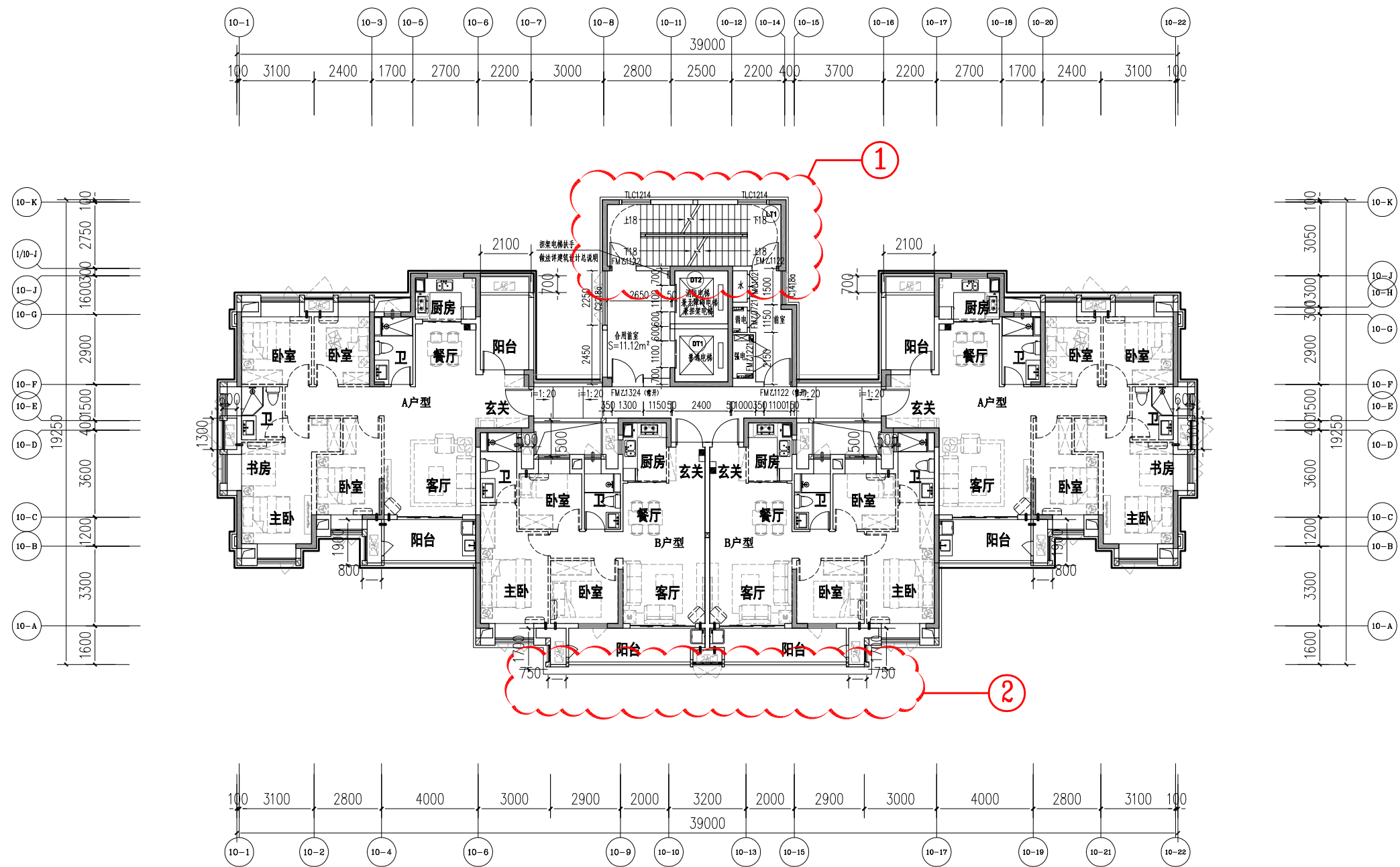
10#楼三、四层平面图 1:200
