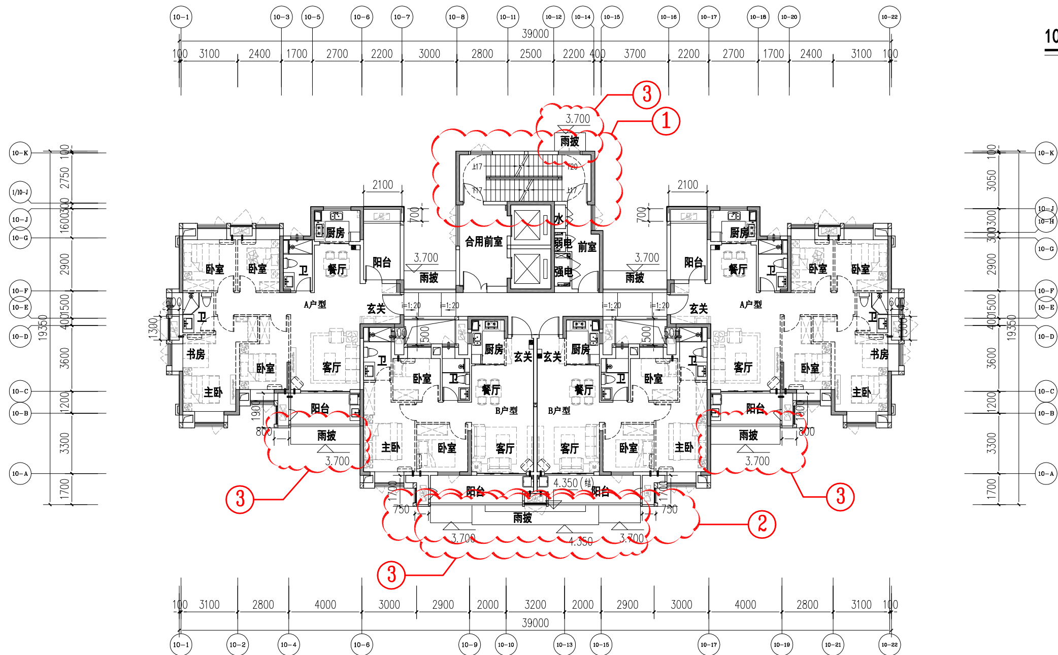
10#楼二层平面图 1:200
