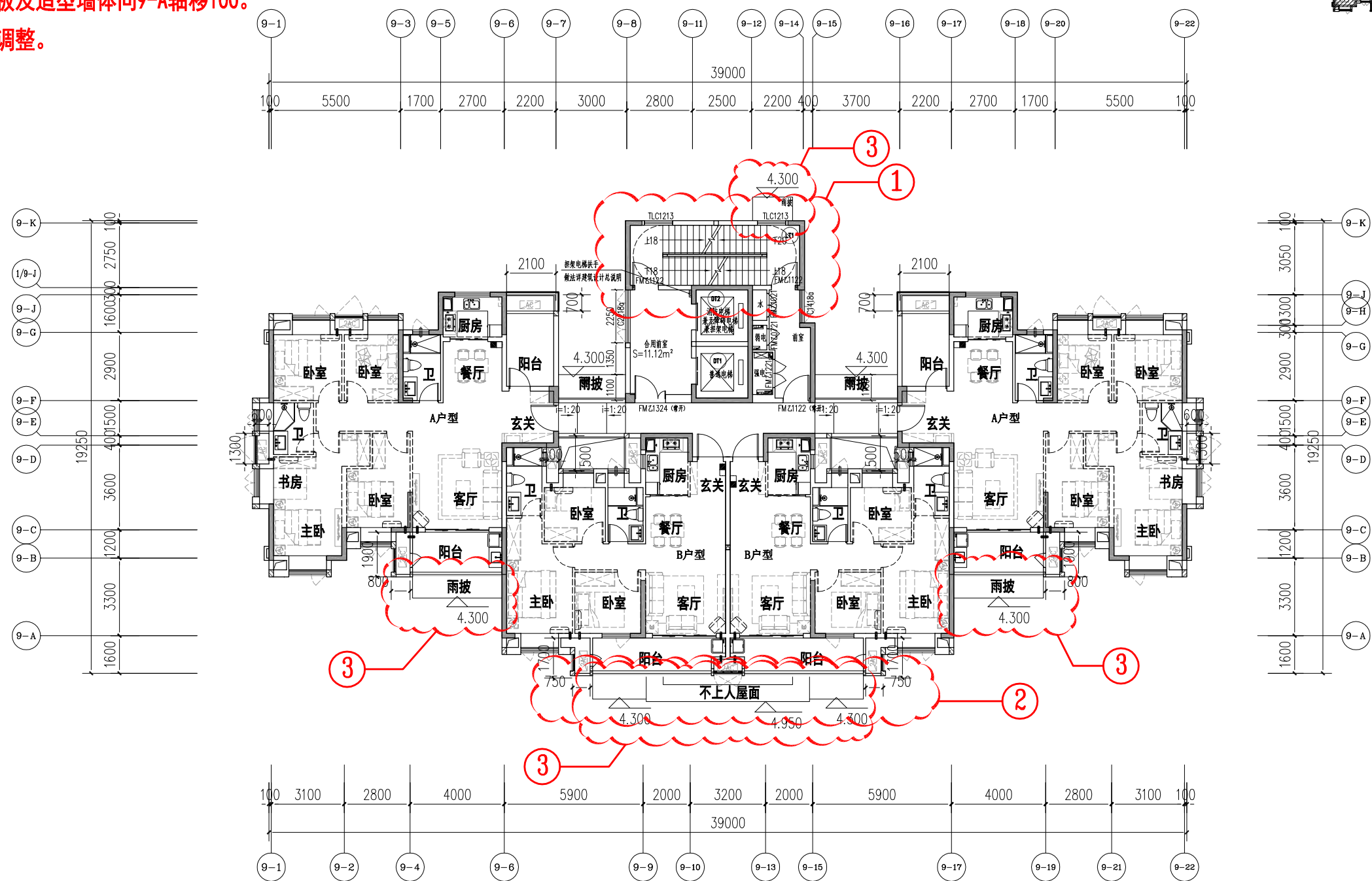
9#结构走向示意图
