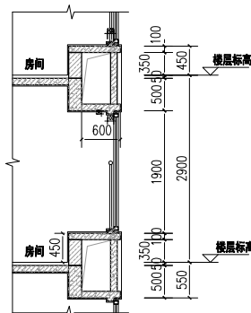
凸窗大样
