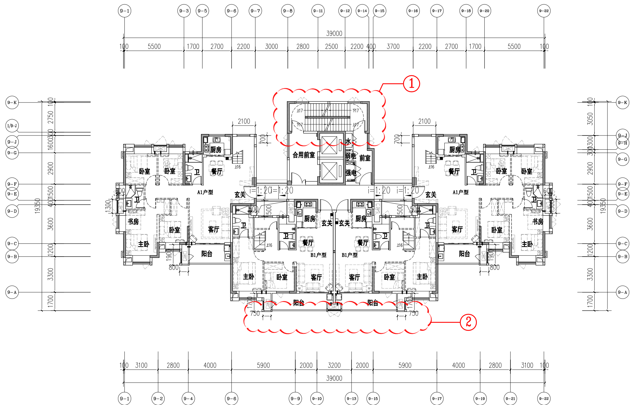
9#楼二十四层平面图 1:200 67.400
