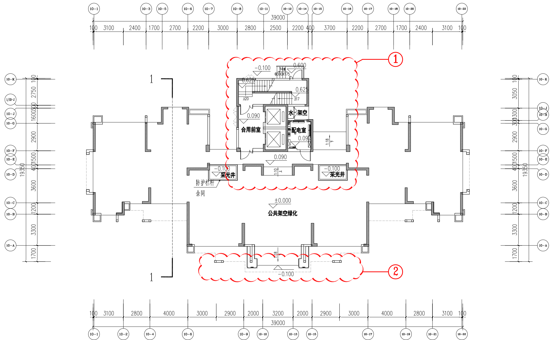
10#楼一层平面图 1:200 ±0.000 (158.00)
