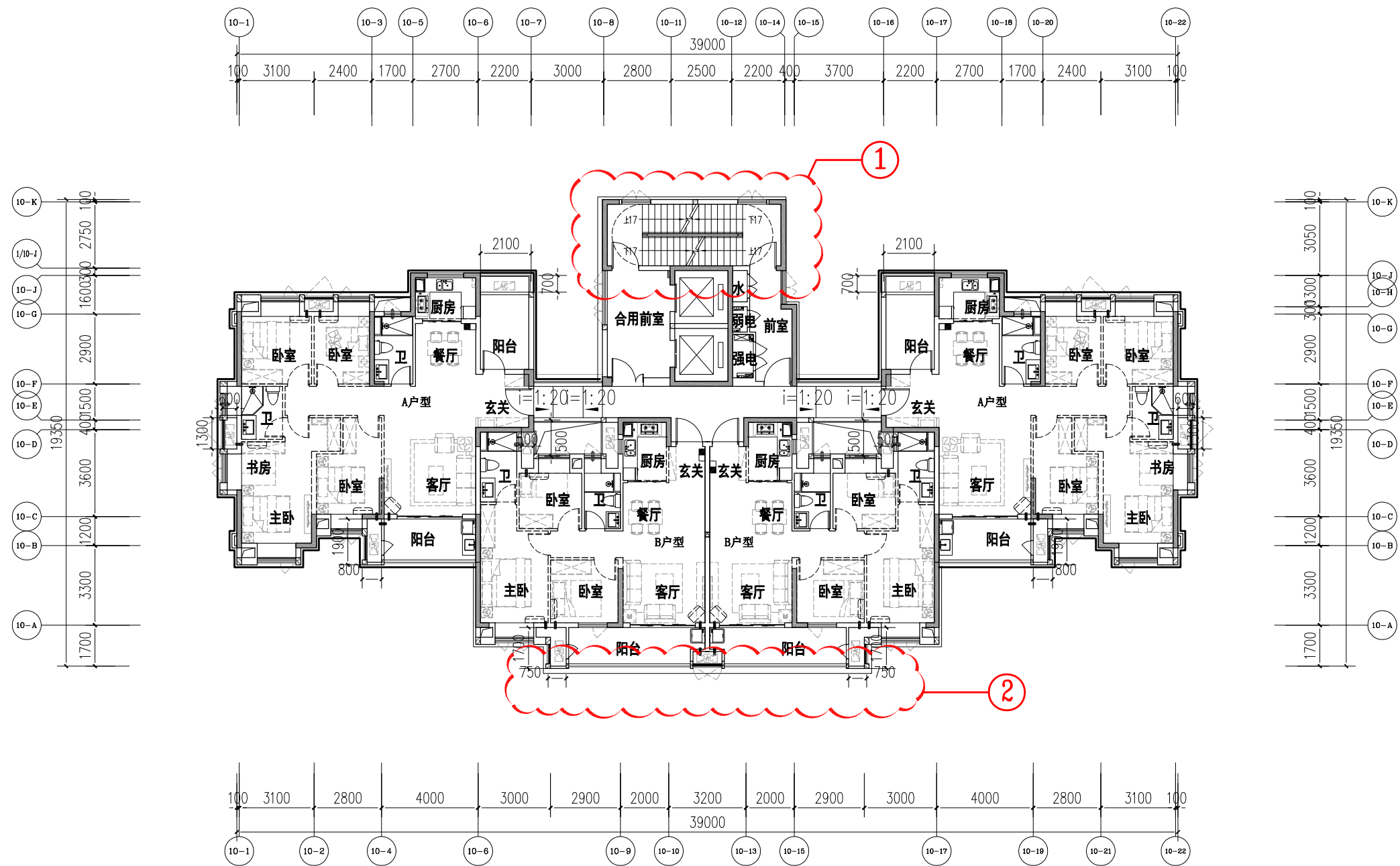
10#楼三、四层平面图 1:200 (9.400) 4F 6.500 3F
