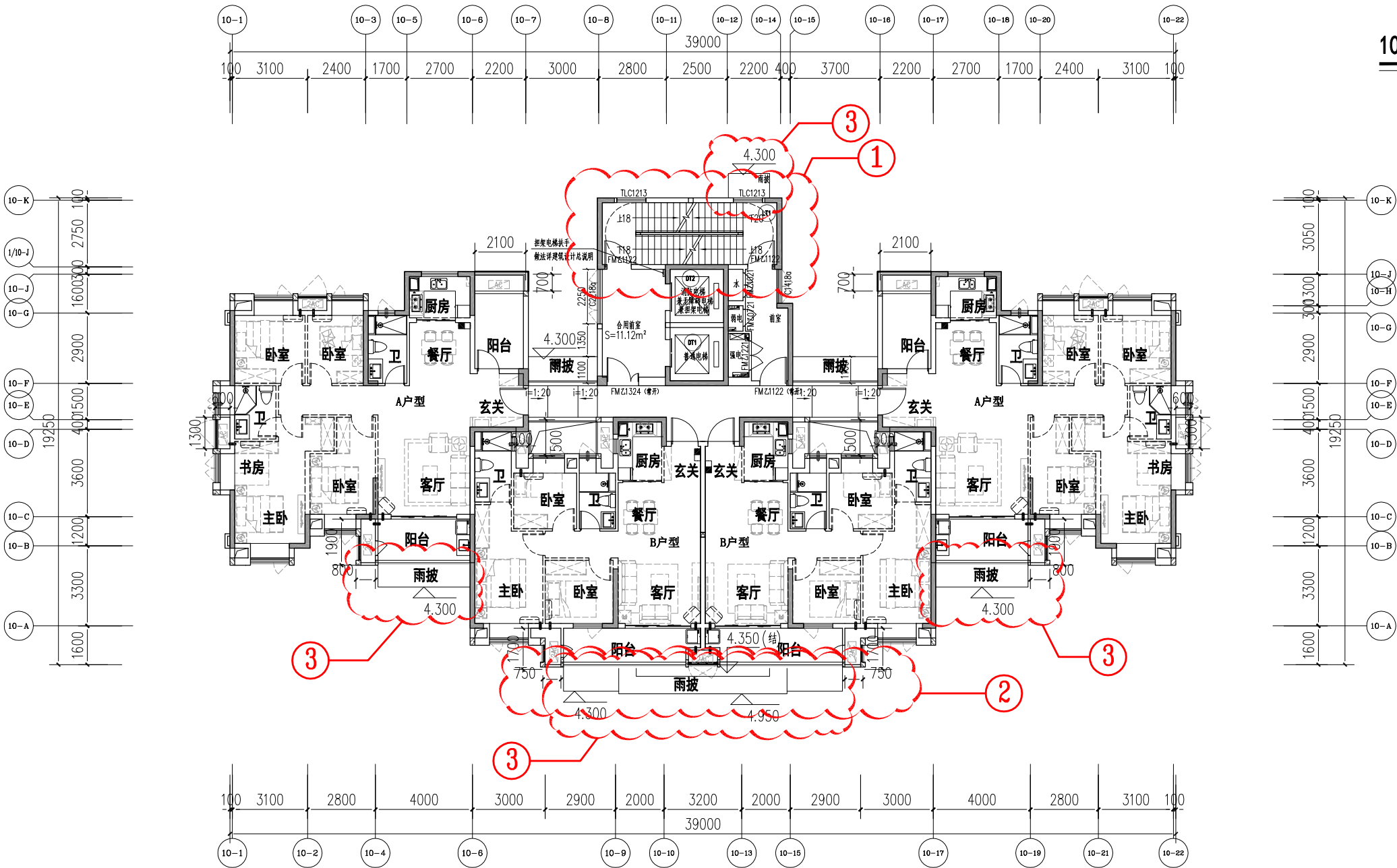
10#楼二层平面图 1:200
