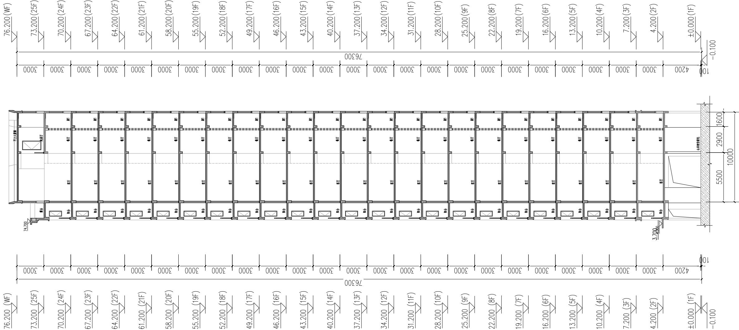
10#楼1-1剖面图 1:200
