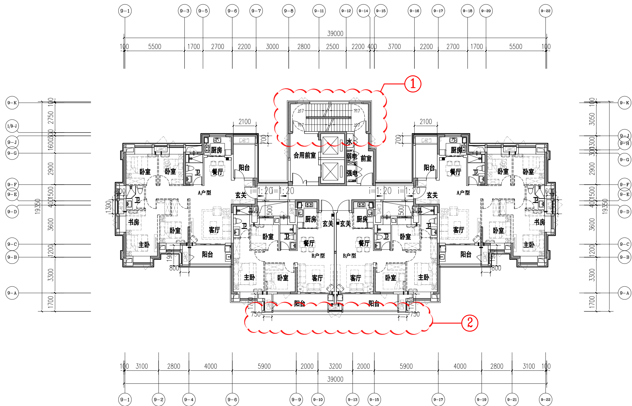
9#楼三、四层平面图 1:200
