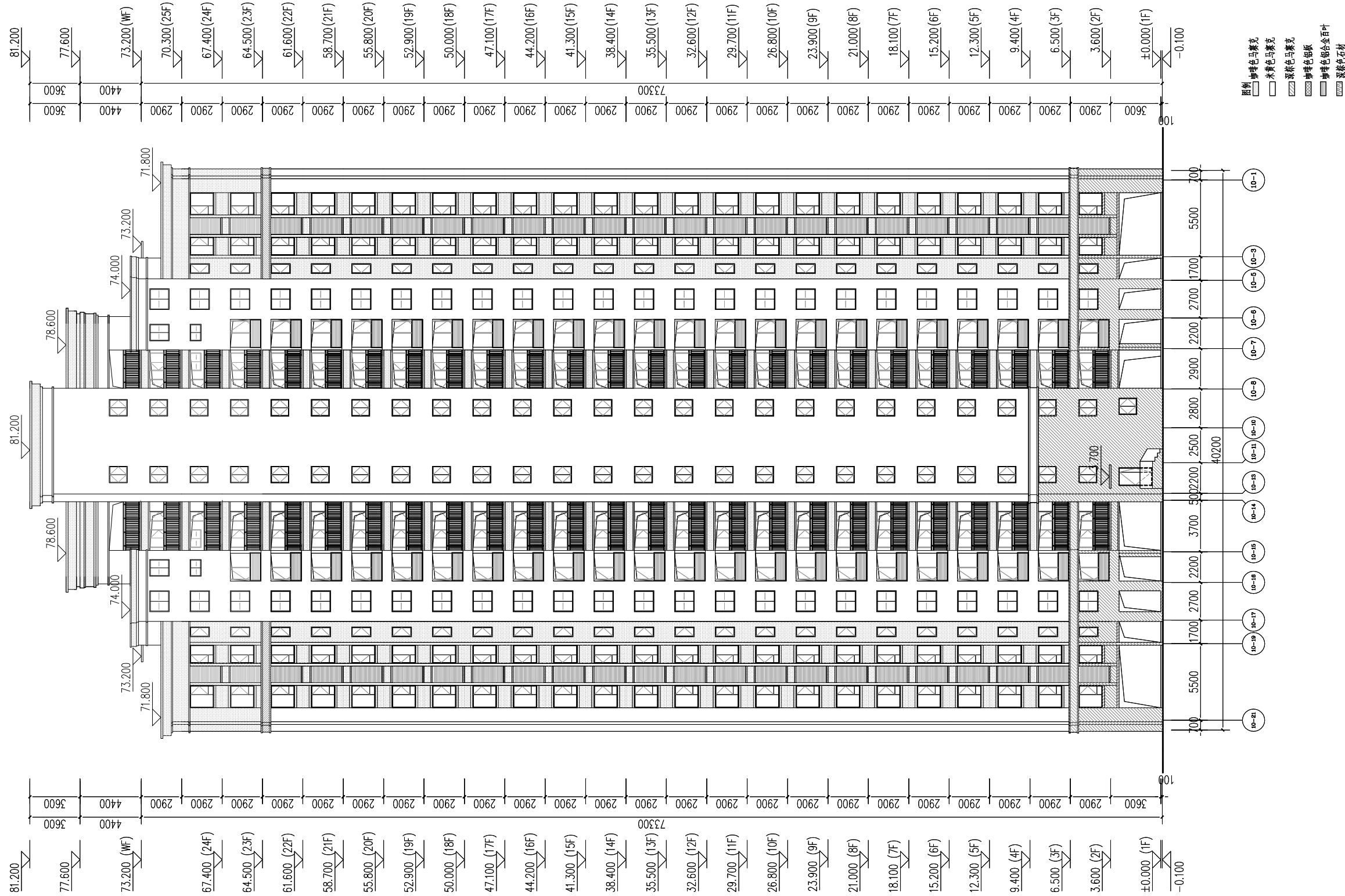
10-1 轴立面图 1:300
