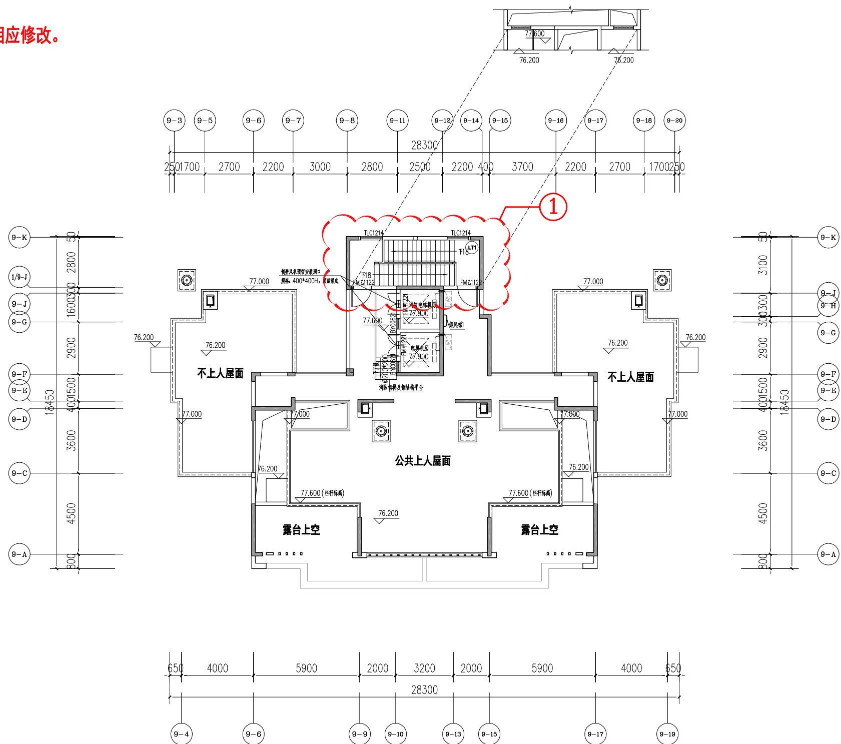
9#楼屋面层平面图 1:200
