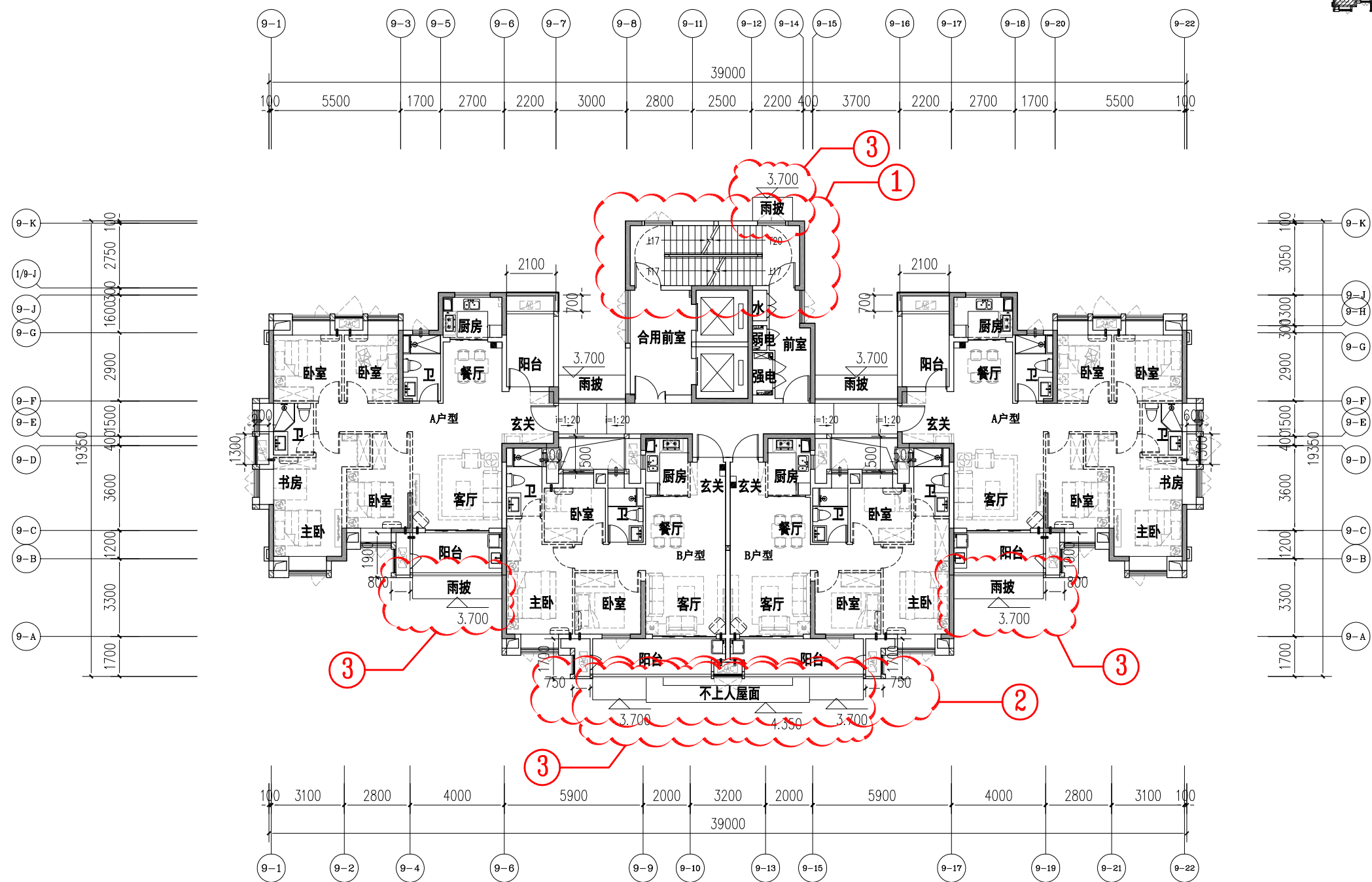
9#楼结构走向示意图
