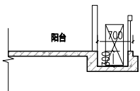
设备平台降板大样
