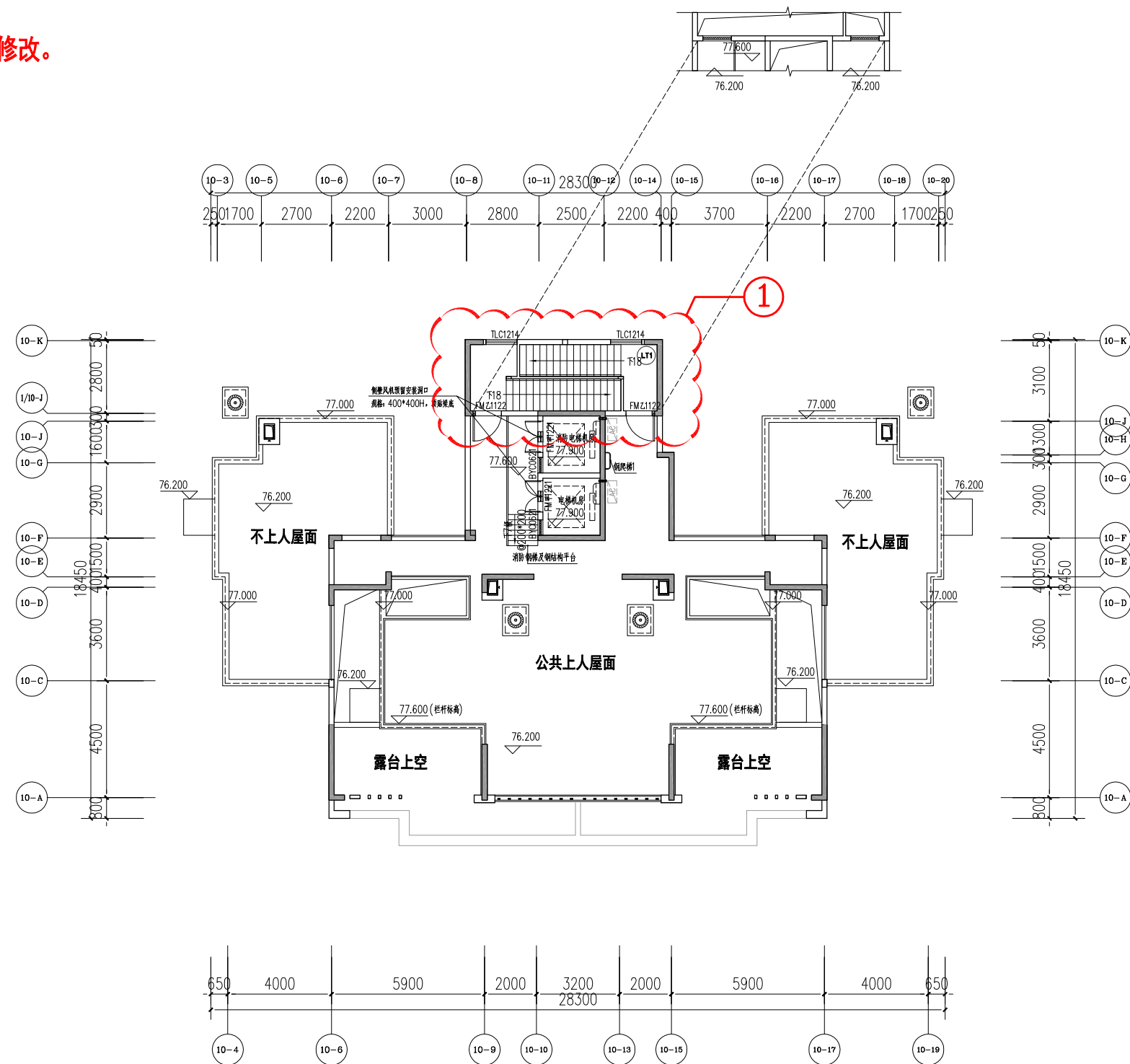
10#楼屋面层平面图 1:200
