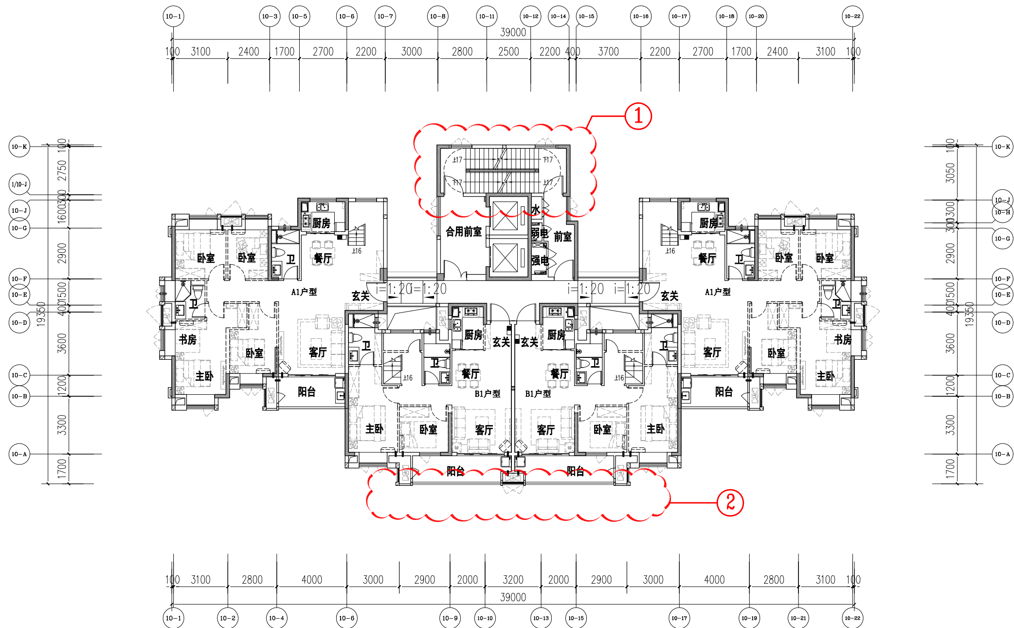
10#楼二十四层平面图 1:200 67.400
