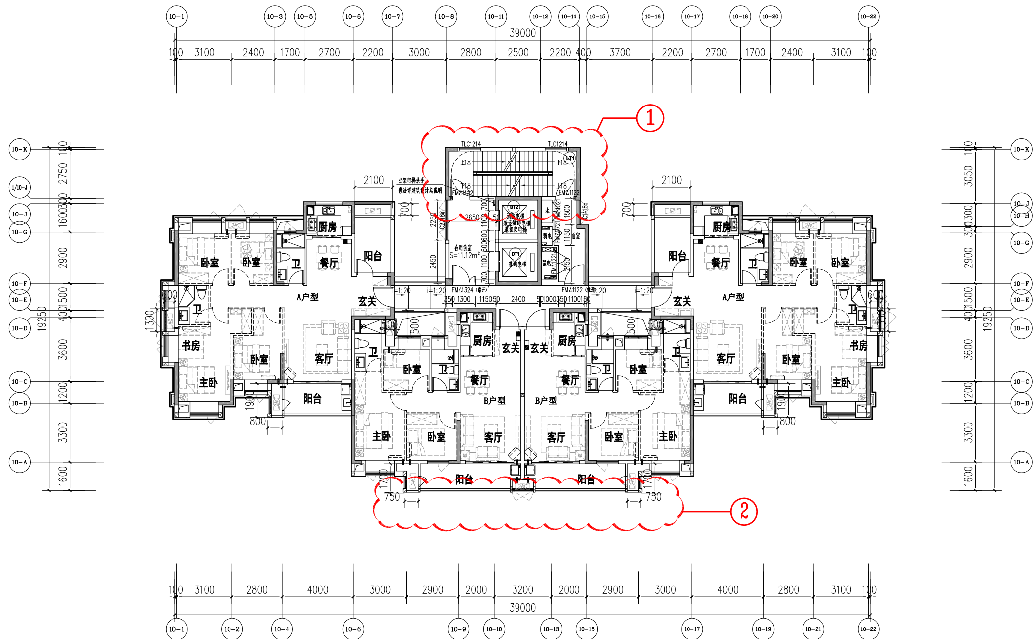
10#楼五至二十三层平面图 1:200
