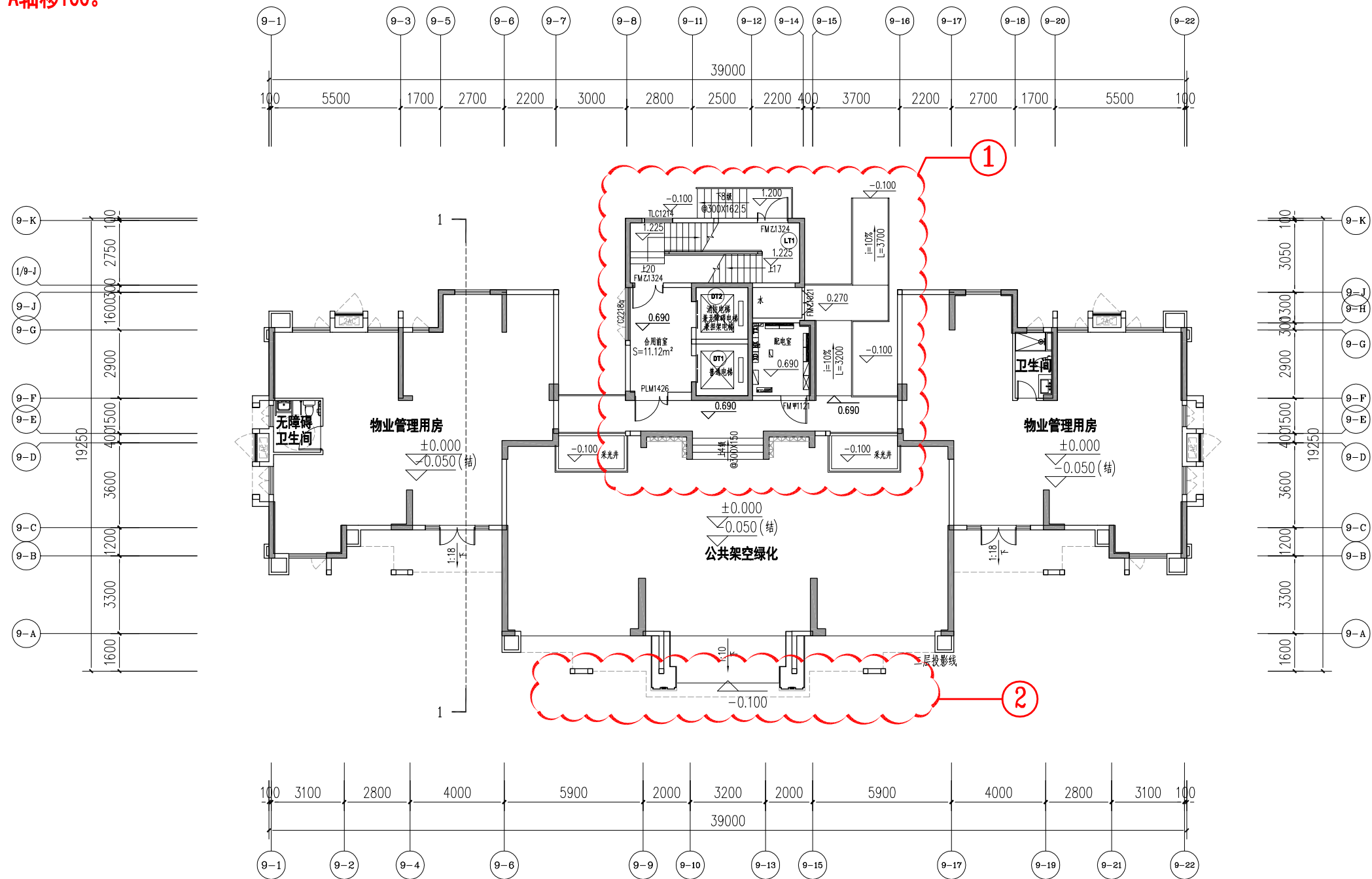
9#楼一层平面图 1:200
