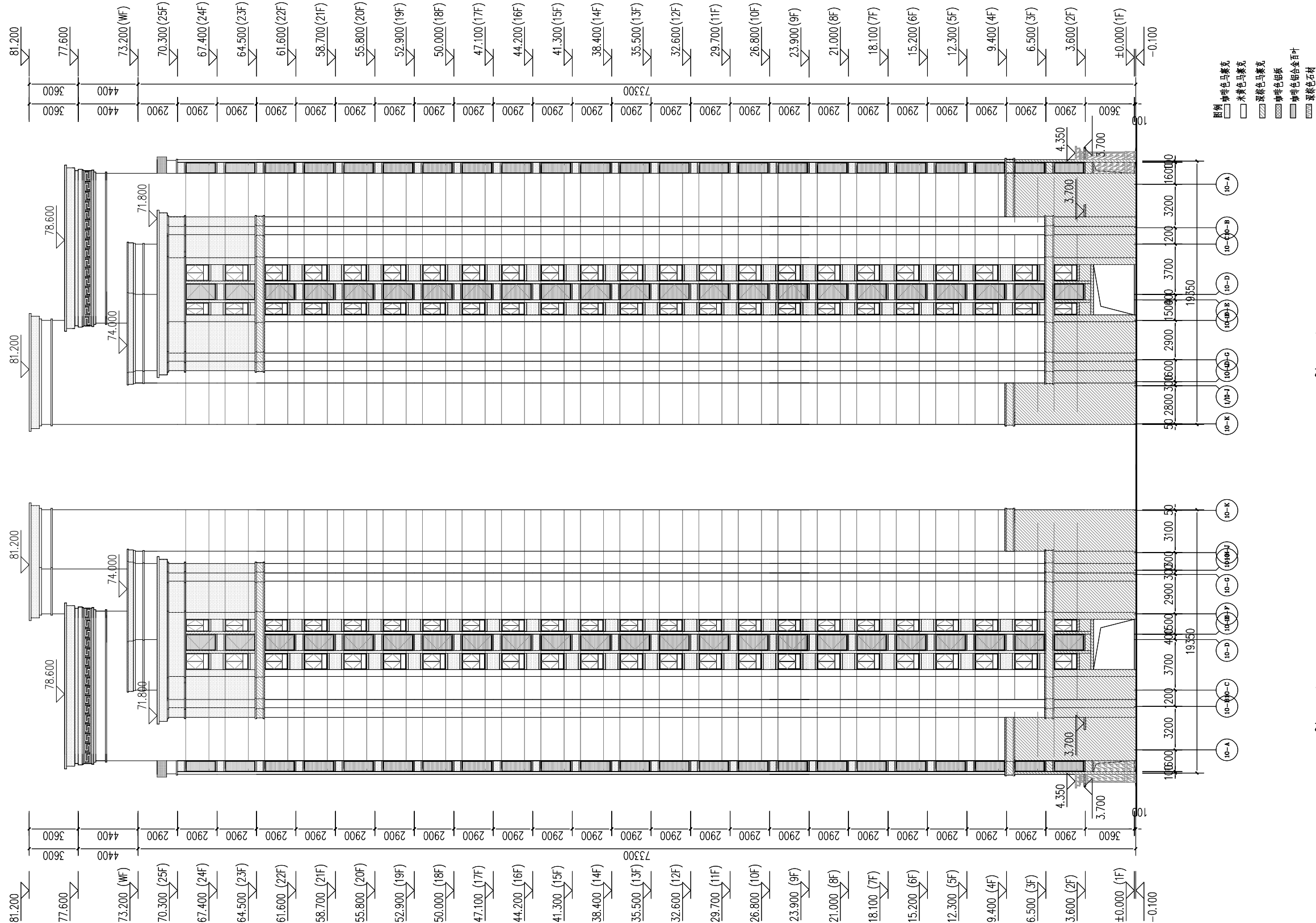
10#楼立面图 1:300
