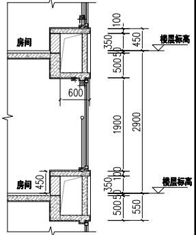
凸窗大样
