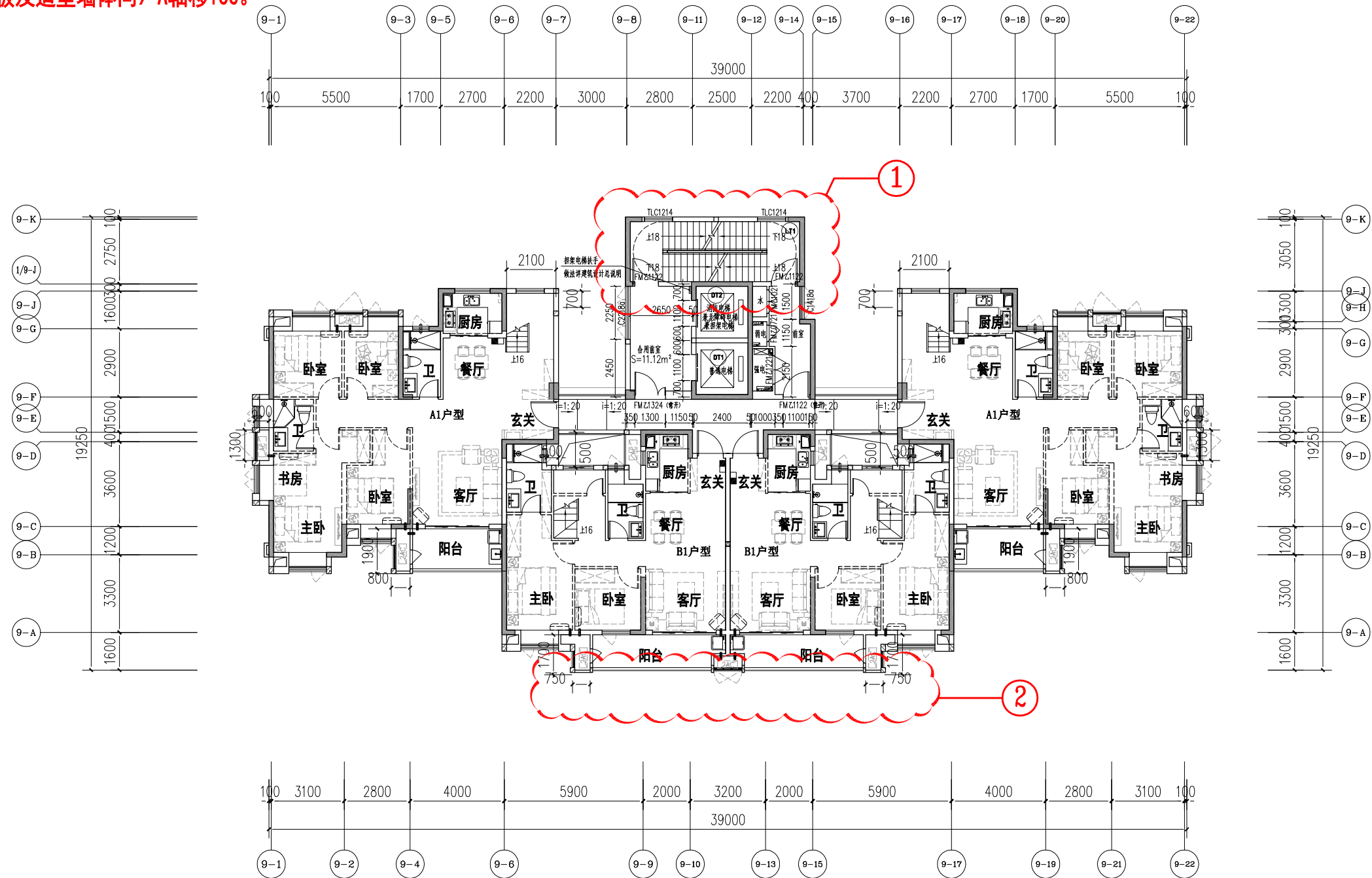
9#楼二十四层平面图 1:200
