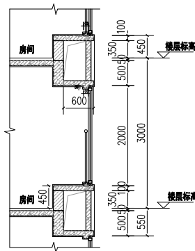
凸窗大样
