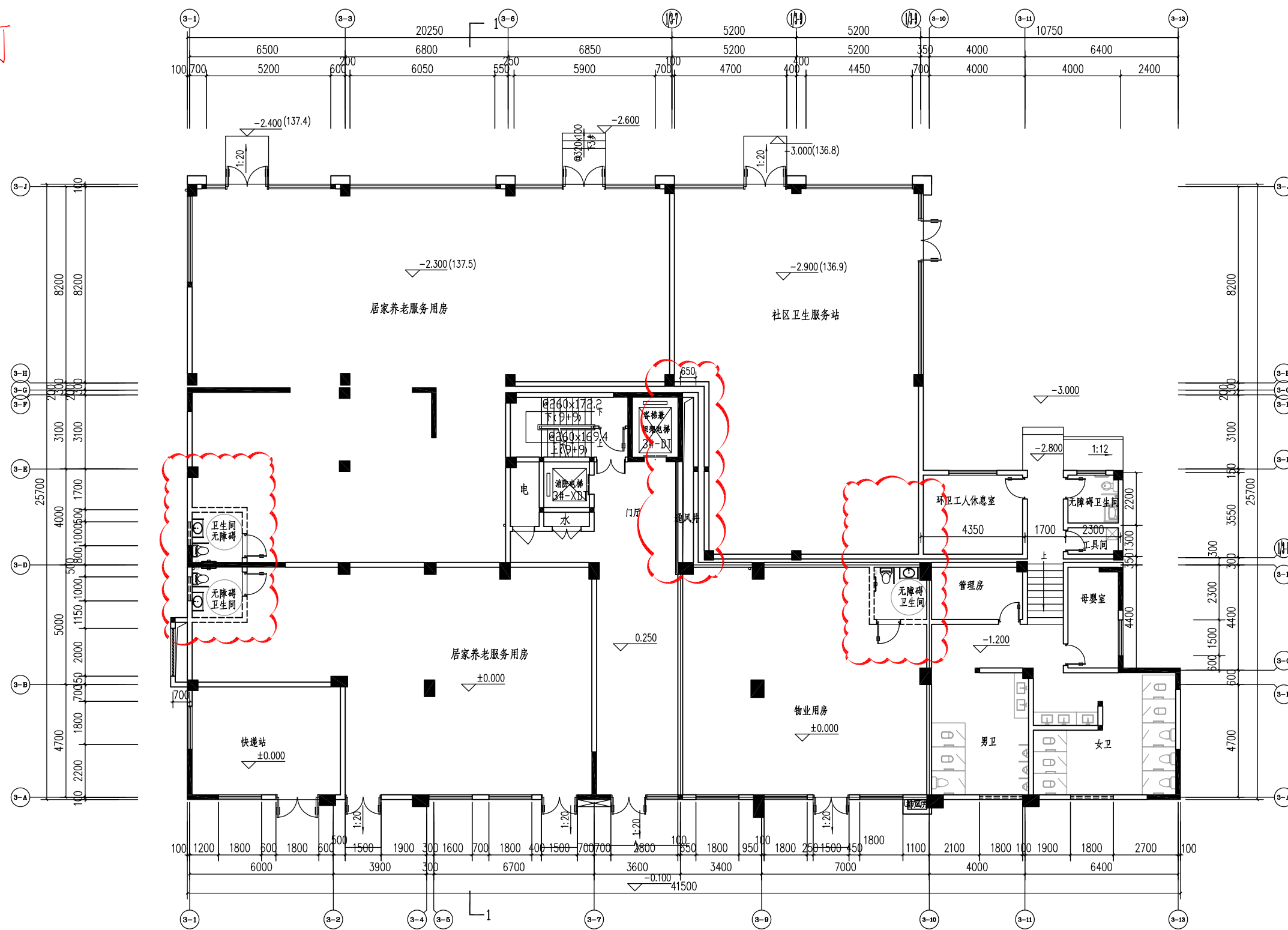
3#楼一层平面图
