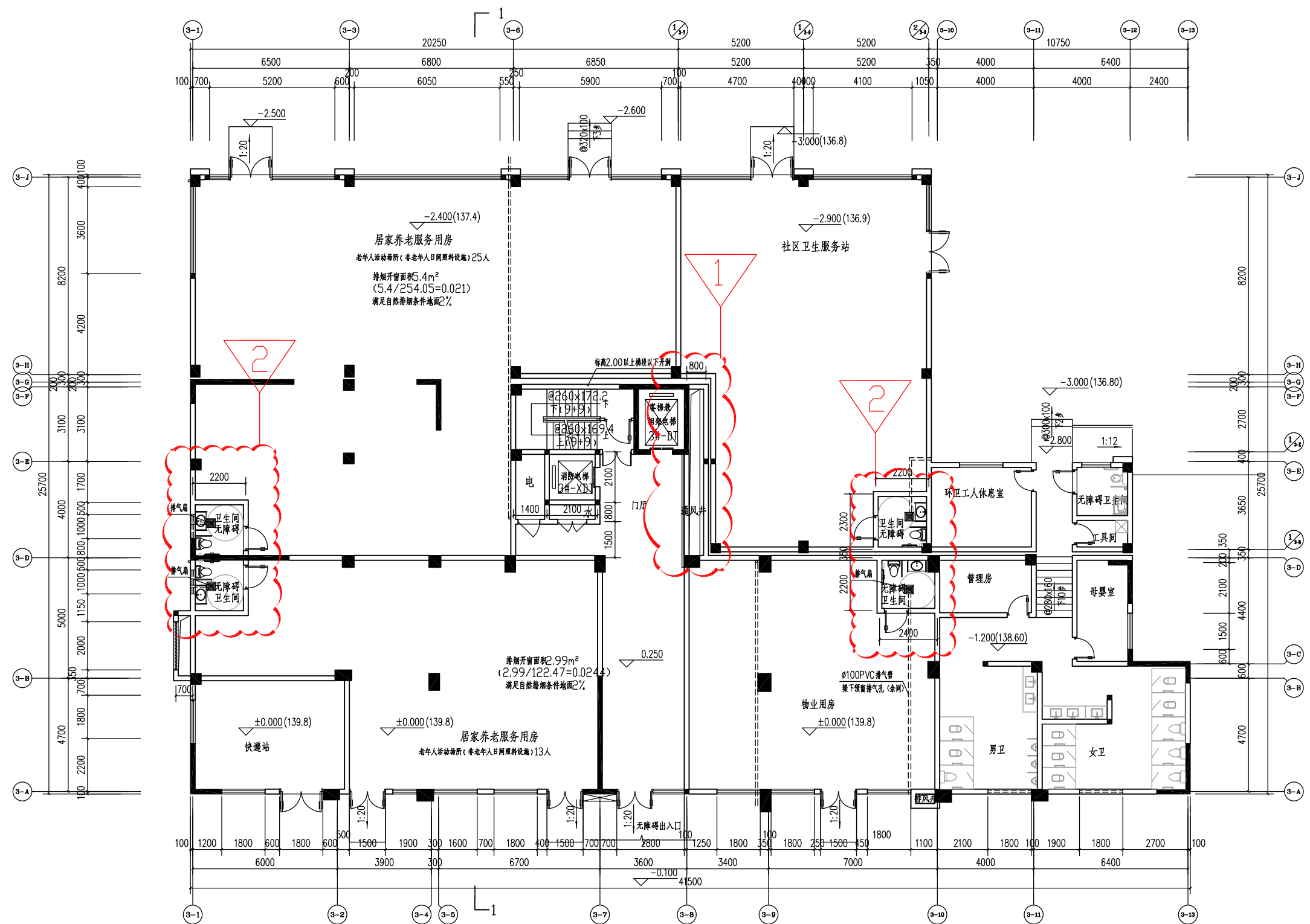
3#楼一层平面图
