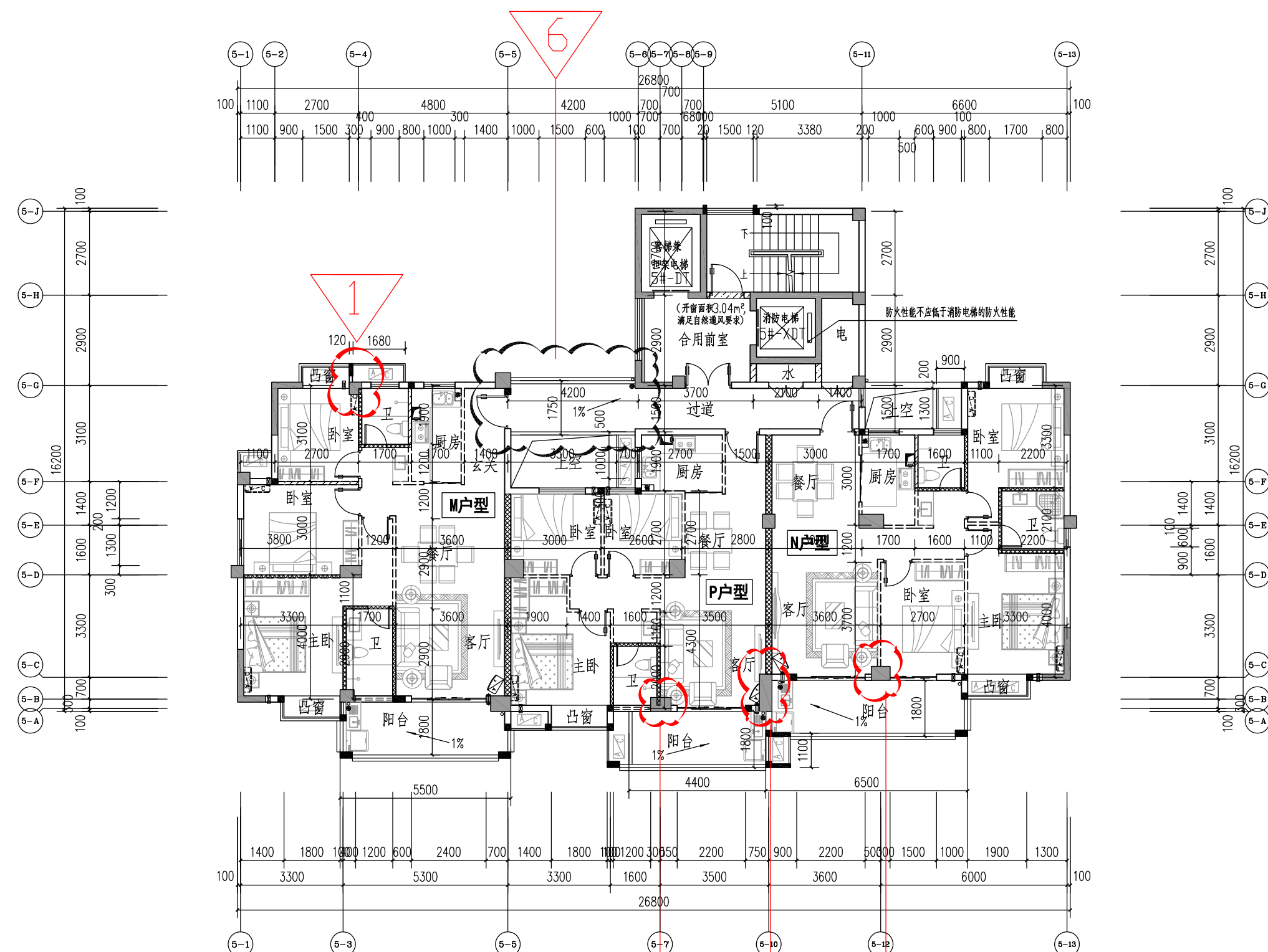
三~十八层平面图 1:100
