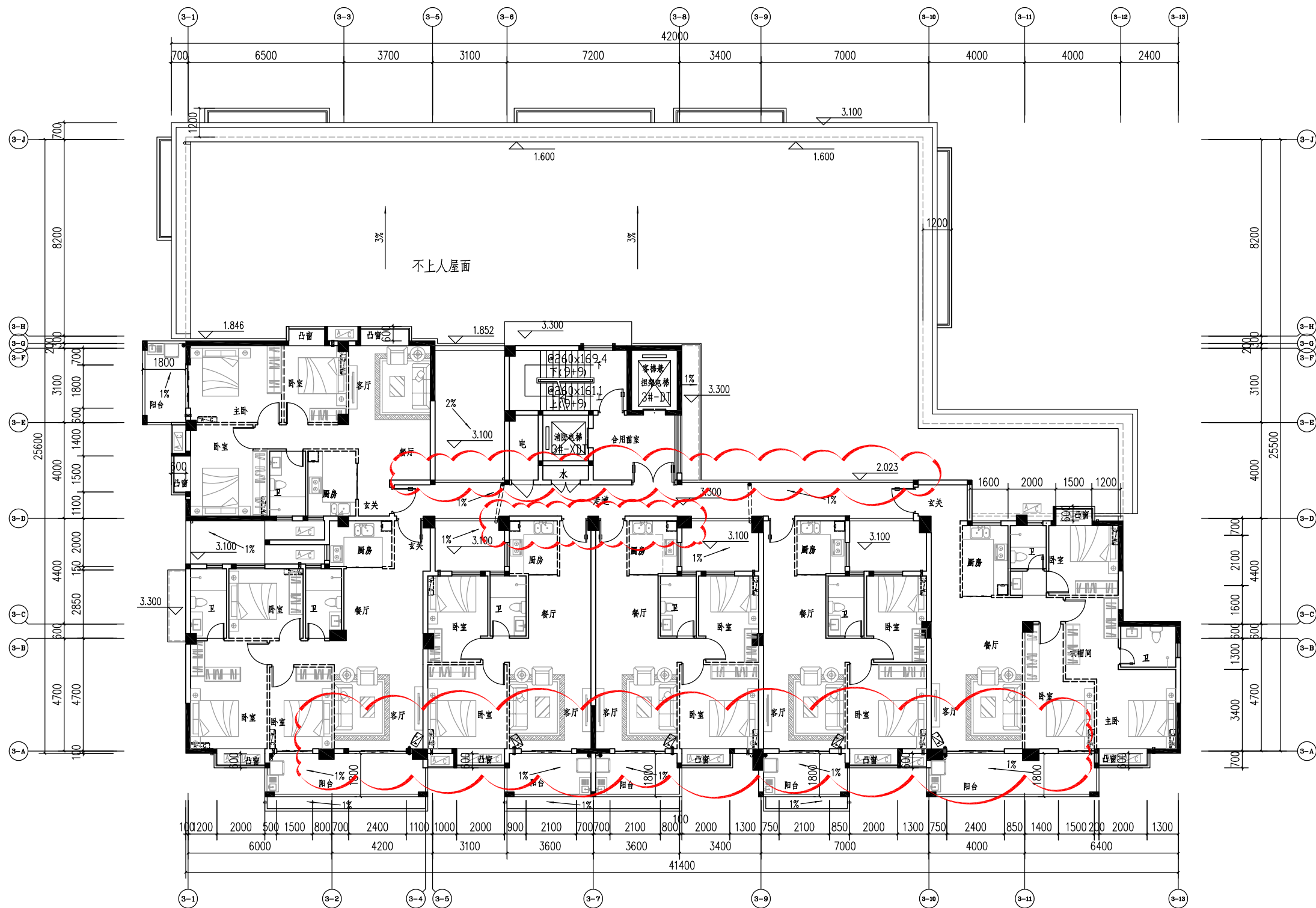
3#楼二层平面图
