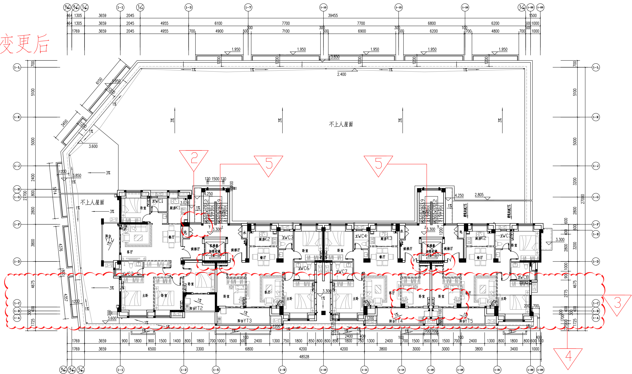
1#楼二层平面图
