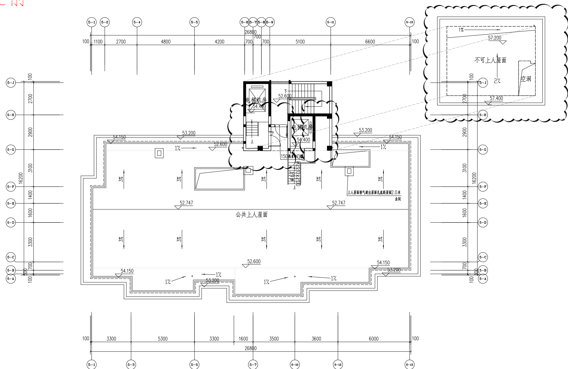
5#楼 屋面层平面图
