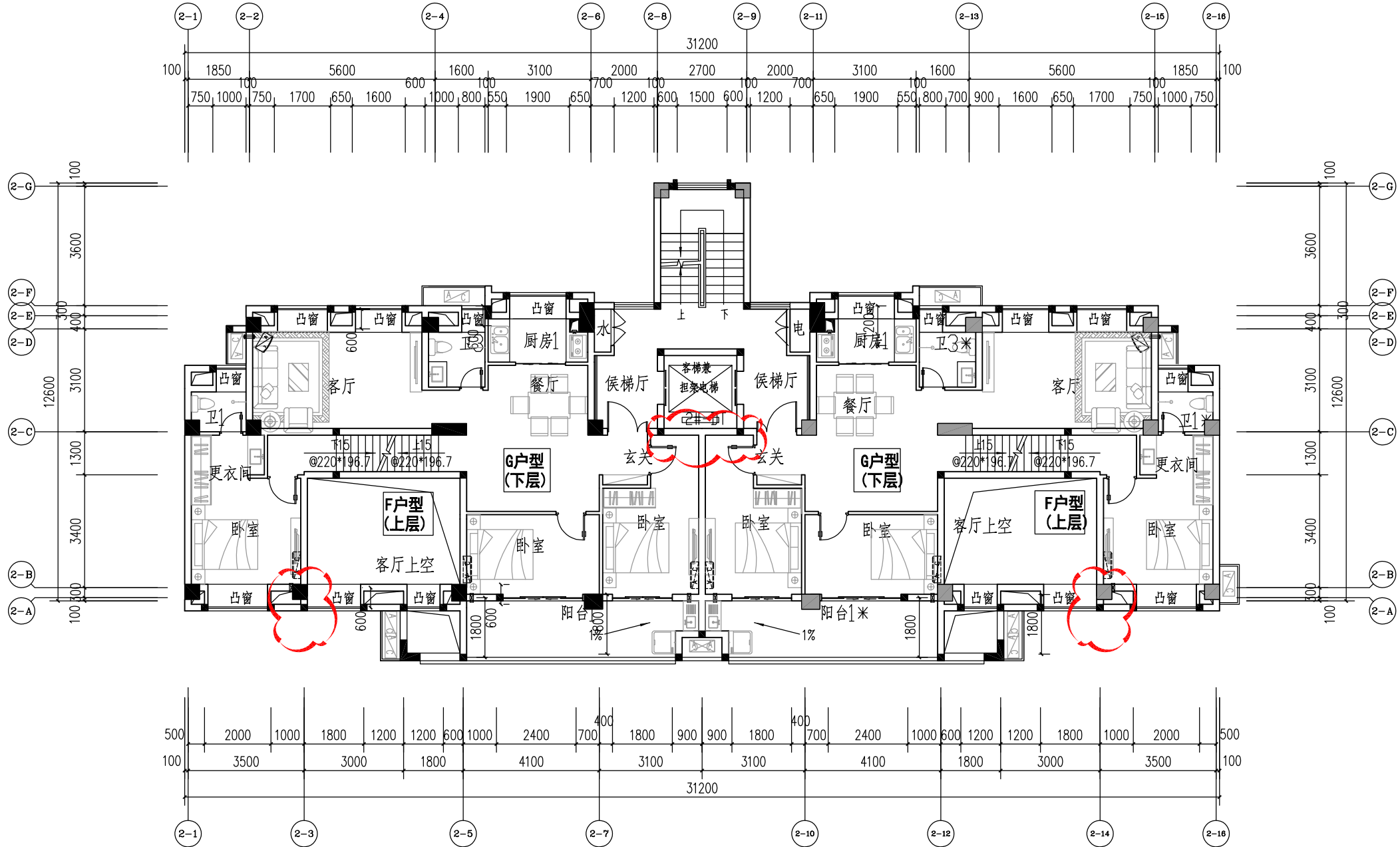
2#楼 四、六、八、十层平面图
