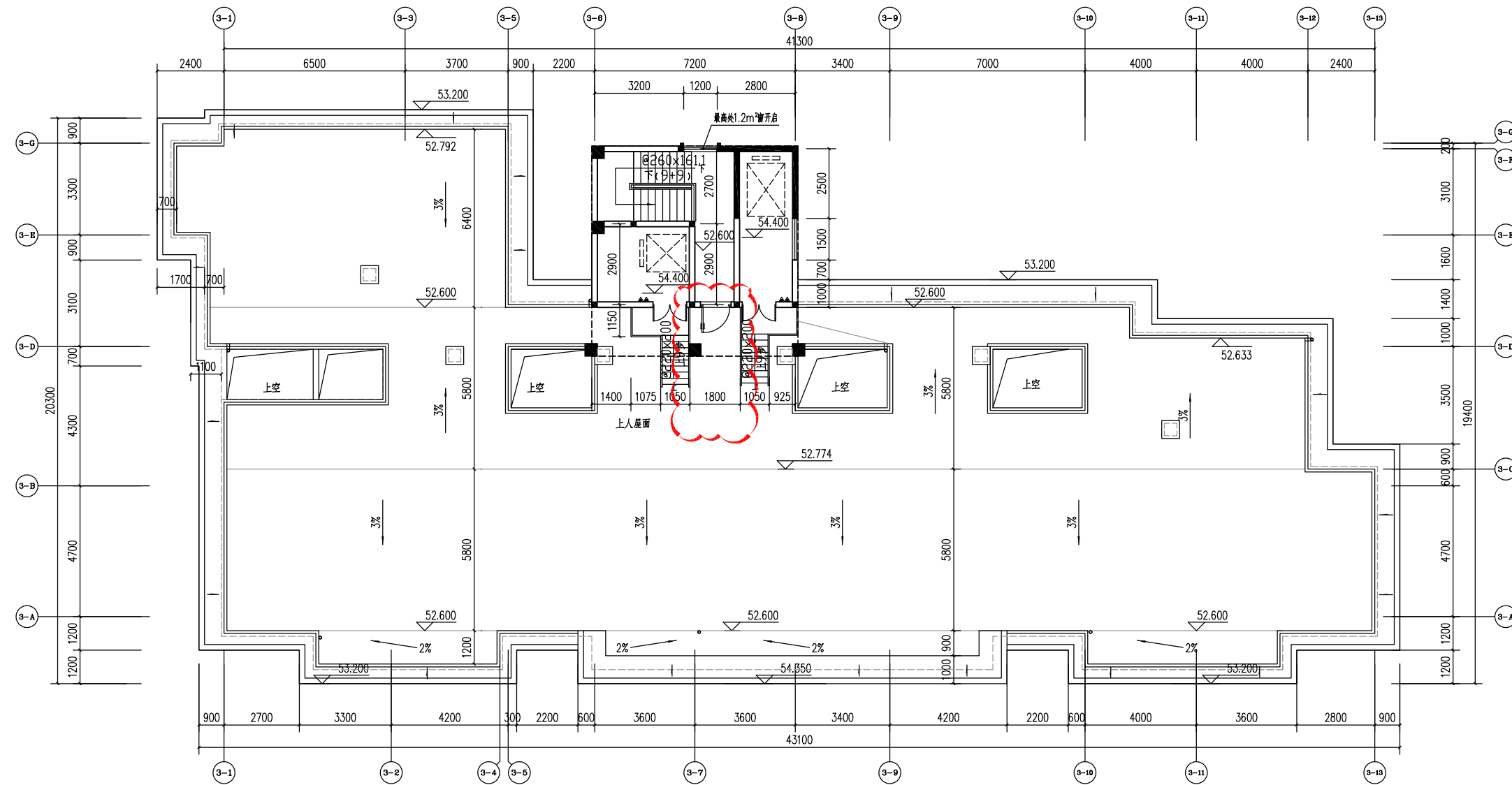
3#楼屋面平面图
