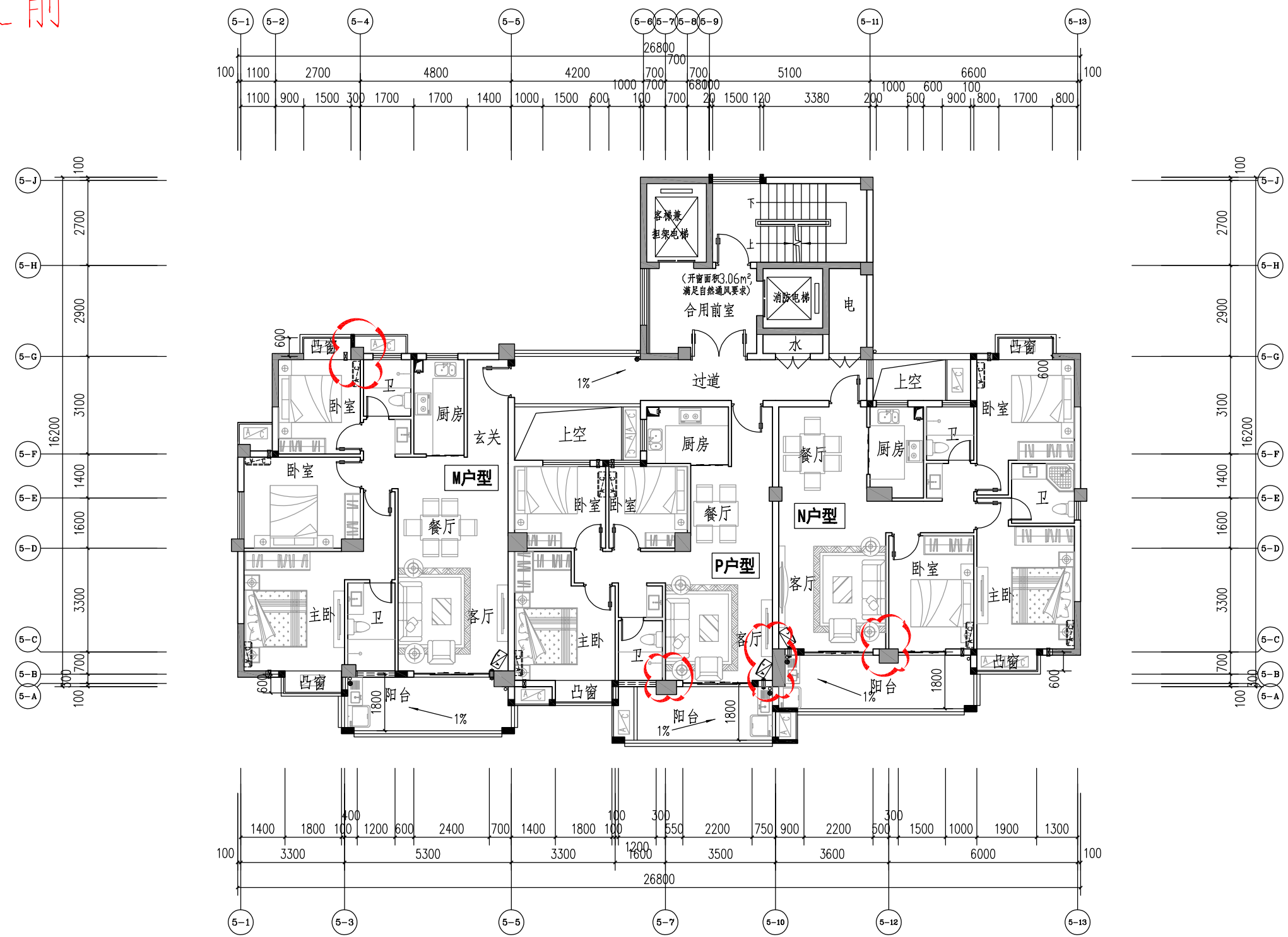
5#楼 三~十八层平面图
