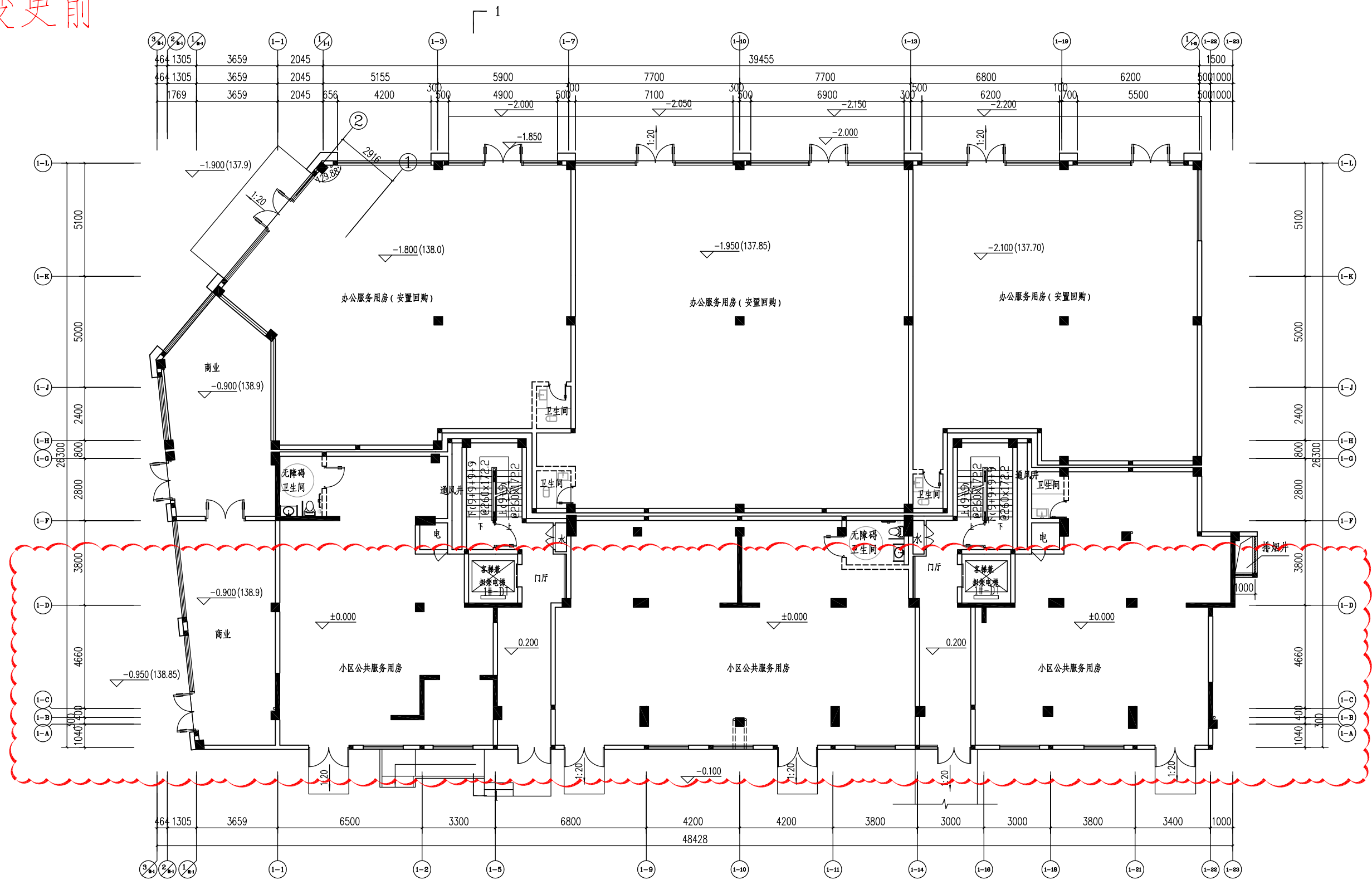
1#楼一层平面图
