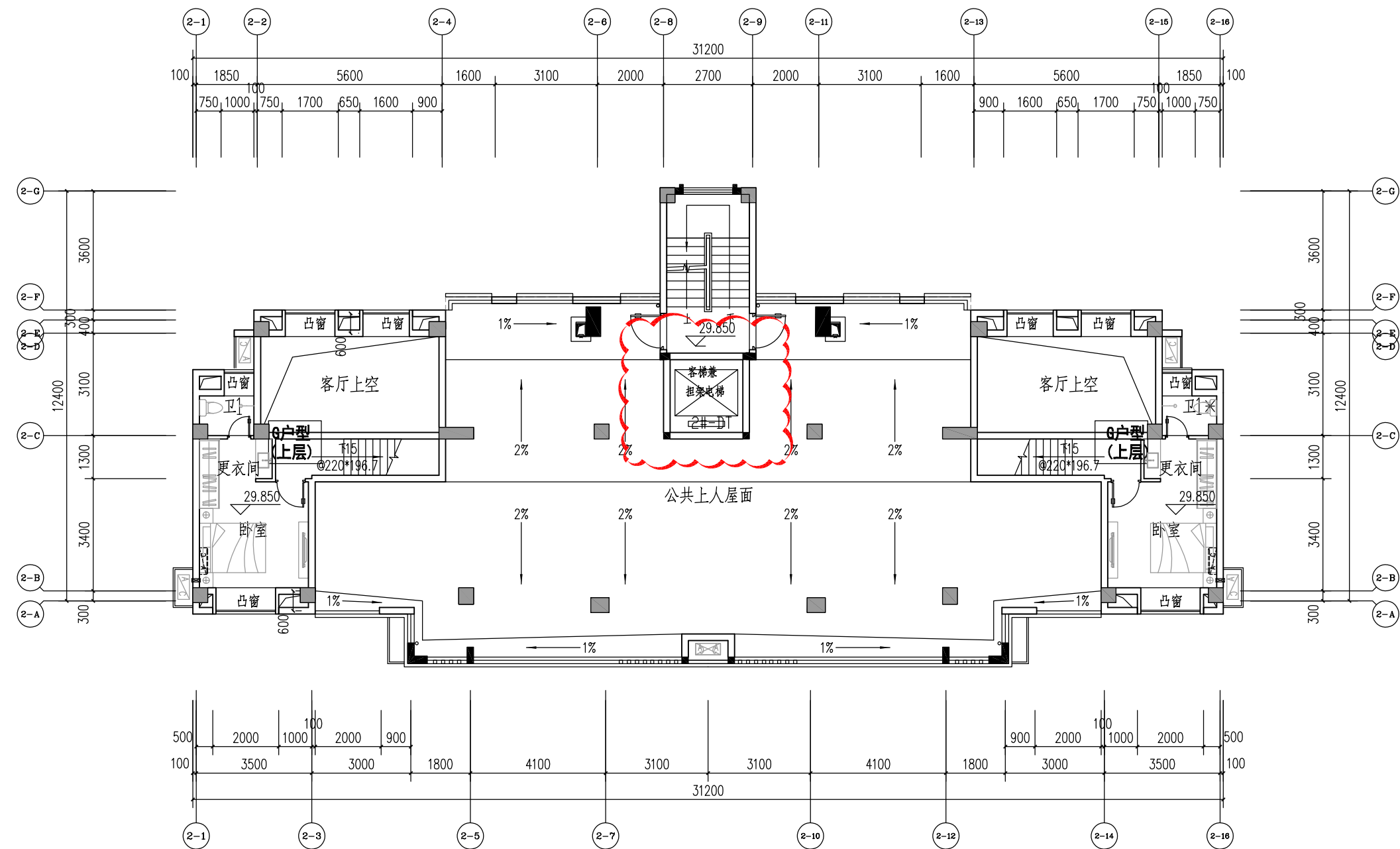
2#楼 十一层平面图
