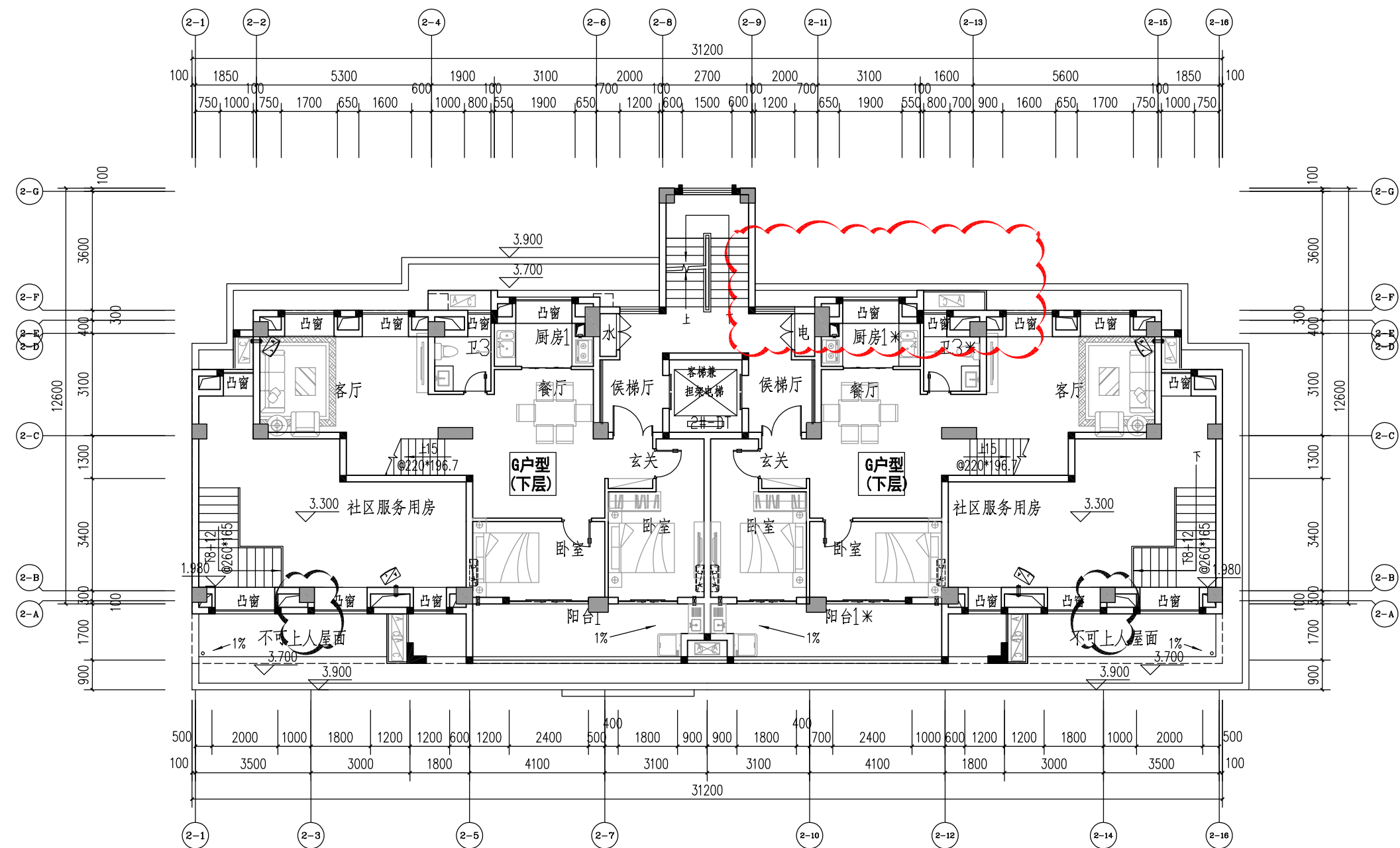
2#楼 二层平面图
