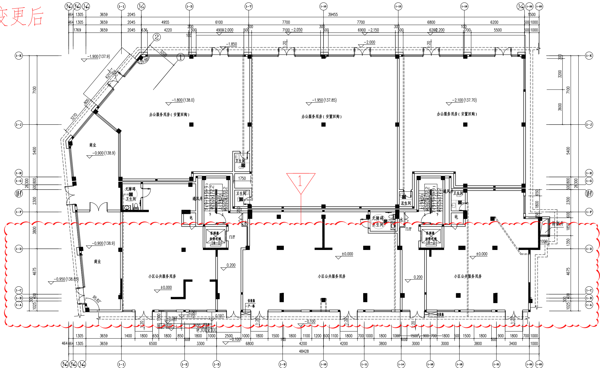
1#楼一层平面图
