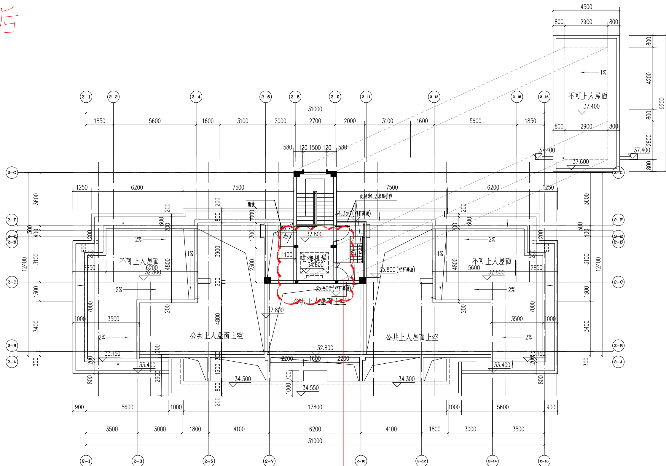
屋面层平面图
