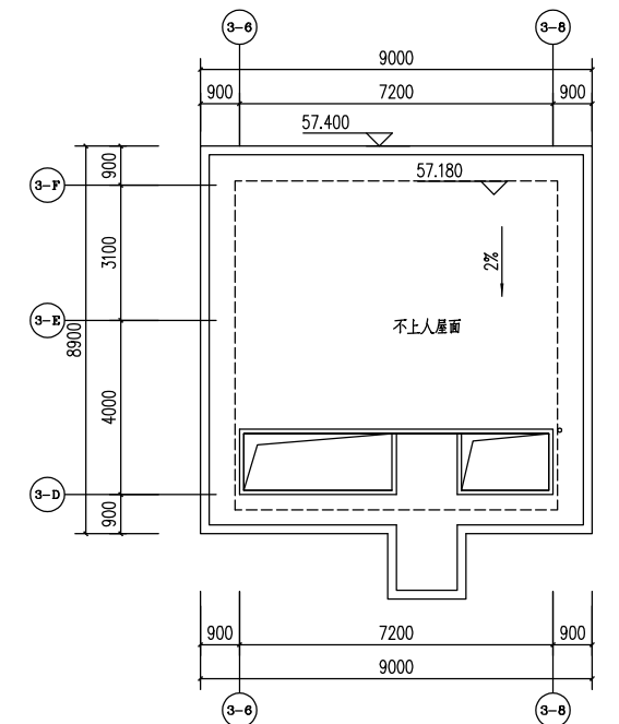
梯间屋面平面图 1:100
