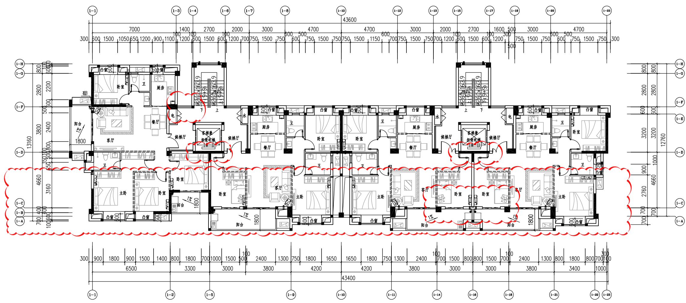
1#楼三~十层平面图
