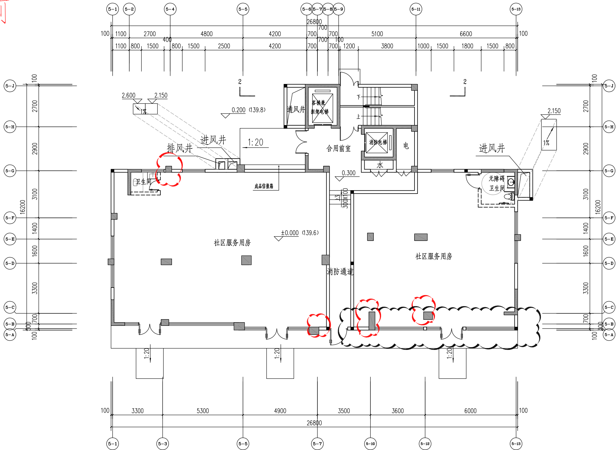
5#楼 一层平面图
