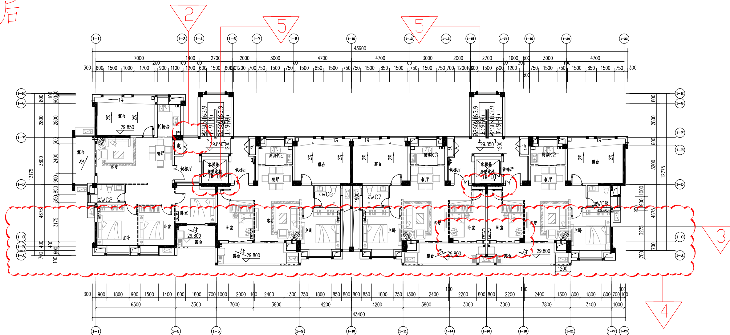
1#楼十一层平面图
