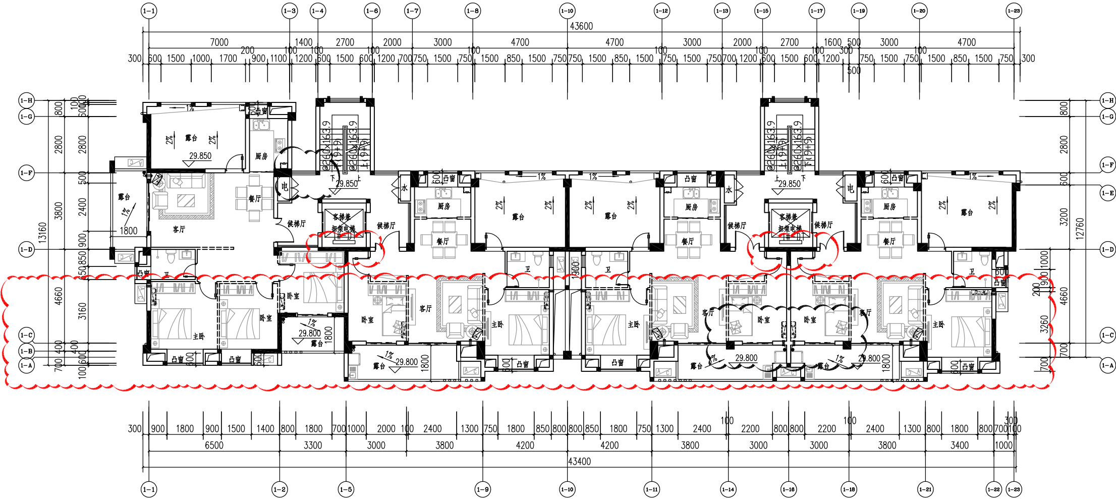
1#楼十一层平面图
