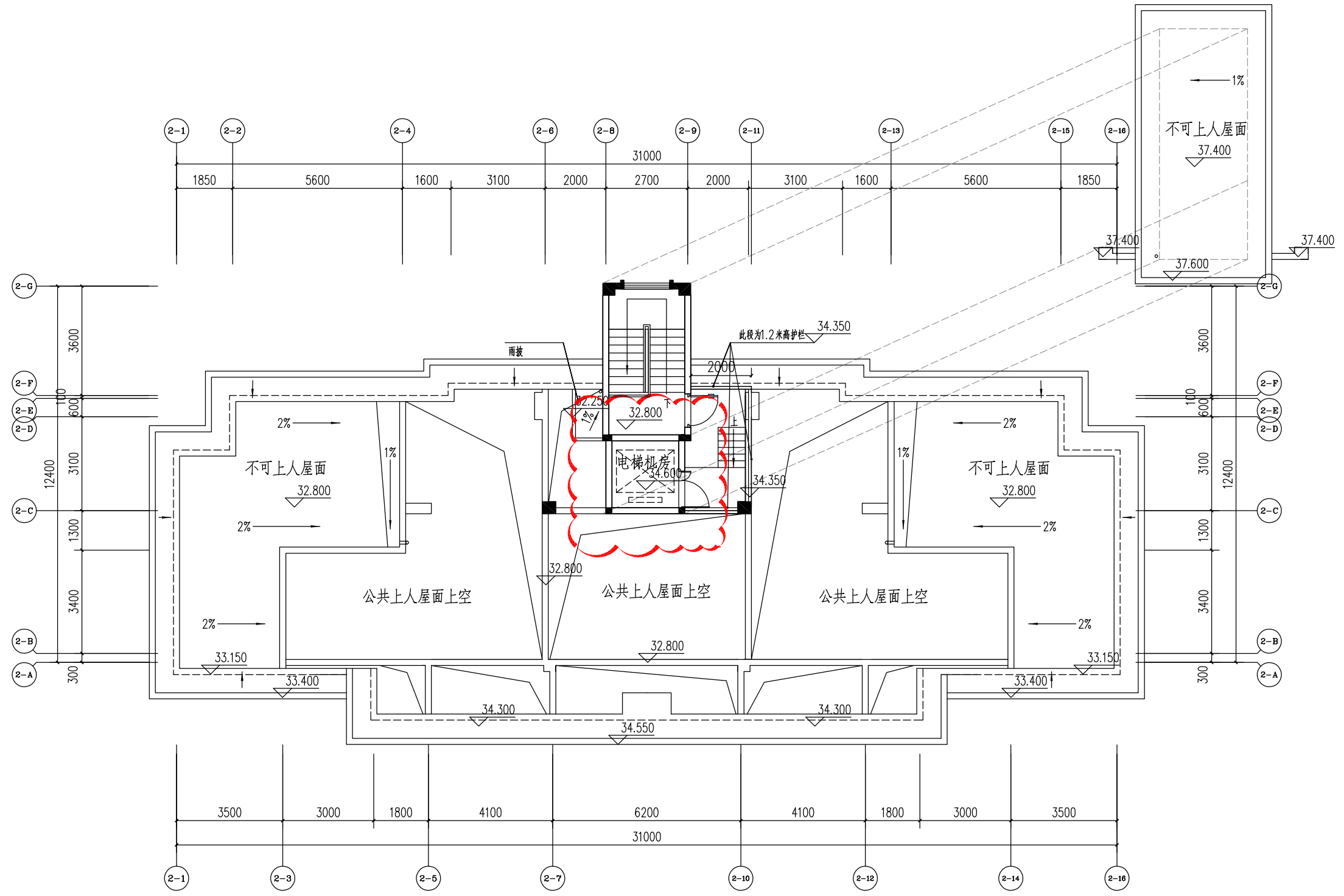
2#楼 屋面层平面图
