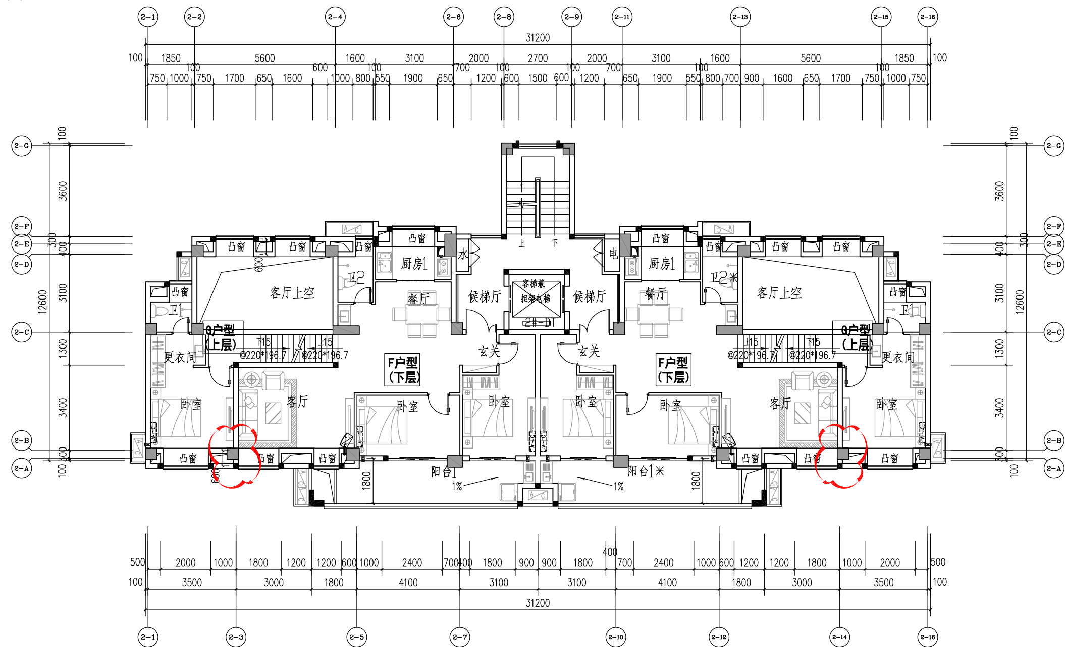
2#楼 三、五、七、九层平面图
