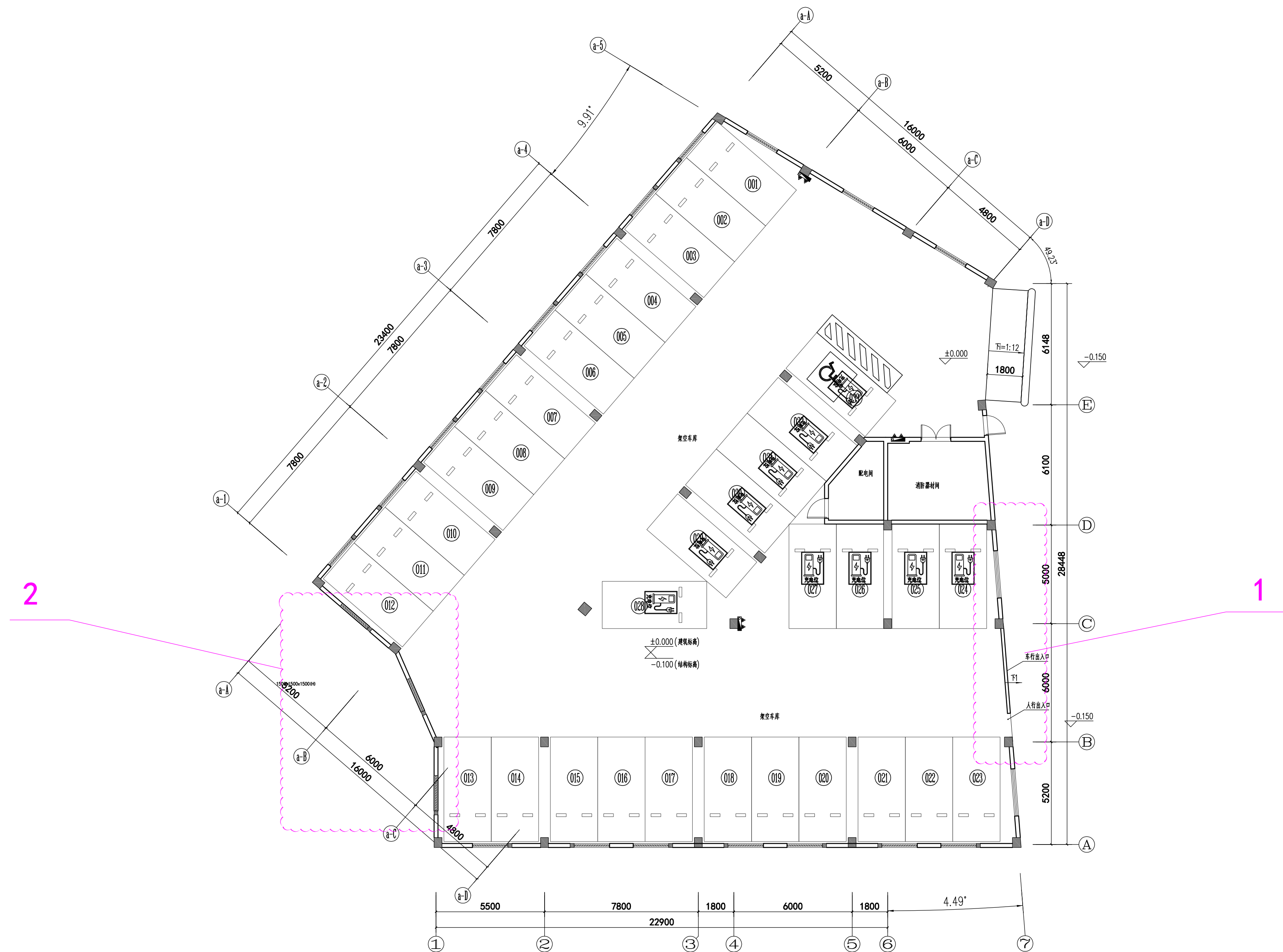
架空车库平面图 \pm 0.000 (黄海高程139.05)
