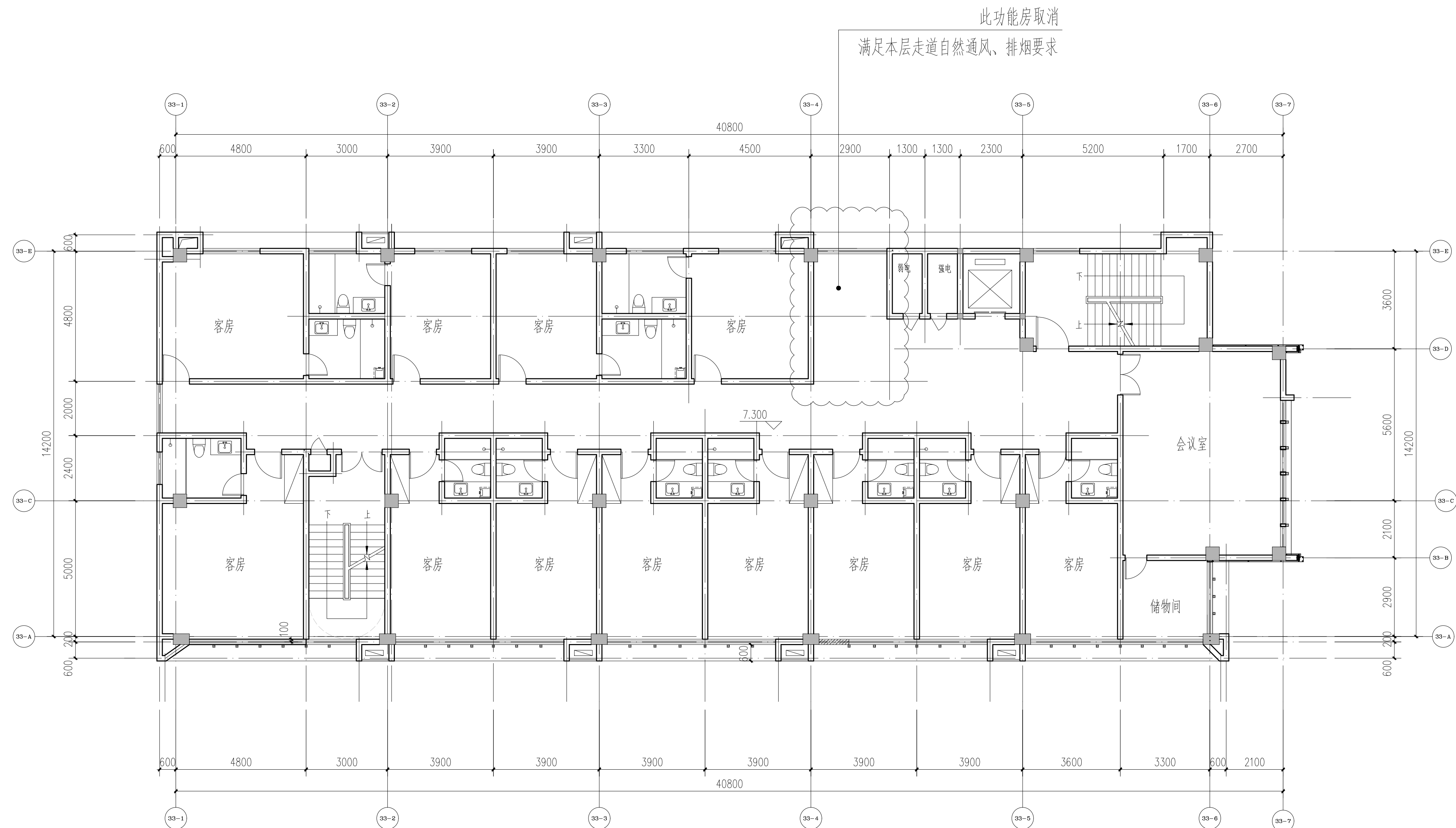
三~五层平面图 1:100
