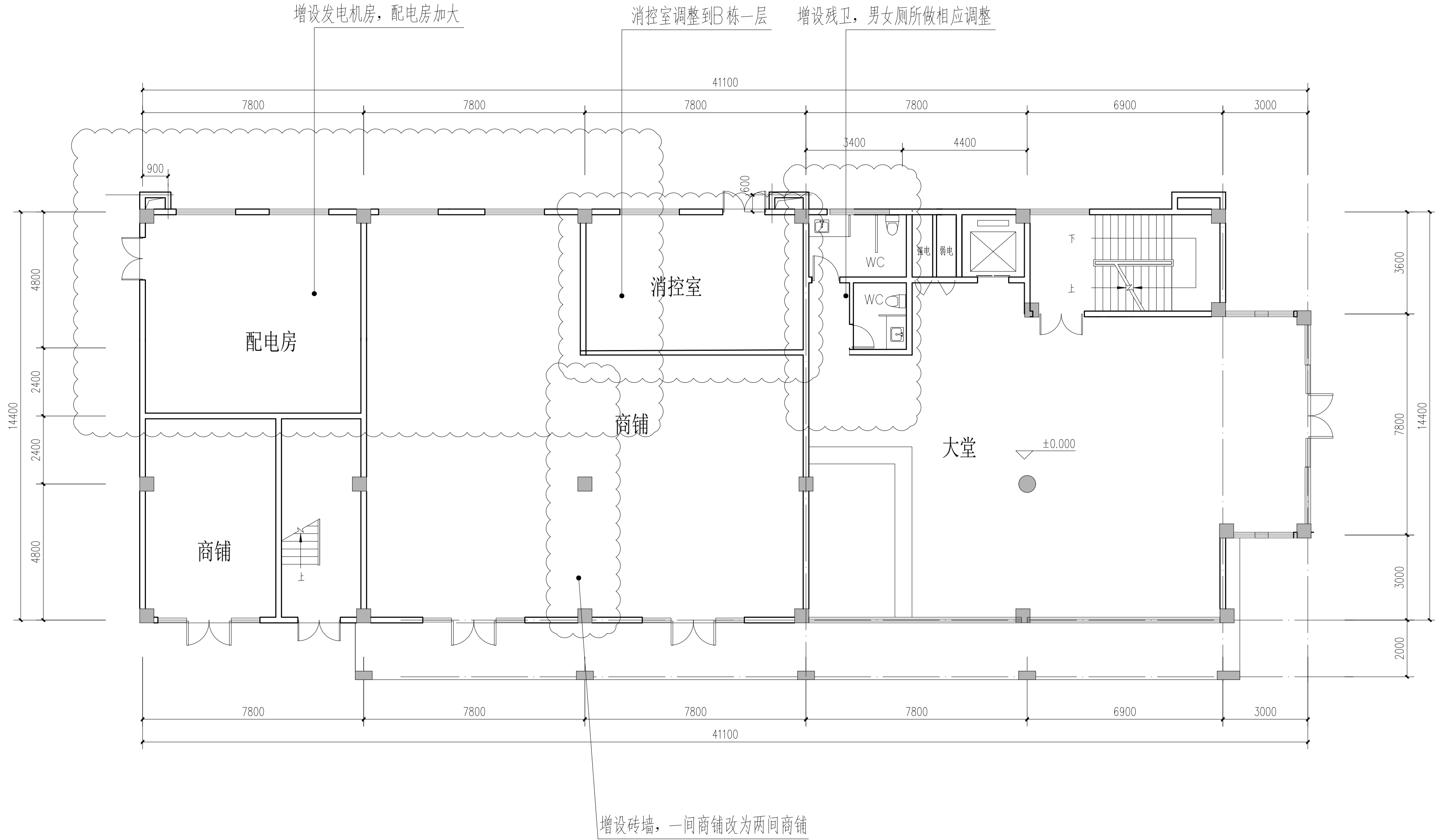
一层平面图（33井幢）
