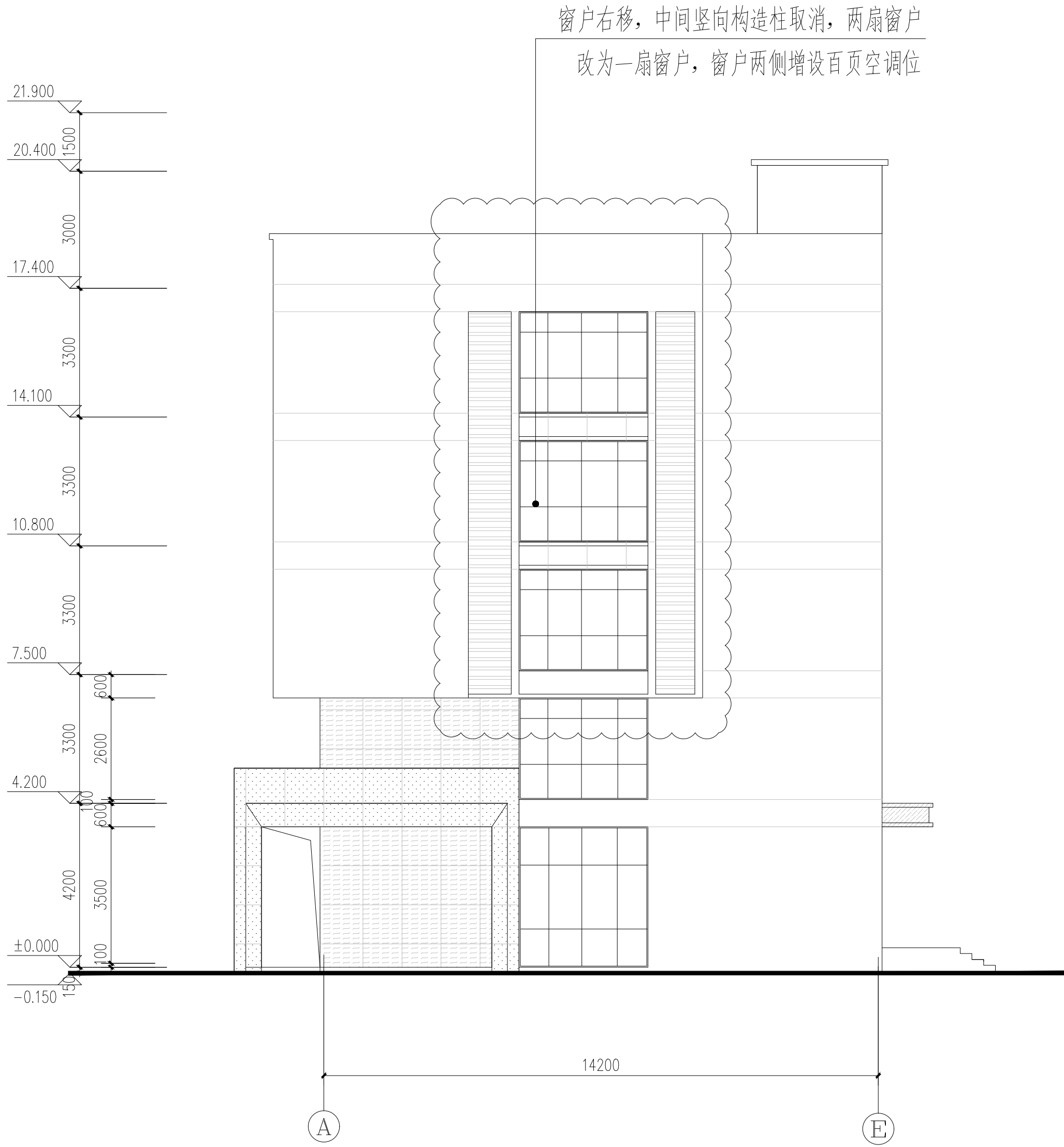
侧立面图 1:100
