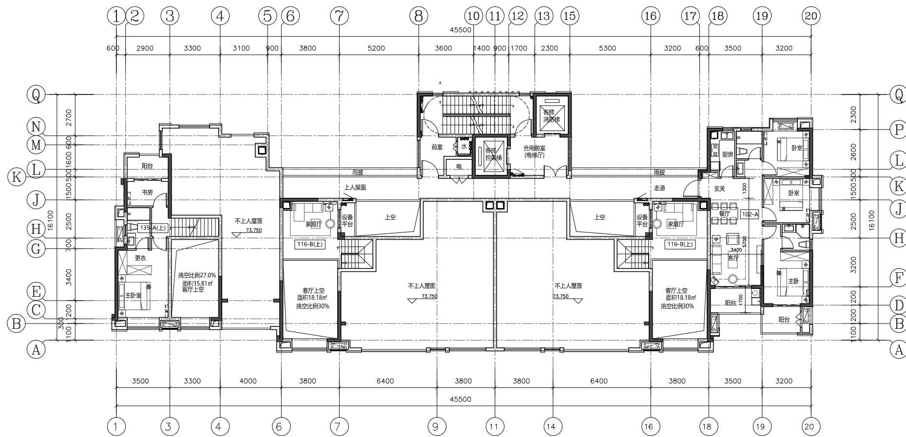
2#楼二十六层平面图（变更前）
