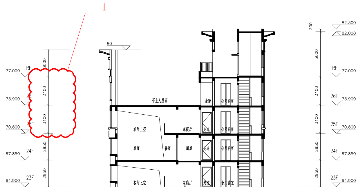
2#1-1剖面局部立面图（变更后）
