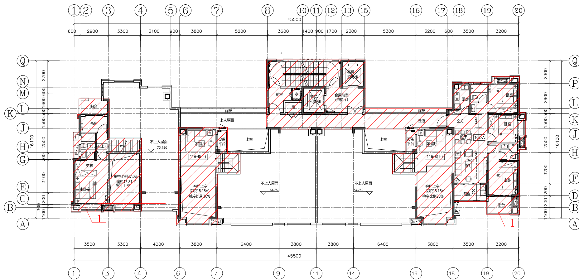
2#楼二十六层平面图（变更后）
