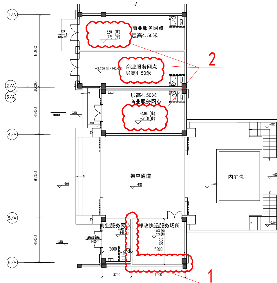
1#楼一层局部平面图（变更后）
