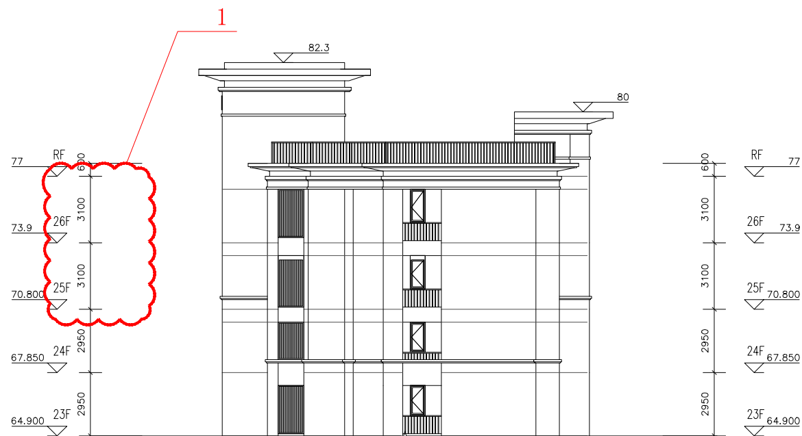
2#西立面局部立面图（变更前）
