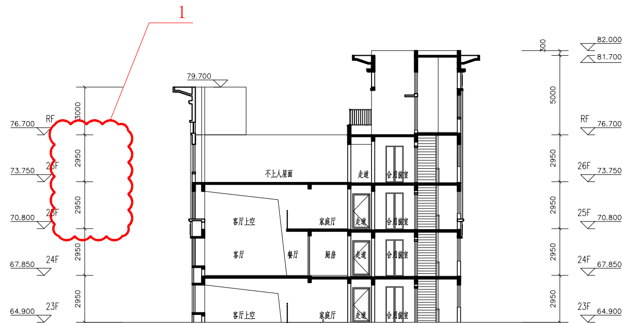
2#1-1剖面局部立面图（变更前）
