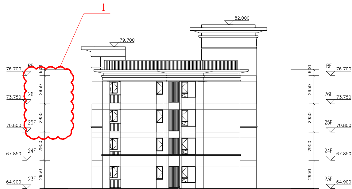
2#东立面局部立面图（变更前）
