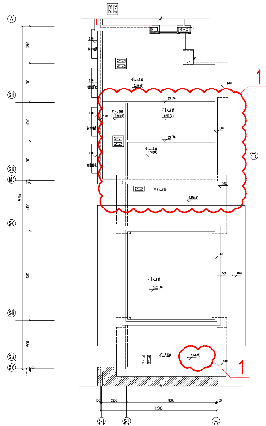
1#楼二层局部平面图（变更后）
