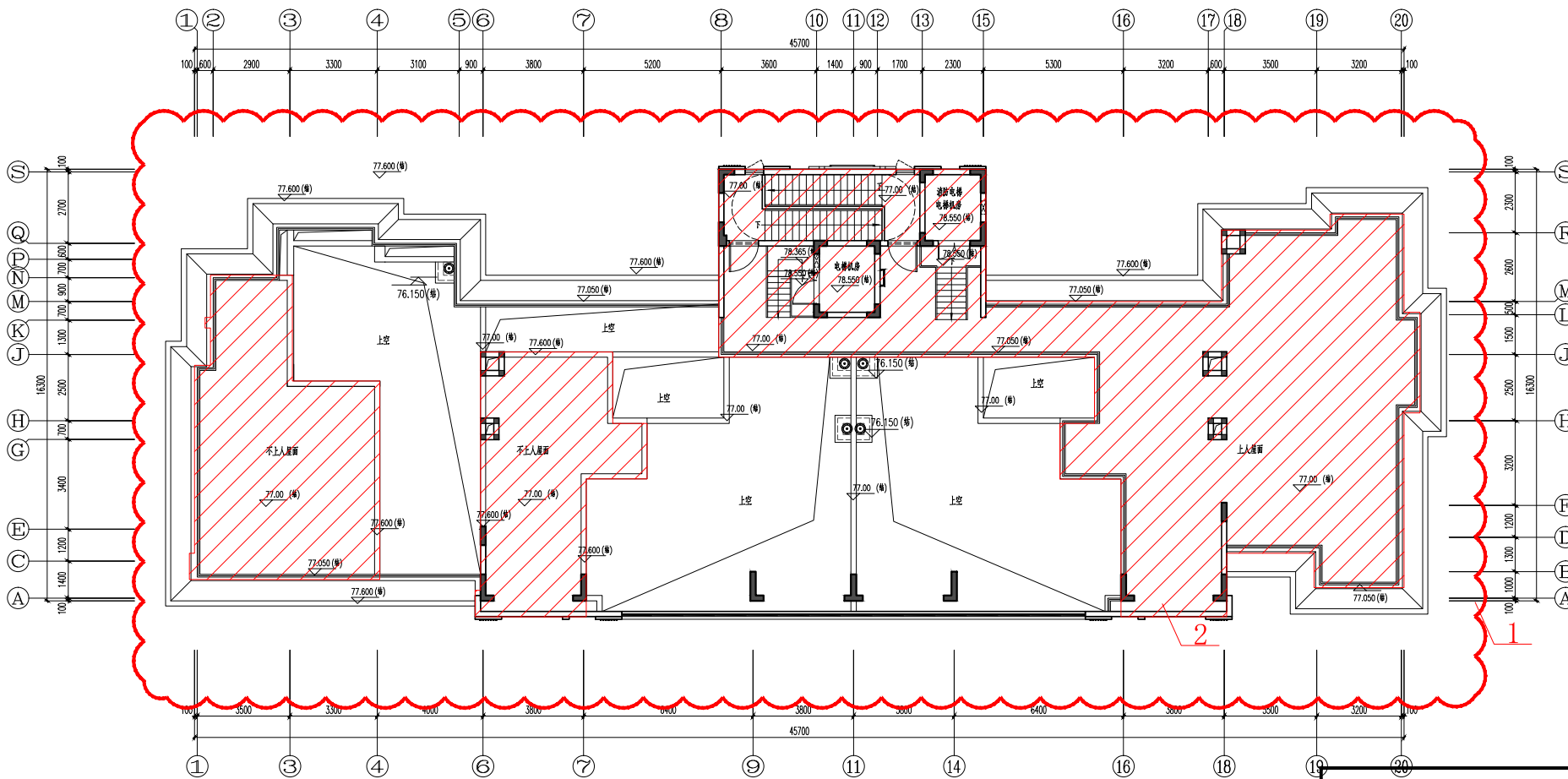
2#楼屋面层平面图（变更后）
