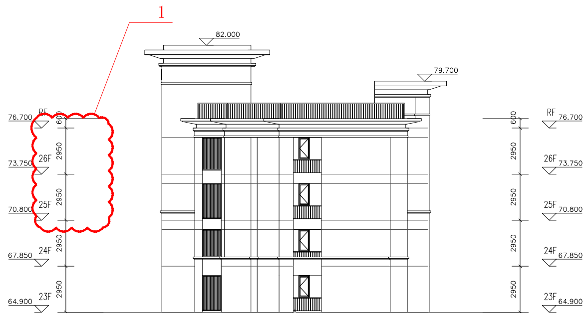
2#西立面局部立面图（变更前）
