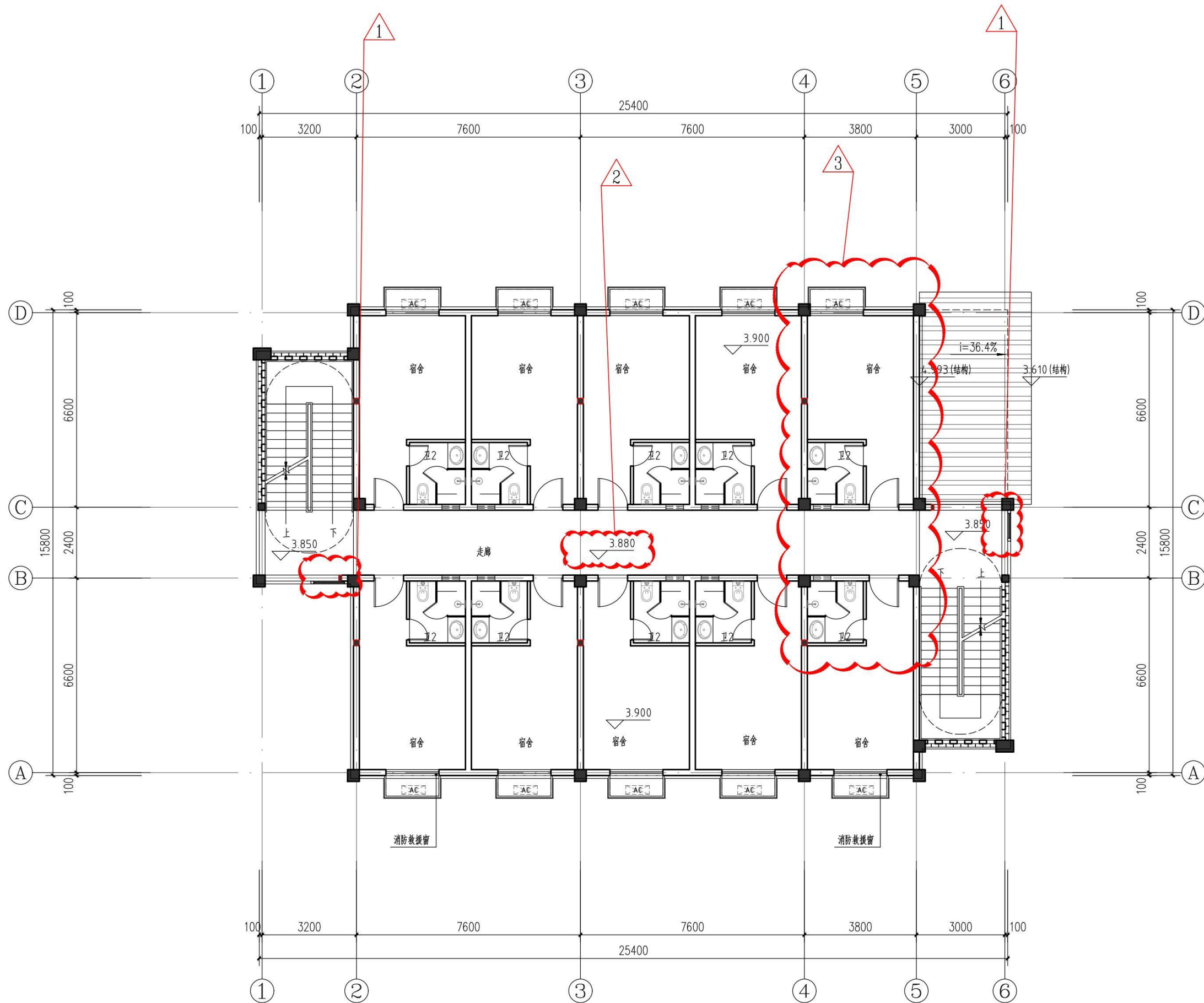
二层平面图变更前 1:100 本层建筑面积353.32平方米
