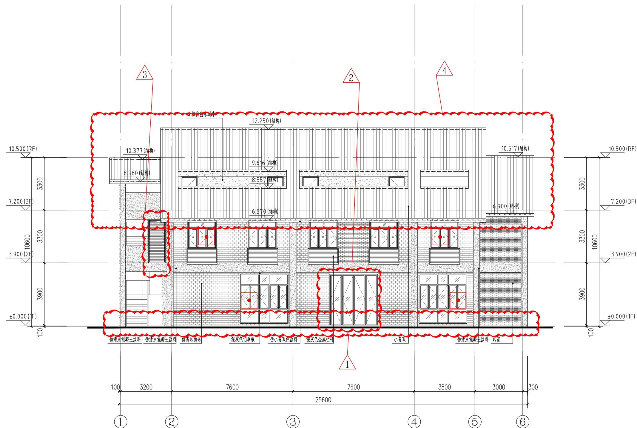
①-⑥轴立面图变更前 1:100
