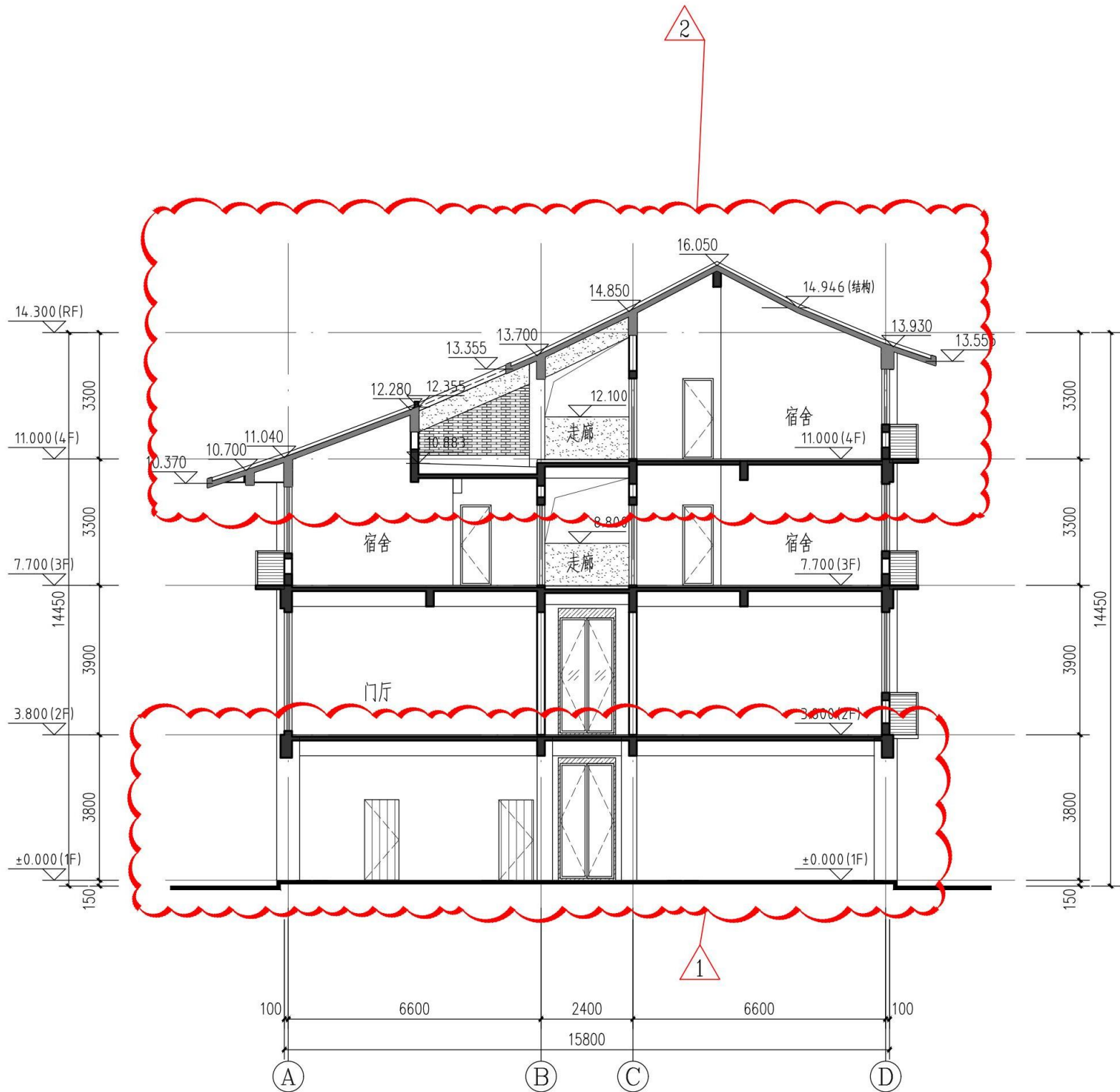
1-1剖面图变更后 1:100
