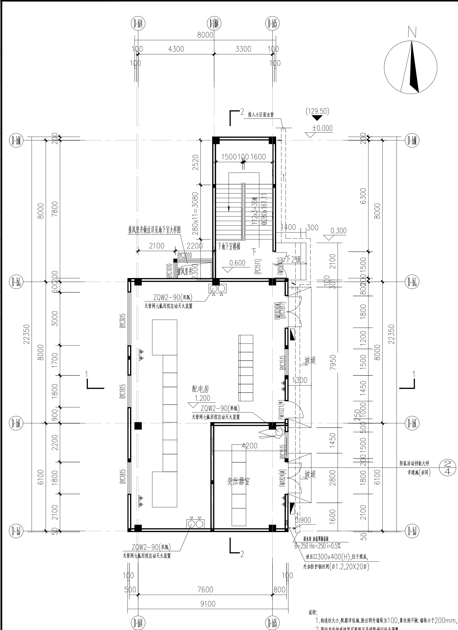
一层平面图 1:100
