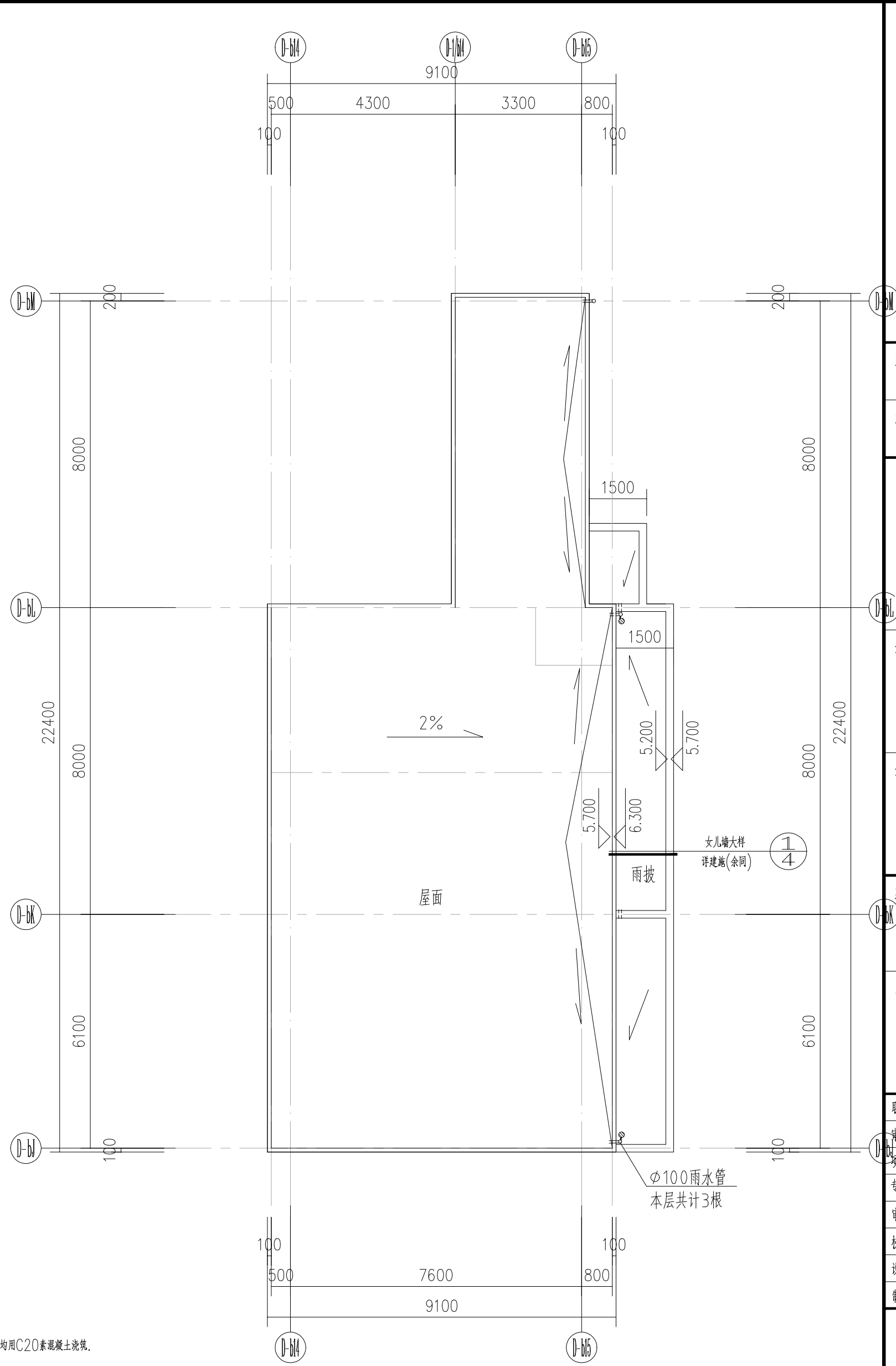
屋顶平面图 1:100
