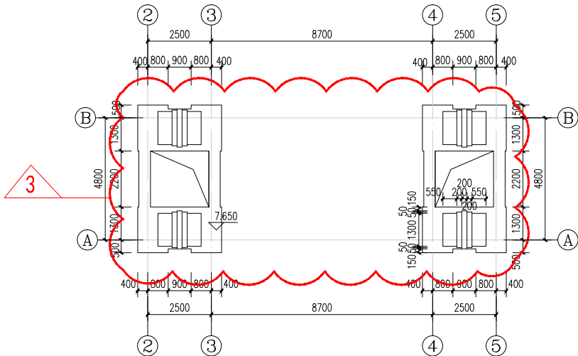
造型屋顶平面图 1:100
