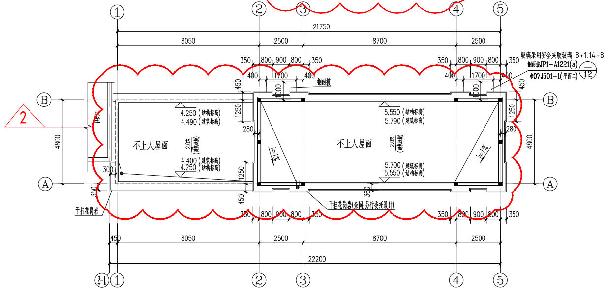
屋面平面图 1:100
