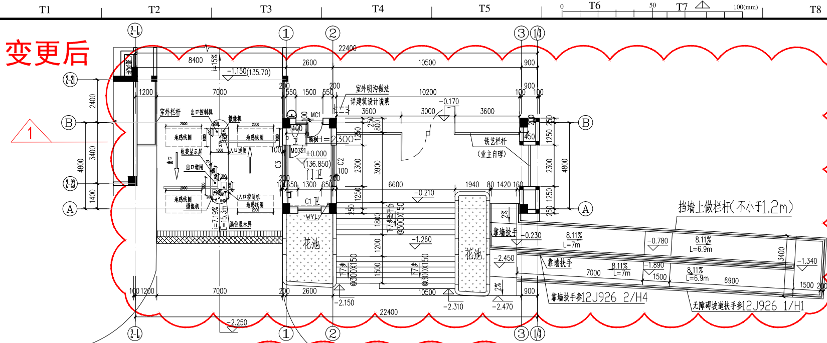
一层平面图 1:100
