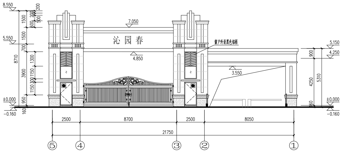
⑤~①轴立面图 1:100
