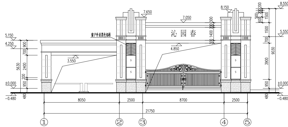
①~⑤轴立面图 1:100
