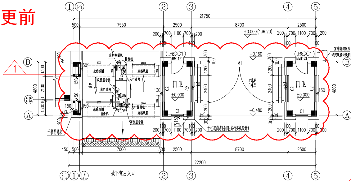
一层平面图 1:100
