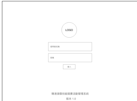
登入页面
