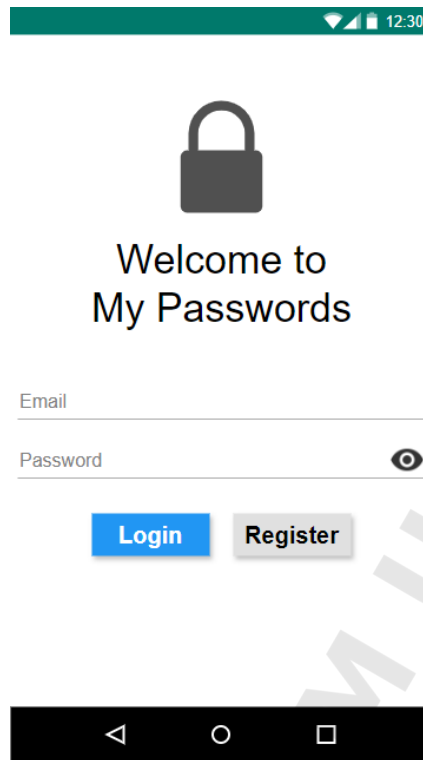
Login Page
