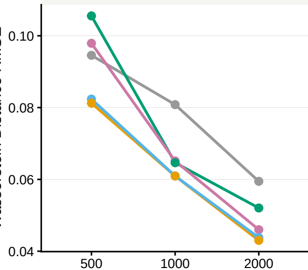
Normal Linear
