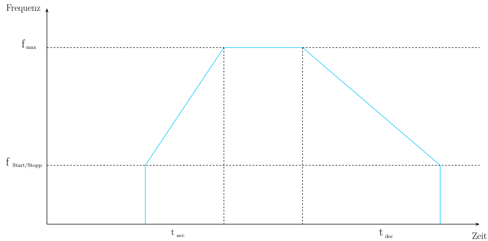
Figure 8.3.: Trapezförmiges Geschwindigkeitsprofil [FaulhaberDriveSystems.2020]
