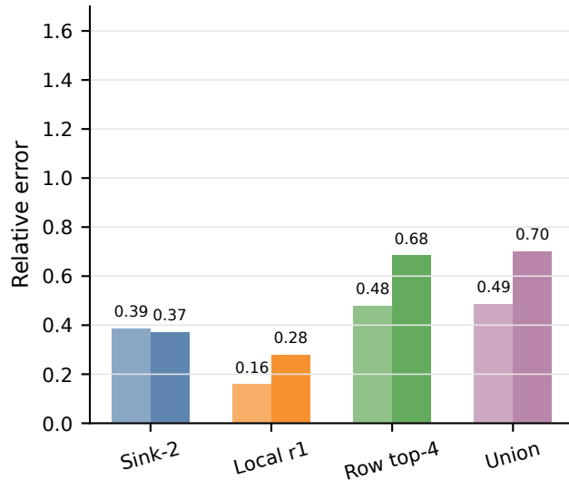
Drop + renorm A@V error
