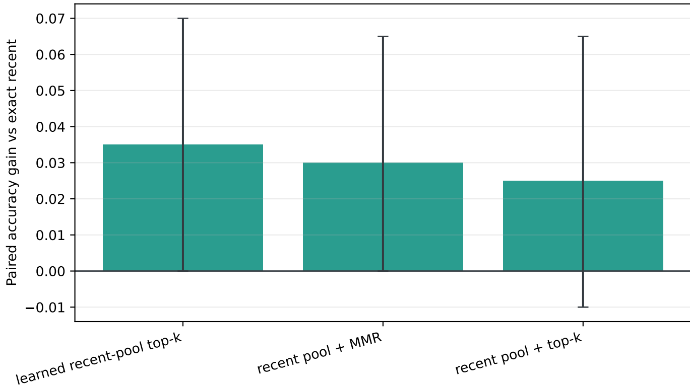
LLaVA frame-policy paired comparison
