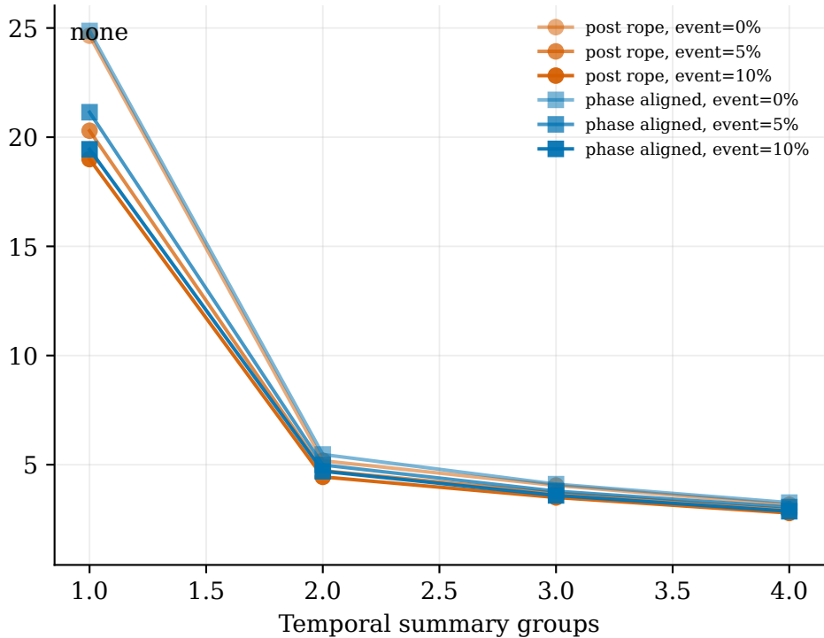
Held Out aggregate AV error (%)
