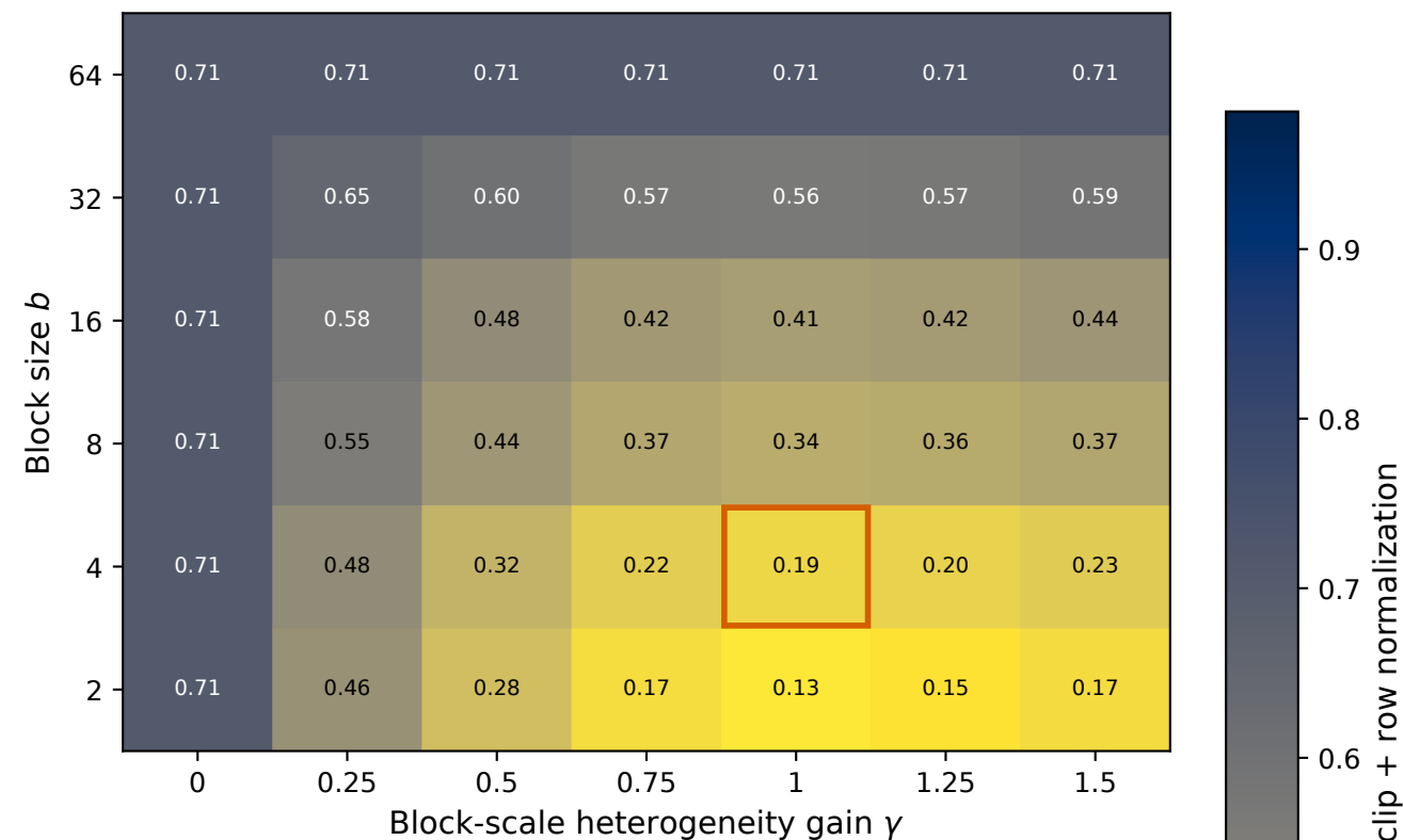
(d) Qwen L26 H0 F0
