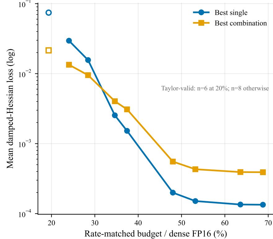
(d) \leq 1\% rate match, both endpoints Taylor-valid
